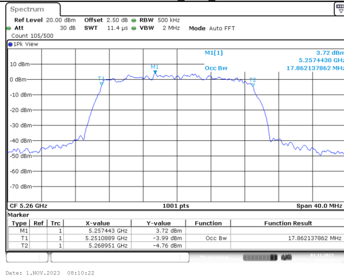
11N20MIMO_Ant4_5260
