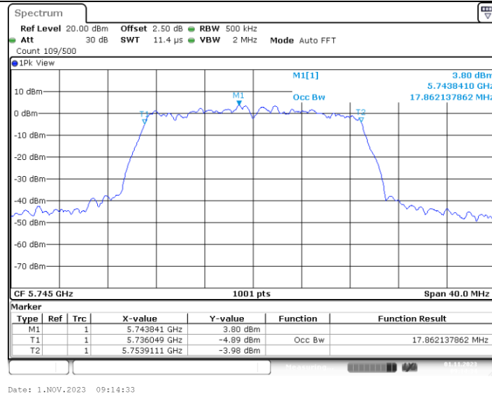
11N20MIMO_Ant3_5745
