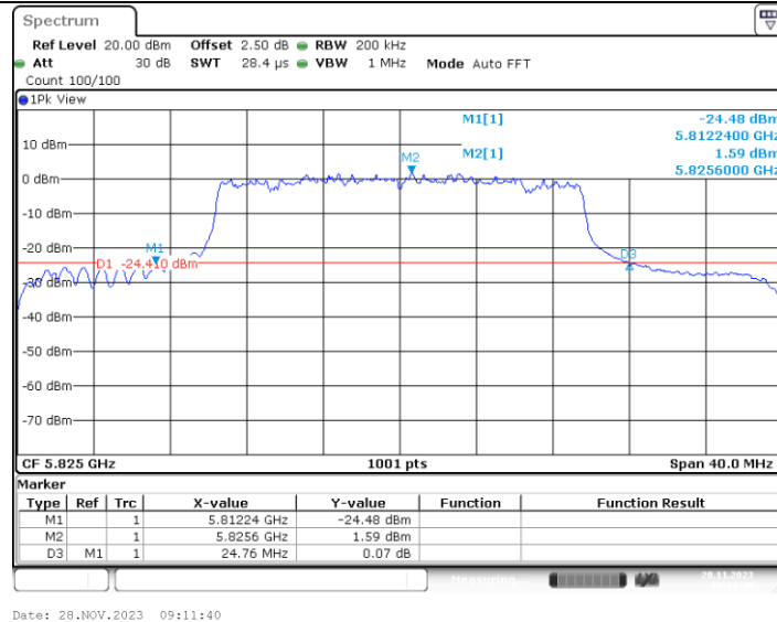
11AX20MIMO Ant2 5825 242Tone_RU61
