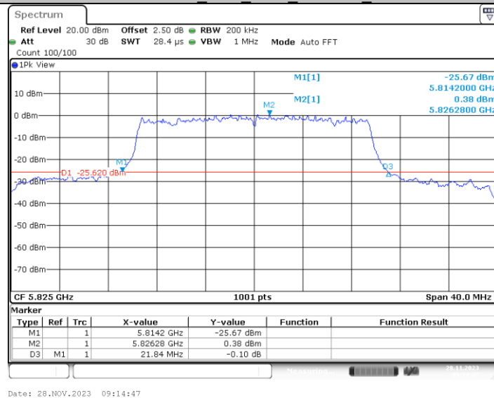
11AX20MIMO Ant3 5825 242Tone_RU61
