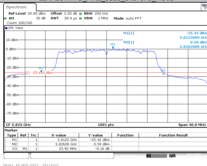
11AX20MIMO Ant4 5825 242Tone_RU61
