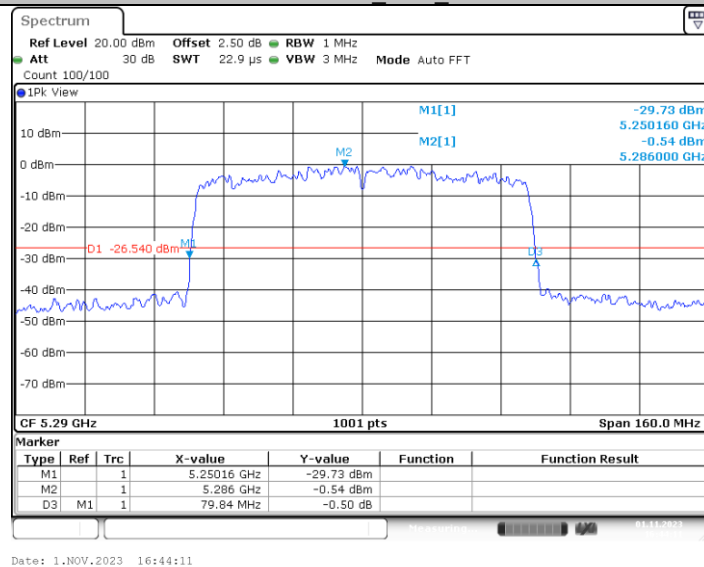
11AC80MIMO_Ant4_5290
