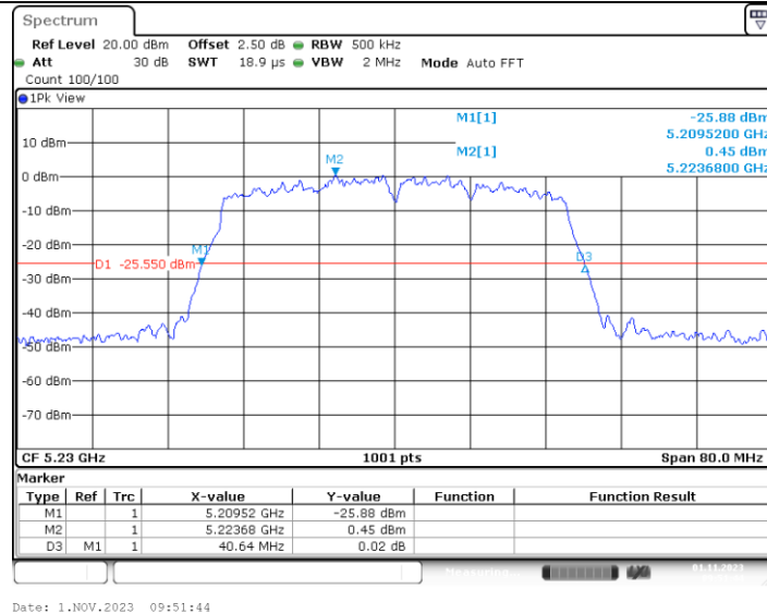
11N40MIMO_Ant3_5230
