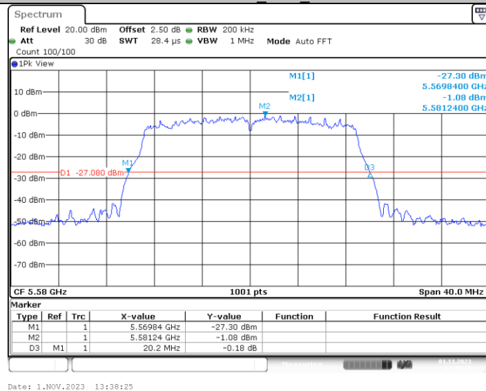
11AC20MIMO_Ant4_5580
