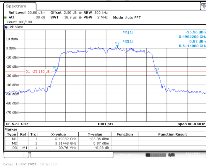
11N40MIMO_Ant4_5510
