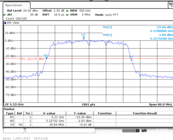
11N40MIMO_Ant4_5230
