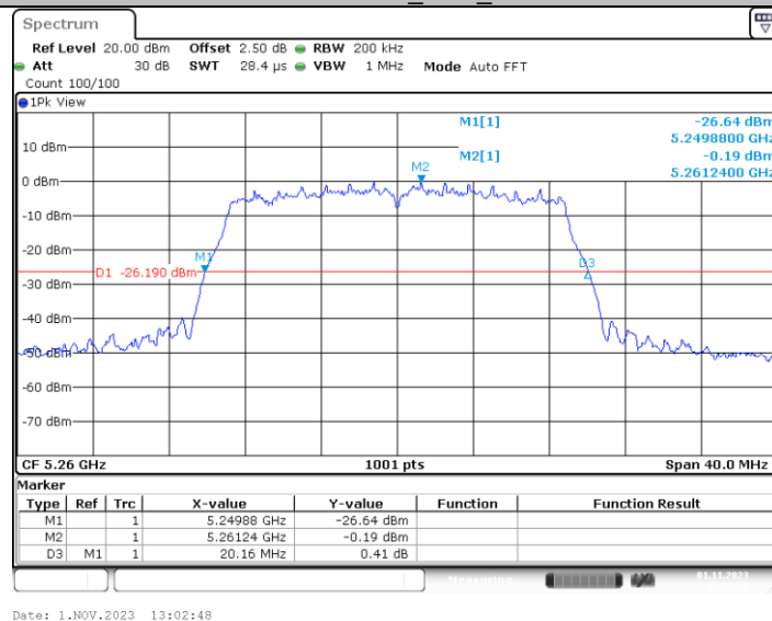
11AC20MIMO_Ant3_5260
