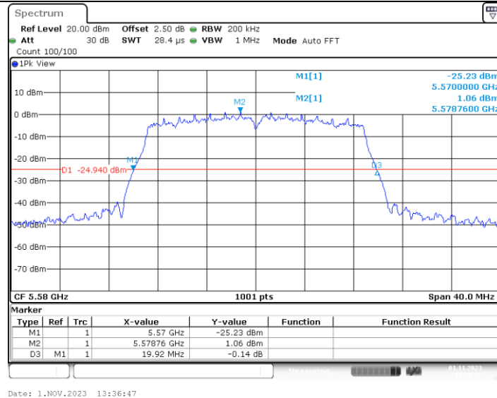
11AC20MIMO_Ant3_5580
