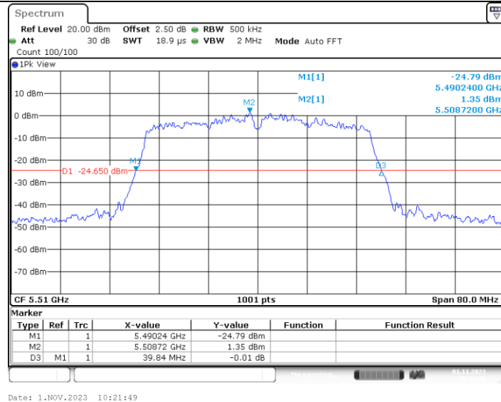
11N40MIMO_Ant3_5510
