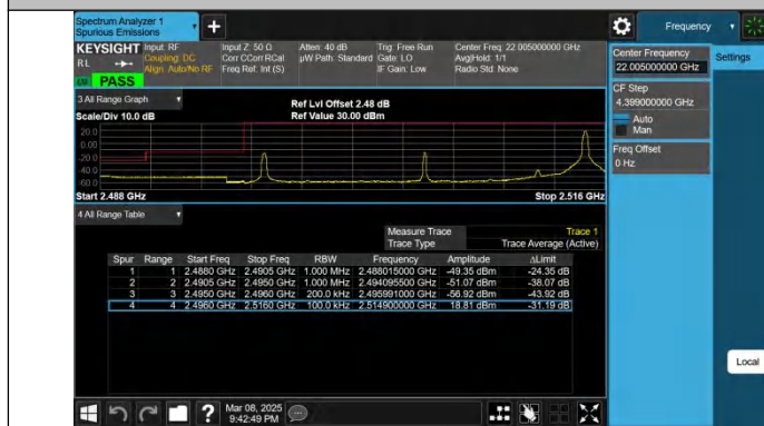
Band41-20MHz-QPSK-39750-1RB#99-PASS
