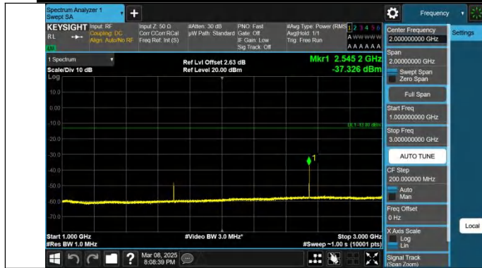
Band26(824-849)-10MHz-QPSK-26990-1RB#49-1000~3000-PAS
