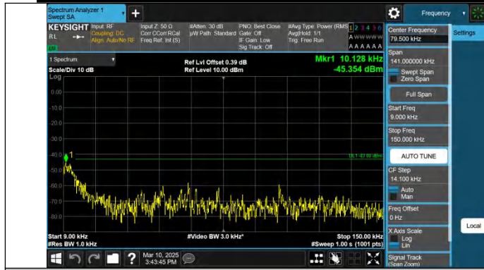
Band25-20MHz-QPSK-26365-1RB#0-0.009~0.15-PASS
