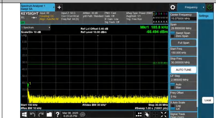
Band25-10MHz-QPSK-26365-1RB#0-0.15~30-PASS
