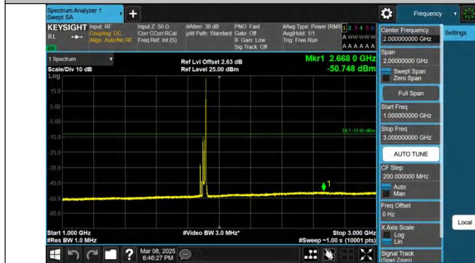
Band25-20MHz-QPSK-26590-1RB#99-1000~3000-PASS
