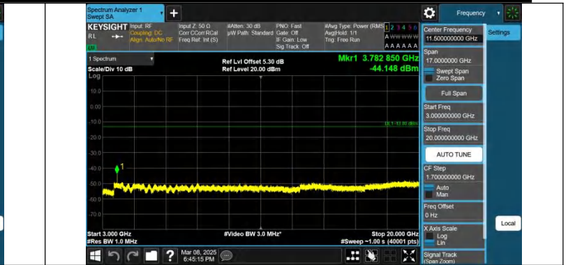
Band25-20MHz-QPSK-26365-1RB#99-3000~20000-PASS
