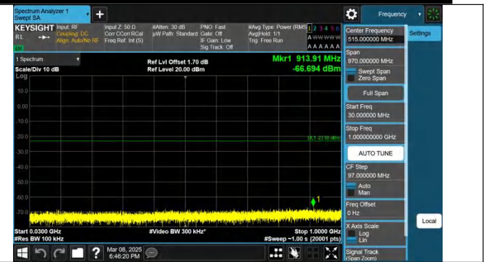
Band25-20MHz-QPSK-26590-1RB#99-30~1000-PASS
