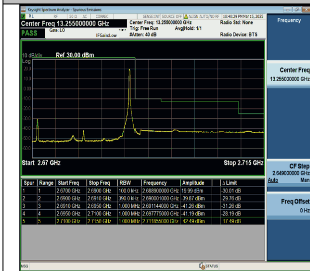
Band41-20MHz-QPSK-41490-1RB#99-PASS
