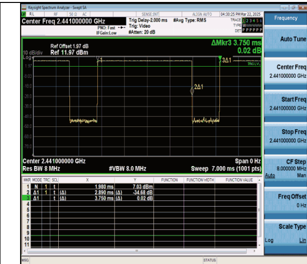
NTNV-DH5-Ant0-2441
