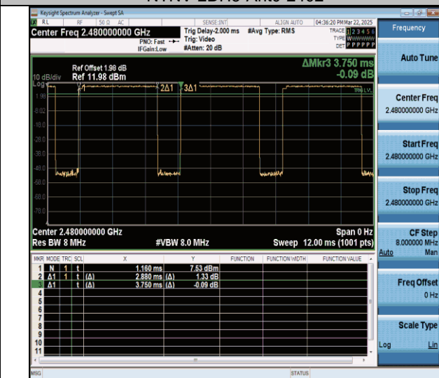
NTNV-2DH5-Ant0-2480
