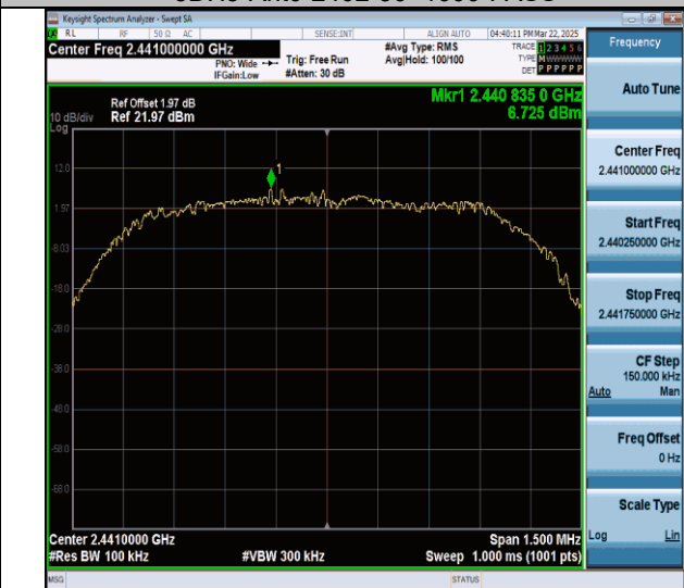
3DH5-Ant0-2441-0~Reference-PASS
