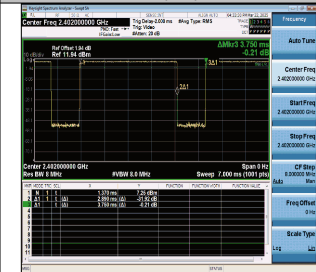
NTNV-2DH5-Ant0-2402
