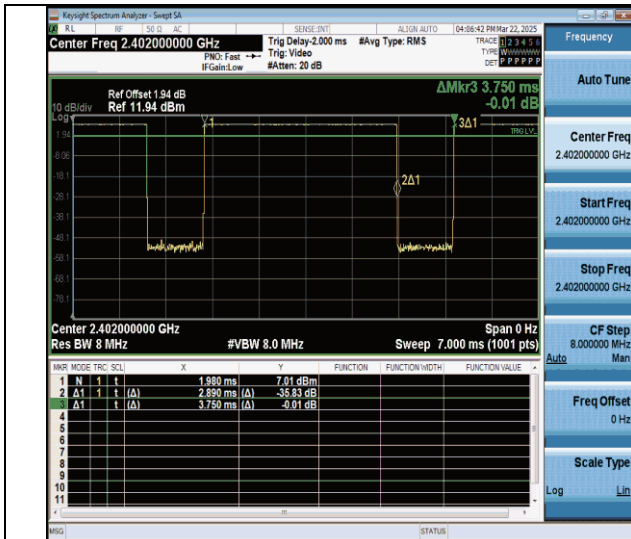
NTNV-DH5-Ant0-2402
