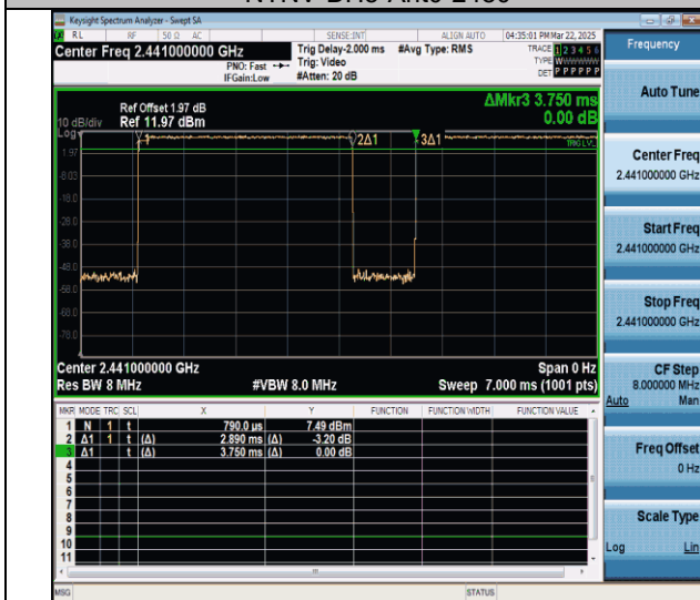
NTNV-2DH5-Ant0-2441
