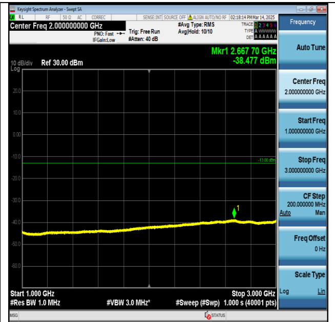
Band71-20MHz-QPSK-133372-1RB#0-1000~3000-PASS
