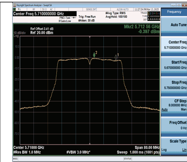
11ac40SISO-Ant0-5710_UNII-2C-PASS
