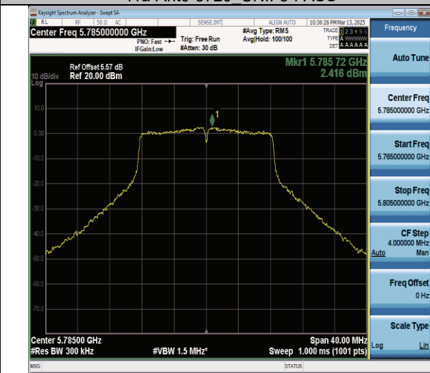
11a-Ant0-5785-PASS
