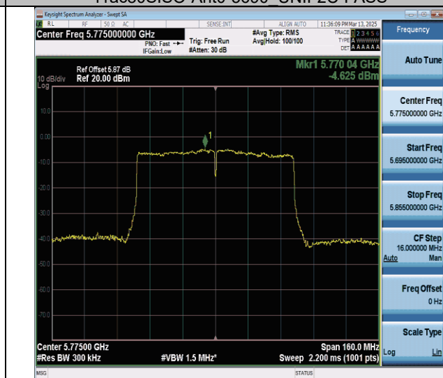
11ac80SISO-Ant0-5775-PASS
