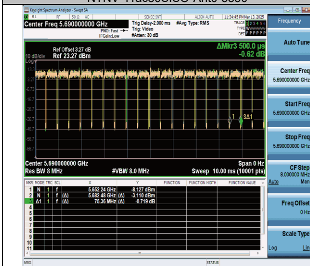
NTNV-11ac80SISO-Ant0-5690
