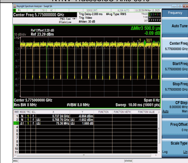
NTNV-11ac80SISO-Ant0-5775
