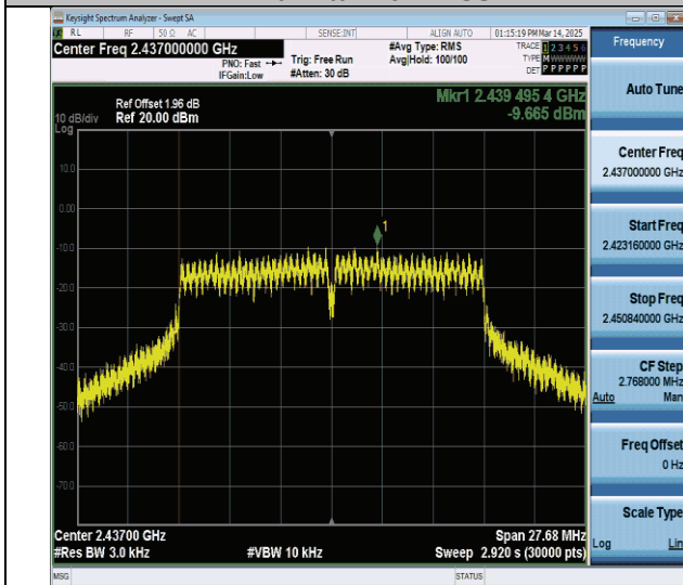
11g-Ant0-2437-PASS
