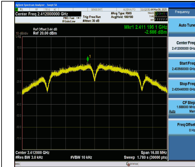
11b-Ant0-2412-PASS
