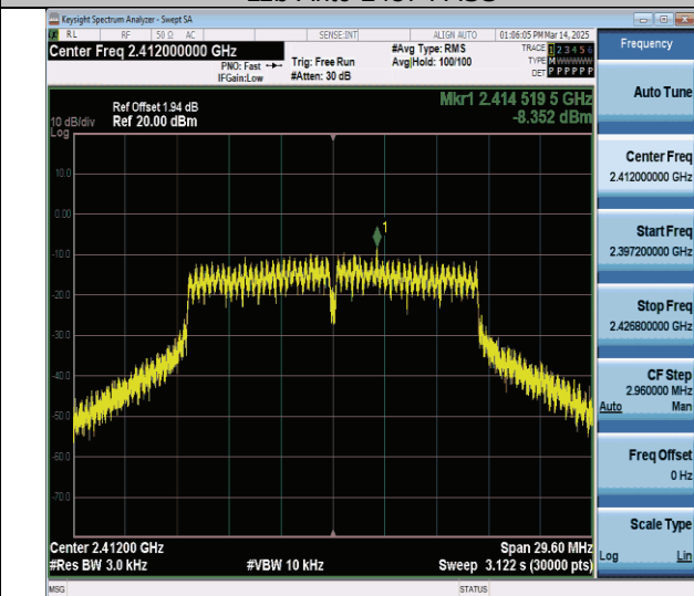
11g-Ant0-2412-PASS
