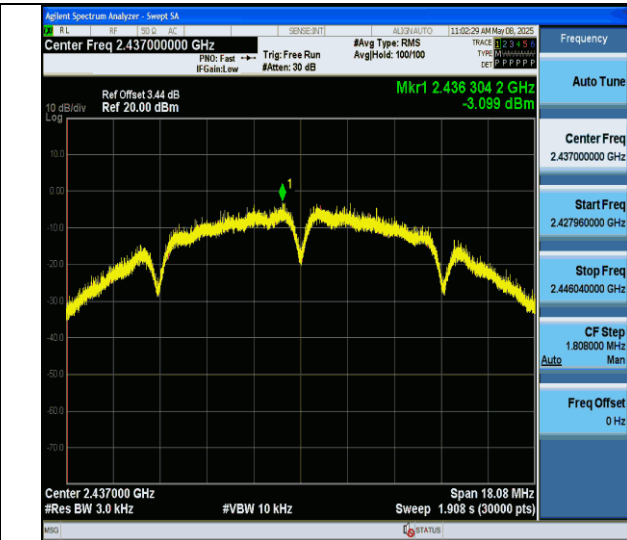
11b-Ant0-2437-PASS
