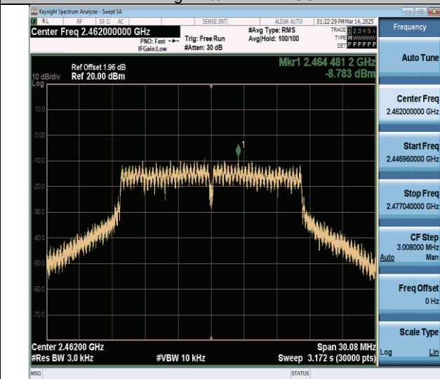
11g-Ant0-2462-PASS
