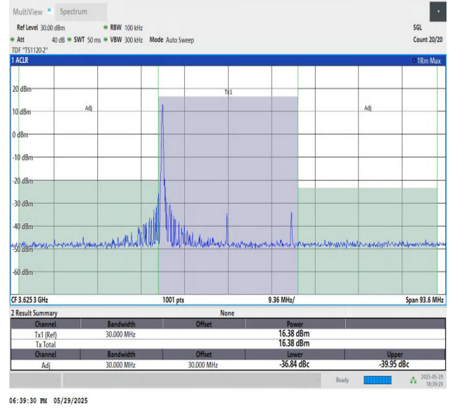
48-48-10MHz-20MHz-16QAM-16QAM-55896-56040-1RB#0-1RB#9 9-PASS
