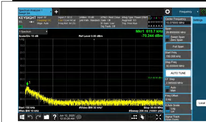
48-48-20MHz-20MHz-QPSK-QPSK-55891-56089-1RB#99-0RB# 0-0.15~30MHz-PASS
