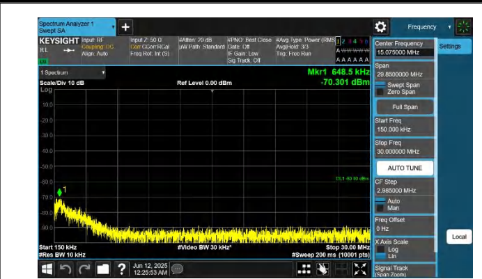
48-48-20MHz-15MHz-QPSK-QPSK-55916-56087-1RB#0-0RB#0- 0.15~30MHz-PASS
