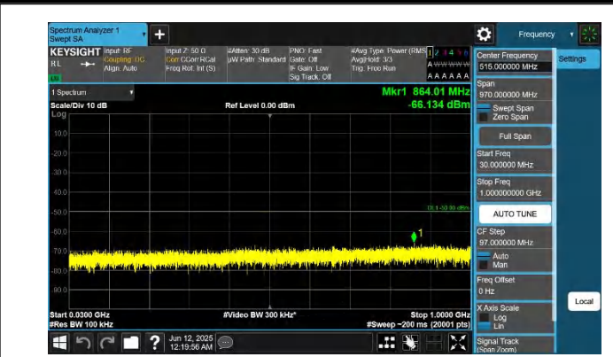
48-48-20MHz-10MHz-QPSK-QPSK-55941-56085-1RB#99-0RB# 0-30~1000MHz-PASS
