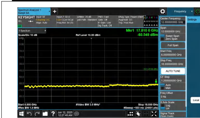
48-48-20MHz-15MHz-QPSK-QPSK-55916-56087-1RB#0-1RB#7 4-6000~18000MHz-PASS
