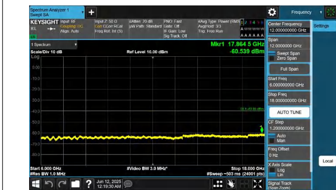
48-48-20MHz-10MHz-QPSK-QPSK-55941-56085-1RB#0-0RB#0- 6000~18000MHz-PASS
