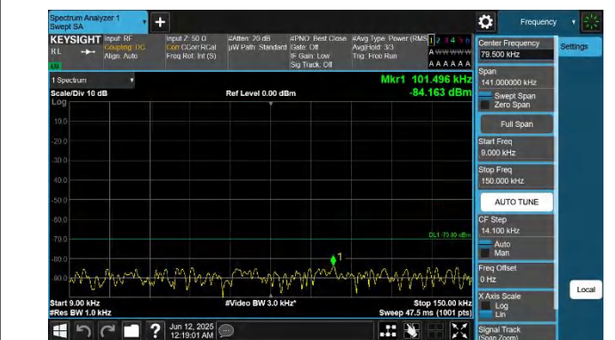
48-48-20MHz-10MHz-QPSK-QPSK-55941-56085-1RB#0-0RB#- 0.009~0.15MHz-PASS
