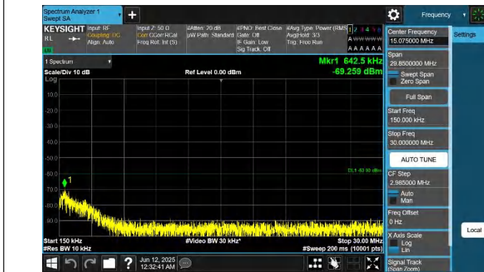
48-48-20MHz-20MHz-QPSK-QPSK-55891-56089-1RB#0-0RB#- 0.15~30MHz-PASS
