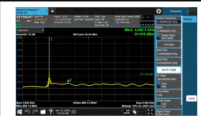
48-48-20MHz-20MHz-QPSK-QPSK-55891-56089-1RB#0-0RB#0- 3000~6000MHz-PASS
