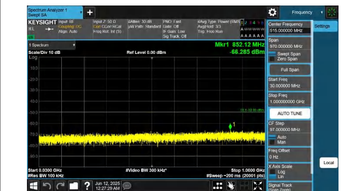
48-48-20MHz-15MHz-QPSK-QPSK-55916-56087-1RB#0-1RB#7 4-30~1000MHz-PASS
