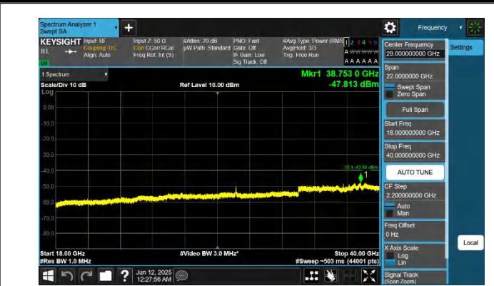
48-48-20MHz-15MHz-QPSK-QPSK-55916-56087-1RB#0-1RB#7 4-18000~40000MHz-PASS
