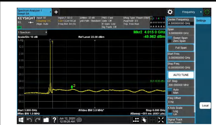
48-48-20MHz-15MHz-QPSK-QPSK-55340-55511-1RB#0-0RB#0- 3000~6000MHz-PASS
