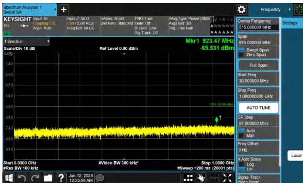
48-48-20MHz-15MHz-QPSK-QPSK-55916-56087-1RB#0-0RB#0- 30~1000MHz-PASS
