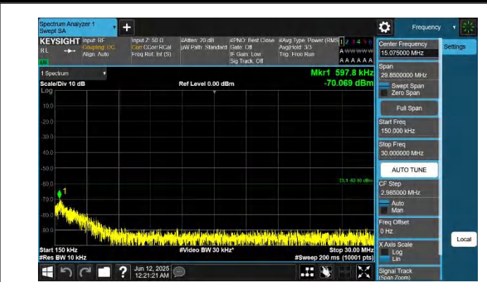
48-48-20MHz-10MHz-QPSK-QPSK-56541-56685-1RB#0-0RB#0- 0.15~30MHz-PASS
