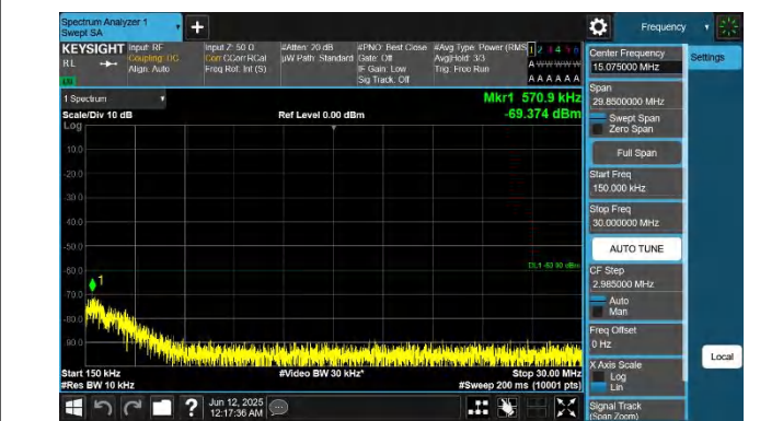
48-48-20MHz-10MHz-QPSK-QPSK-55340-55484-1RB#99-0RB# 0-0.15~30MHz-PASS
