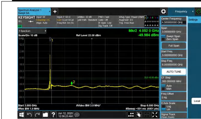
48-48-20MHz-10MHz-QPSK-QPSK-55340-55484-1RB#99-0RB# 0-3000~6000MHz-PASS
