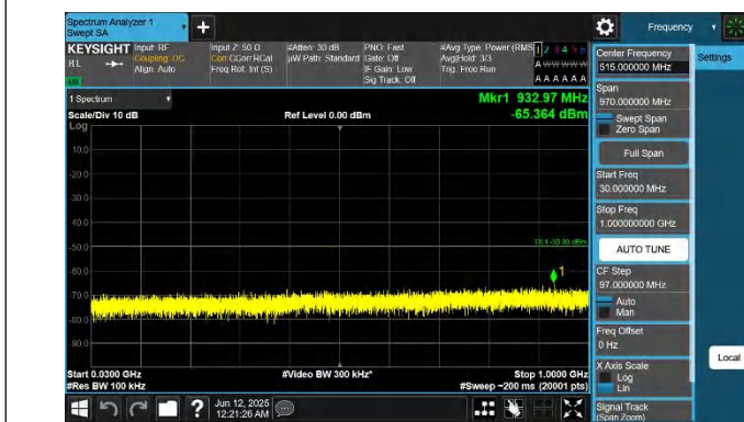
48-48-20MHz-10MHz-QPSK-QPSK-56541-56685-1RB#0-0RB#0- 30~1000MHz-PASS
