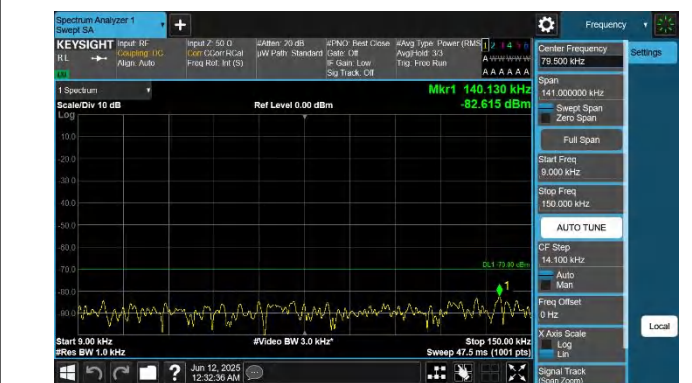
48-48-20MHz-20MHz-QPSK-QPSK-55891-56089-1RB#0-0RB#- 0.009~0.15MHz-PASS
