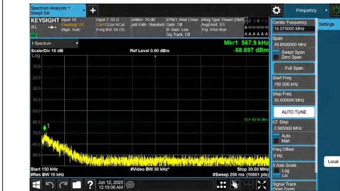
48-48-20MHz-10MHz-QPSK-QPSK-55941-56085-1RB#0-0RB#- 0.15~30MHz-PASS
