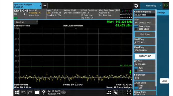
48-48-20MHz-20MHz-QPSK-QPSK-55891-56089-1RB#99-0RB# 0-0.009~0.15MHz-PASS
