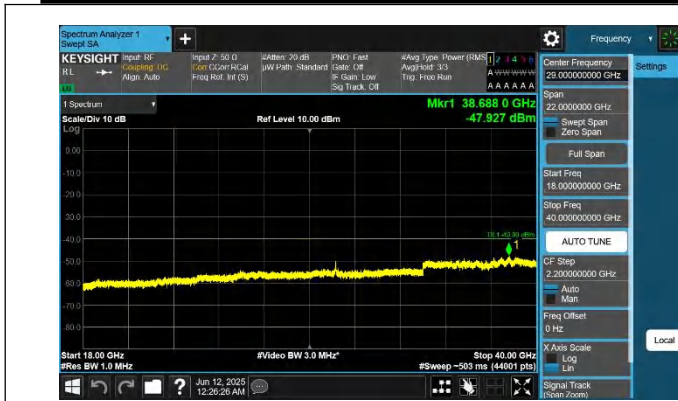
48-48-20MHz-15MHz-QPSK-QPSK-55916-56087-1RB#0-0RB#0- 18000~40000MHz-PASS
