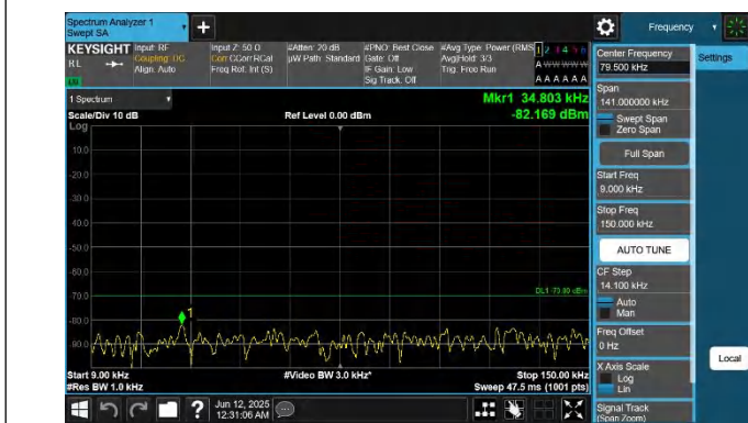
48-48-20MHz-20MHz-QPSK-QPSK-55340-55538-1RB#99-0RB# 0-0.009~0.15MHz-PASS
