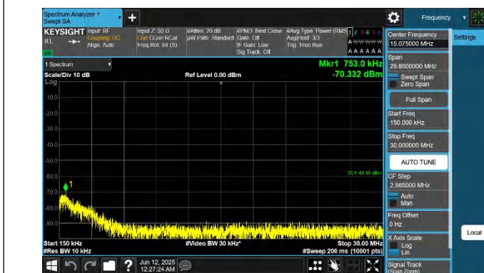
48-48-20MHz-15MHz-QPSK-QPSK-55916-56087-1RB#0-1RB#7 4-0.15~30MHz-PASS
