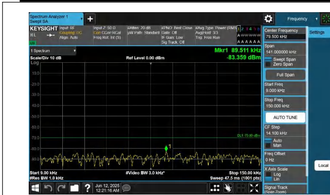
48-48-20MHz-10MHz-QPSK-QPSK-56541-56685-1RB#0-0RB#0- 0.009~0.15MHz-PASS
