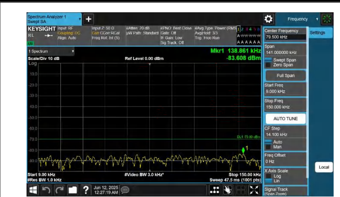
48-48-20MHz-15MHz-QPSK-QPSK-55916-56087-1RB#0-1RB#7 4-0.009~0.15MHz-PASS
