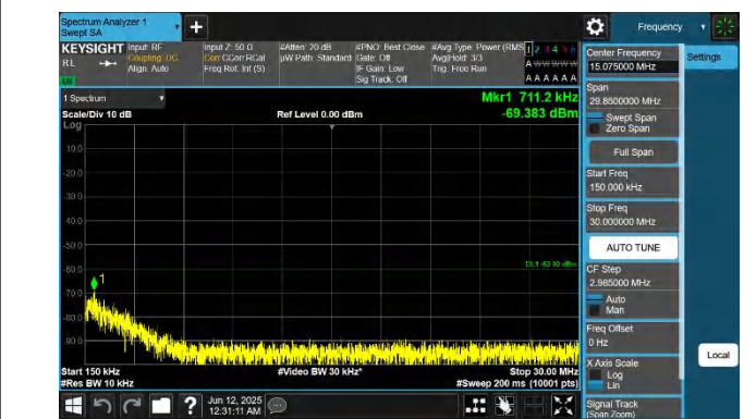
48-48-20MHz-20MHz-QPSK-QPSK-55340-55538-1RB#99-0RB# 0-0.15~30MHz-PASS
