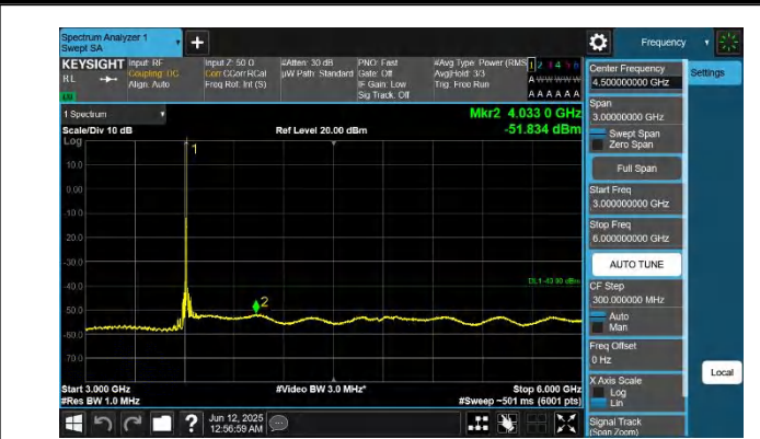
48-48-20MHz-10MHz-QPSK-QPSK-55941-56085-1RB#0-0RB#0- 3000~6000MHz-PASS
