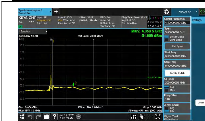
48-48-20MHz-20MHz-QPSK-QPSK-55340-55538-1RB#99-0RB# 0-3000~6000MHz-PASS
