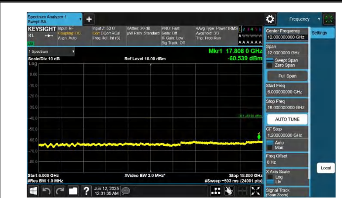
48-48-20MHz-20MHz-QPSK-QPSK-55340-55538-1RB#99-0RB# 0-6000~18000MHz-PASS
