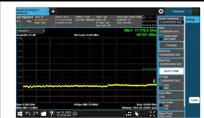
48-48-20MHz-10MHz-QPSK-QPSK-55340-55484-1RB#99-0RB# 0-6000~18000MHz-PASS
