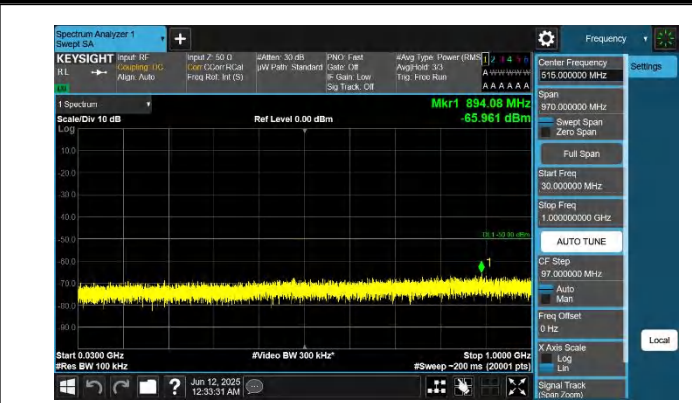
48-48-20MHz-20MHz-QPSK-QPSK-55891-56089-1RB#99-0RB# 0-30~1000MHz-PASS
