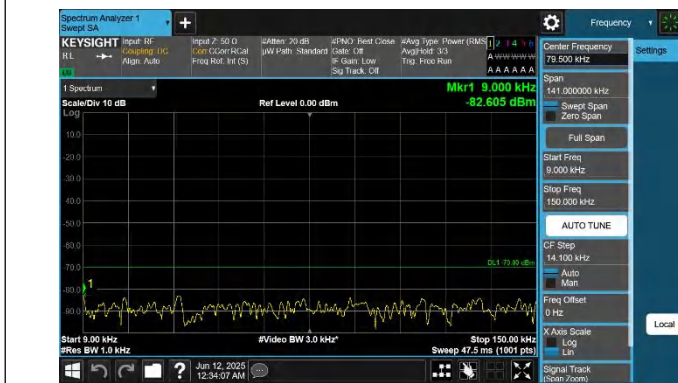
48-48-20MHz-20MHz-QPSK-QPSK-55891-56089-1RB#0-1RB#9 9-0.009~0.15MHz-PASS
