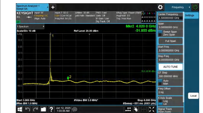
48-48-20MHz-20MHz-QPSK-QPSK-55891-56089-1RB#99-0RB# 0-3000~6000MHz-PASS
