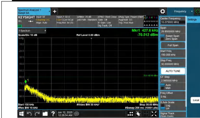
48-48-20MHz-15MHz-QPSK-QPSK-56491-56662-1RB#99-0RB# 0-0.15~30MHz-PASS
