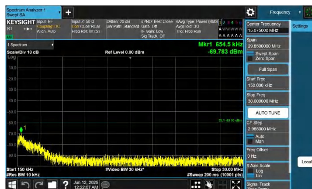
48-48-20MHz-10MHz-QPSK-QPSK-56541-56685-1RB#99-0RB# 0-0.15~30MHz-PASS
