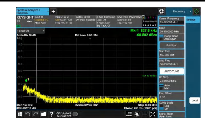
48-48-20MHz-20MHz-QPSK-QPSK-55340-55538-1RB#0-0RB#0- 0.15~30MHz-PASS
