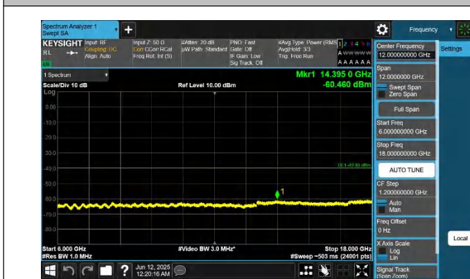
48-48-20MHz-10MHz-QPSK-QPSK-55941-56085-1RB#99-0RB# 0-6000~18000MHz-PASS
