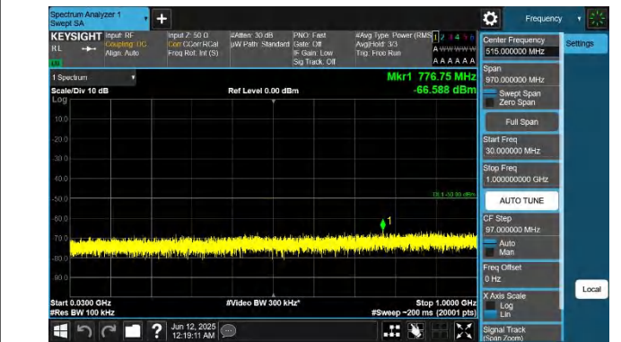
48-48-20MHz-10MHz-QPSK-QPSK-55941-56085-1RB#0-0RB#- 30~1000MHz-PASS
