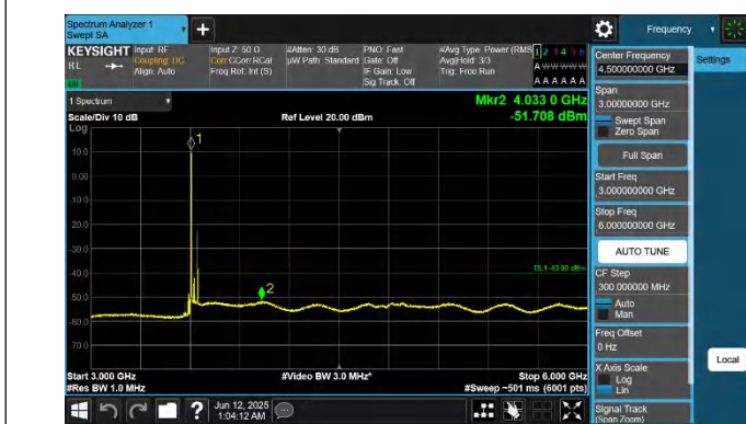
48-48-20MHz-20MHz-QPSK-QPSK-55891-56089-1RB#0-1RB#9 9-3000~6000MHz-PASS
