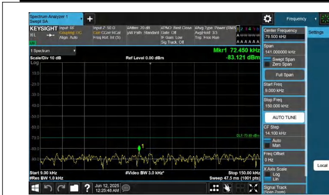
48-48-20MHz-15MHz-QPSK-QPSK-55916-56087-1RB#0-0RB#0- 0.009~0.15MHz-PASS
