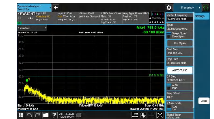
48-48-20MHz-15MHz-QPSK-QPSK-55916-56087-1RB#99-0RB# 0-0.15~30MHz-PASS
