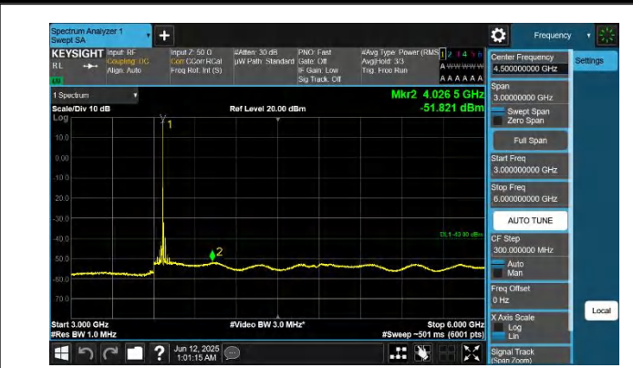
48-48-20MHz-15MHz-QPSK-QPSK-56491-56662-1RB#0-0RB#0- 3000~6000MHz-PASS
