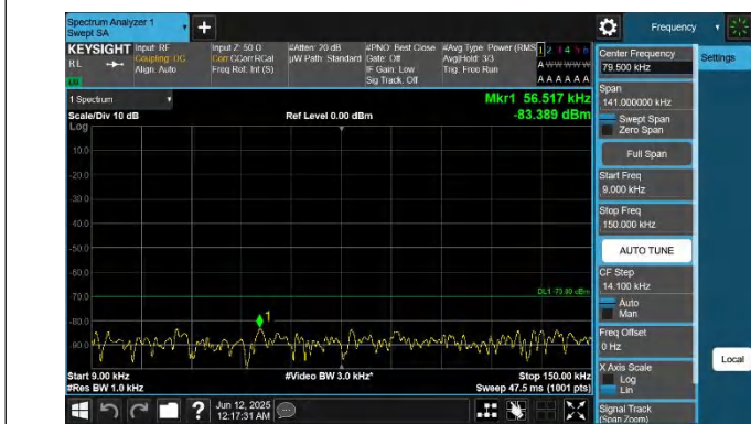
48-48-20MHz-10MHz-QPSK-QPSK-55340-55484-1RB#99-0RB# 0-0.009~0.15MHz-PASS
