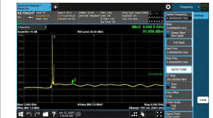
48-48-20MHz-15MHz-QPSK-QPSK-55916-56087-1RB#0-1RB#7 4-3000~6000MHz-PASS
