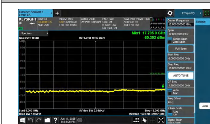
48-48-5MHz-20MHz-QPSK-QPSK-55898-56015-1RB#24-0RB#0- 6000~18000MHz-PASS
