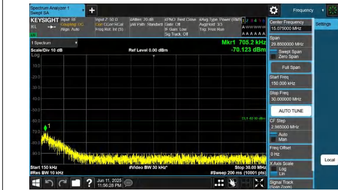
48-48-10MHz-20MHz-QPSK-QPSK-55295-55439-1RB#0-0RB#0- 0.15~30MHz-PASS
