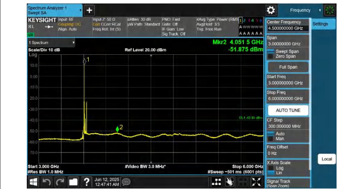
48-48-10MHz-20MHz-QPSK-QPSK-55896-56040-1RB#0-1RB#9-9.3000~6000MHz-PASS
