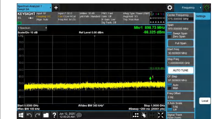
48-48-10MHz-20MHz-QPSK-QPSK-55896-56040-1RB#0-1RB#9-9.30~1000MHz-PASS
