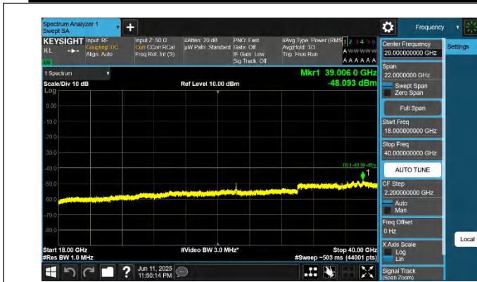
48-48-5MHz-20MHz-QPSK-QPSK-55273-55390-1RB#0-0RB#0-1 8000~40000MHz-PASS
