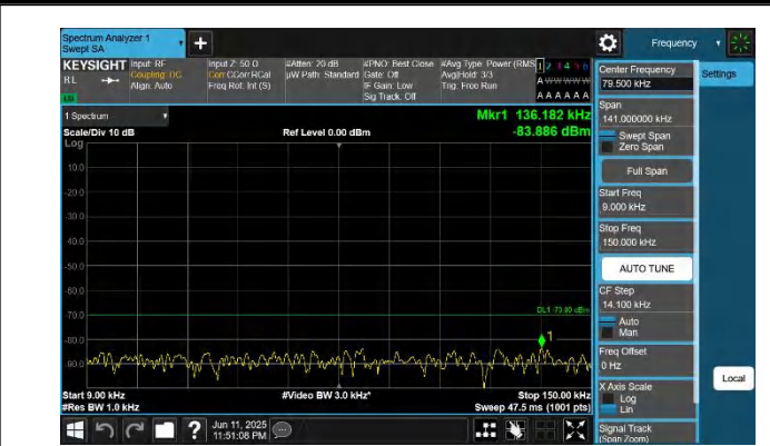
48-48-5MHz-20MHz-QPSK-QPSK-55273-55390-1RB#0-1RB#99- 0.009~0.15MHz-PASS
