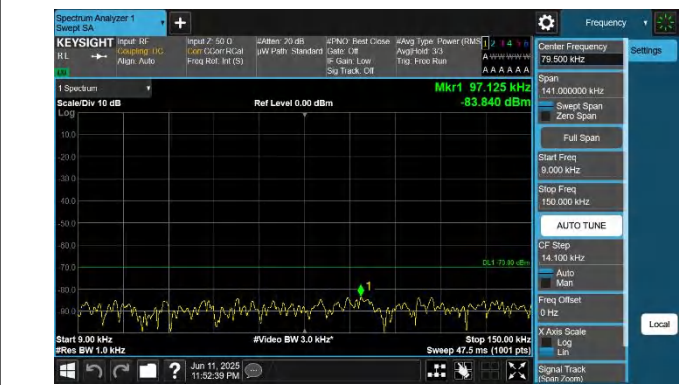
48-48-5MHz-20MHz-QPSK-QPSK-55898-56015-1RB#24-0RB#0- 0.009~0.15MHz-PASS
