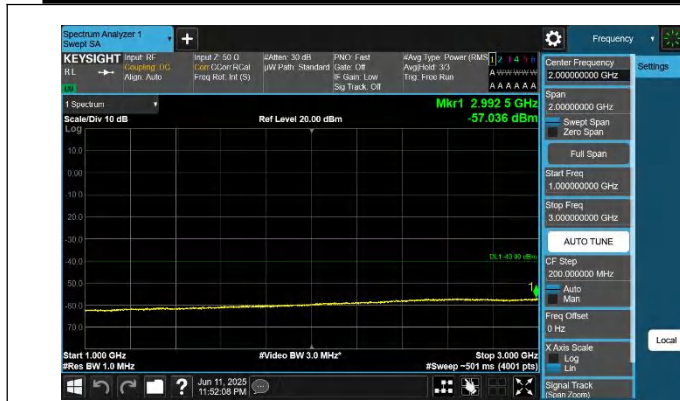
48-48-5MHz-20MHz-QPSK-QPSK-55898-56015-1RB#0-0RB#0-1 000~3000MHz-PASS
