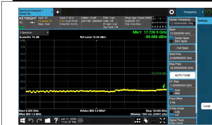
48-48-5MHz-20MHz-QPSK-QPSK-55273-55390-1RB#0-1RB#99- 6000~18000MHz-PASS
