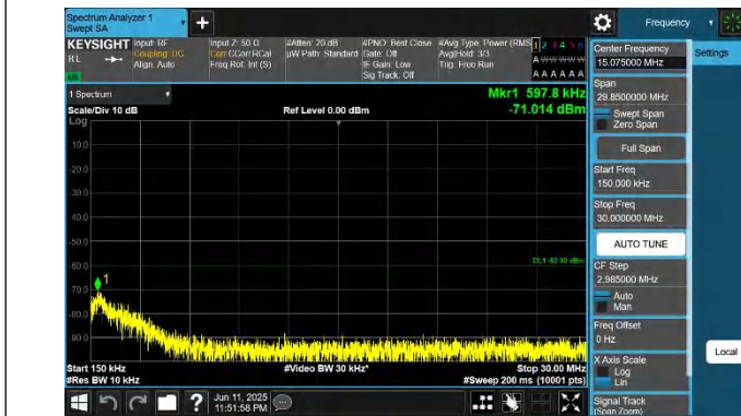
48-48-5MHz-20MHz-QPSK-QPSK-55898-56015-1RB#0-0RB#0-0 .15~30MHz-PASS
