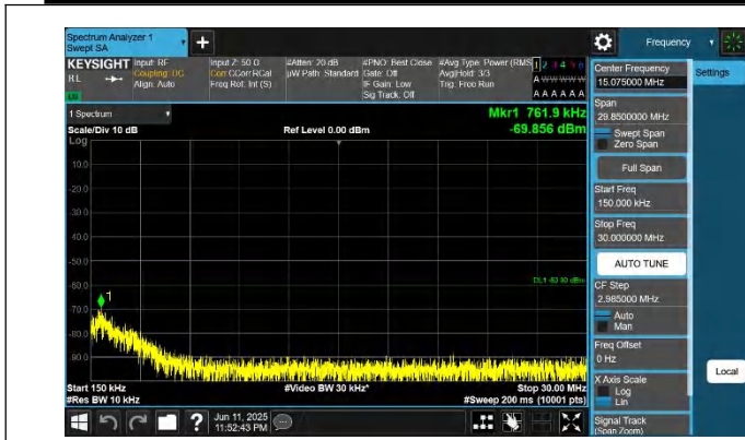
48-48-5MHz-20MHz-QPSK-QPSK-55898-56015-1RB#24-0RB#0- 0.15~30MHz-PASS
