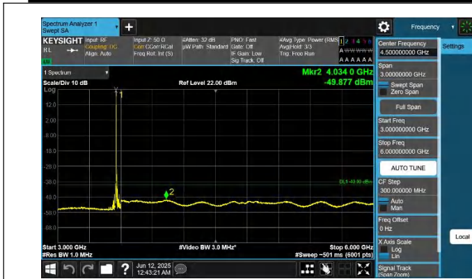
48-48-5MHz-20MHz-QPSK-QPSK-55273-55390-1RB#24-0RB#0- 3000~6000MHz-PASS
