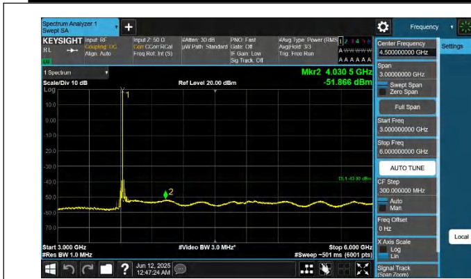
48-48-10MHz-20MHz-QPSK-QPSK-55896-56040-1RB#49-0RB# 0-3000~6000MHz-PASS
