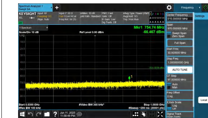
48-48-10MHz-20MHz-QPSK-QPSK-55896-56040-1RB#0-0RB#0- 30~1000MHz-PASS
