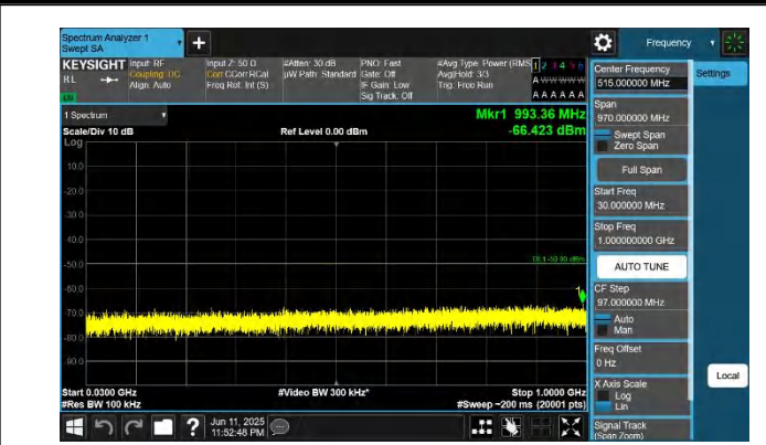
48-48-5MHz-20MHz-QPSK-QPSK-55898-56015-1RB#24-0RB#0- 30~1000MHz-PASS
