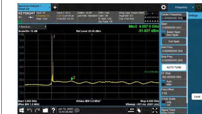
48-48-5MHz-20MHz-QPSK-QPSK-55898-56015-1RB#0-1RB#99- 3000~6000MHz-PASS
