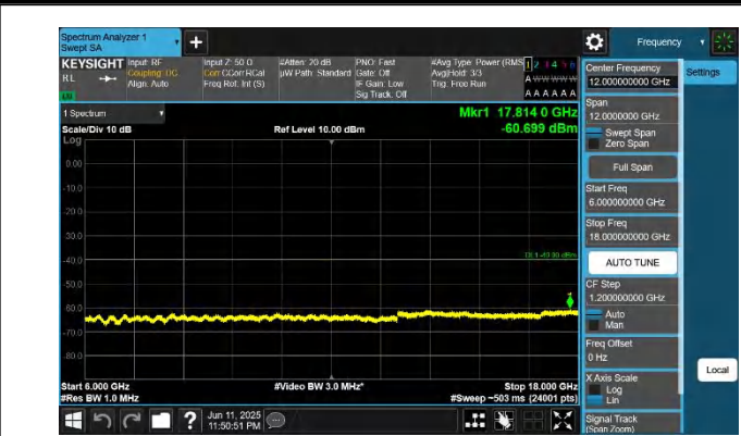
48-48-5MHz-20MHz-QPSK-QPSK-55273-55390-1RB#24-0RB#0- 6000~18000MHz-PASS
