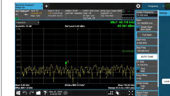
66-66-20MHz-20MHz-QPSK-QPSK-132374-132572-1RB#0-1RB #99-0.009~0.15MHz-PASS
