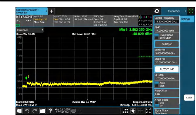
66-66-20MHz-10MHz-QPSK-QPSK-132473-132617-1RB#0-0RB #0-3000~20000MHz-PASS
