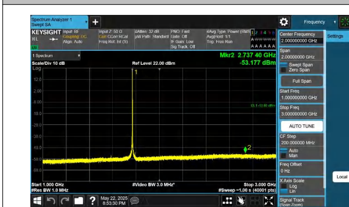
66-66-20MHz-10MHz-QPSK-QPSK-132473-132617-1RB#99-0R B#0-1000~3000MHz-PASS
