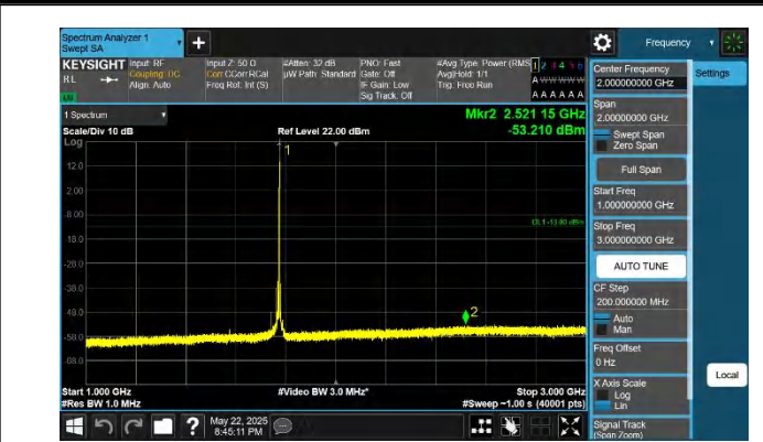
66-66-20MHz-5MHz-QPSK-QPSK-132522-132639-1RB#99-0RB #0-1000~3000MHz-PASS
