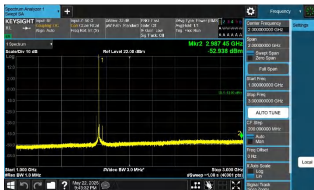
66-66-20MHz-20MHz-QPSK-QPSK-132072-132270-1RB#99-0R B#0-1000~3000MHz-PASS
