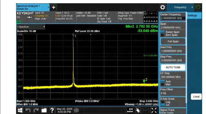
66-66-20MHz-10MHz-QPSK-QPSK-132373-132517-1RB#0-0RB #0-1000~3000MHz-PASS
