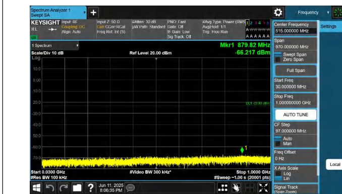
66-66-20MHz-10MHz-QPSK-QPSK-132373-132517-1RB#0-0RB #0-30~1000MHz-PASS
