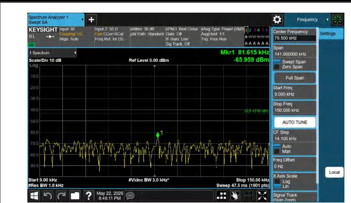
66-66-20MHz-10MHz-QPSK-QPSK-132072-132216-1RB#99-0R B#0-0.009~0.15MHz-PASS
