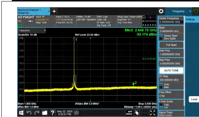
66-66-20MHz-10MHz-QPSK-QPSK-132473-132617-1RB#0-0RB #0-1000~3000MHz-PASS
