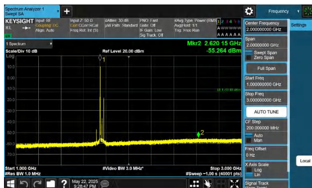
66-66-20MHz-15MHz-QPSK-QPSK-132423-132594-1RB#0-1RB #74-1000~3000MHz-PASS
