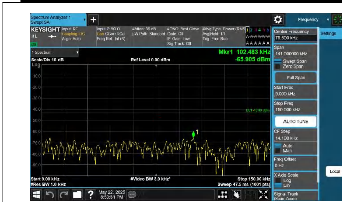
66-66-20MHz-10MHz-QPSK-QPSK-132373-132517-1RB#0-0RB #0-0.009~0.15MHz-PASS
