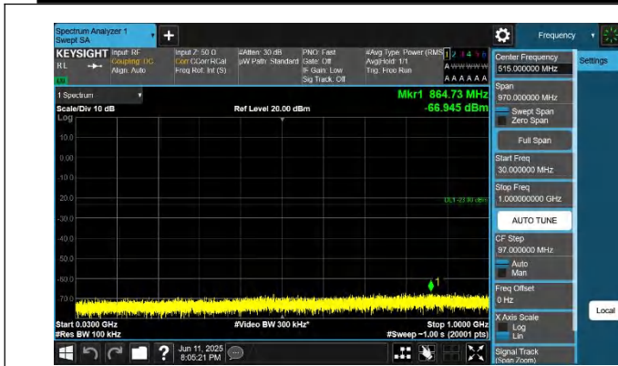
66-66-20MHz-5MHz-QPSK-QPSK-132522-132639-1RB#99-0RB #0-30~1000MHz-PASS
