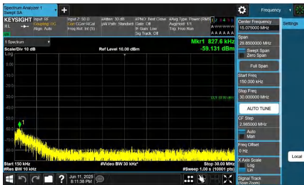
66-66-20MHz-20MHz-QPSK-QPSK-132374-132572-1RB#0-0RB #0-0.15~30MHz-PASS
