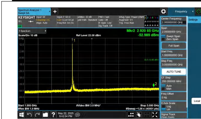
66-66-20MHz-20MHz-QPSK-QPSK-132072-132270-1RB#0-0RB #0-1000~3000MHz-PASS
