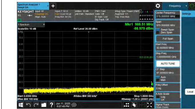
66-66-20MHz-10MHz-QPSK-QPSK-132473-132617-1RB#0-1RB #49-30~1000MHz-PASS
