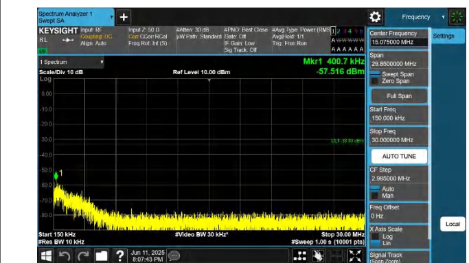
66-66-20MHz-10MHz-QPSK-QPSK-132473-132617-1RB#0-1RB #49-0.15~30MHz-PASS
