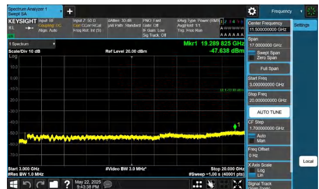
66-66-20MHz-20MHz-QPSK-QPSK-132072-132270-1RB#99-0R B#0-3000~20000MHz-PASS
