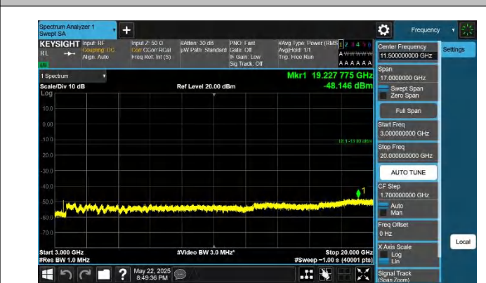
66-66-20MHz-10MHz-QPSK-QPSK-132072-132216-1RB#99-0R B#0-3000~20000MHz-PASS
