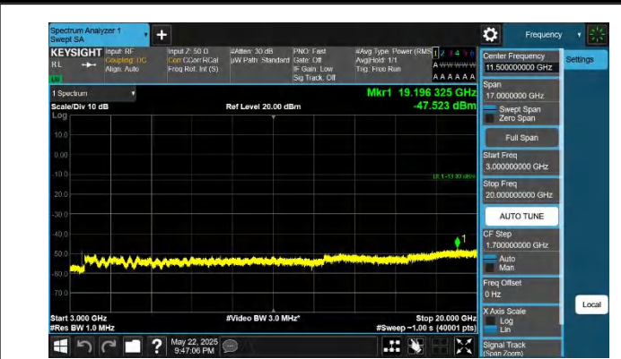
66-66-20MHz-20MHz-QPSK-QPSK-132374-132572-1RB#0-0RB #0-3000~20000MHz-PASS
