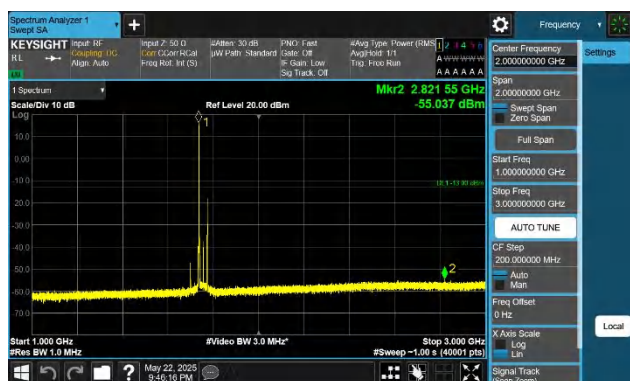
66-66-20MHz-20MHz-QPSK-QPSK-132323-132521-1RB#0-1RB #99-1000~3000MHz-PASS
