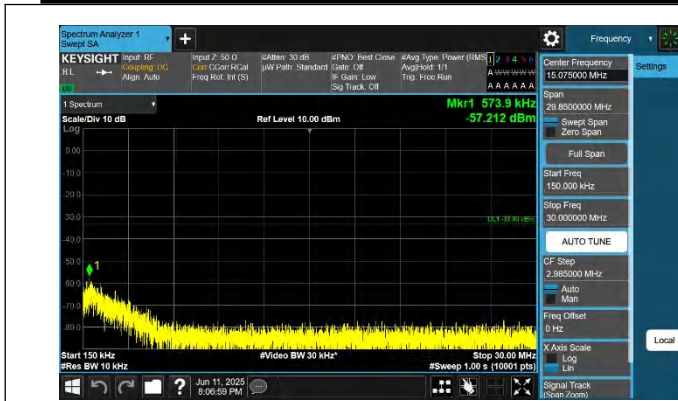
66-66-20MHz-10MHz-QPSK-QPSK-132373-132517-1RB#0-1RB #49-0.15~30MHz-PASS
