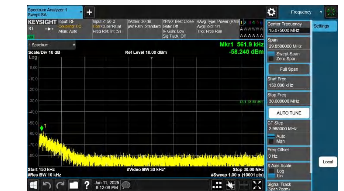
66-66-20MHz-20MHz-QPSK-QPSK-132374-132572-1RB#0-1RB #99-0.15~30MHz-PASS
