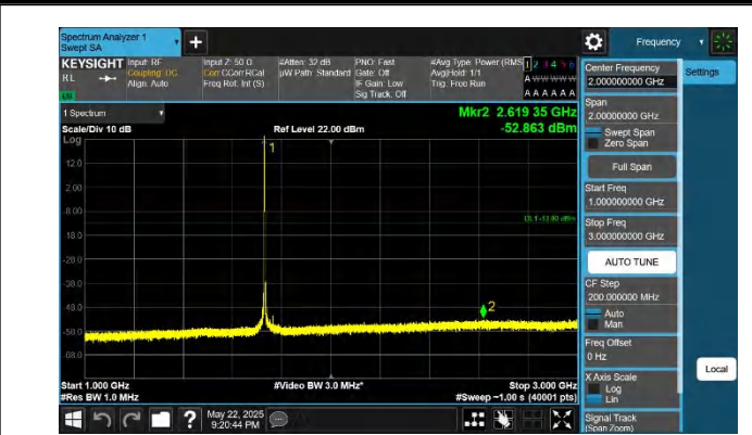
66-66-20MHz-15MHz-QPSK-QPSK-132072-132243-1RB#99-0R B#0-1000~3000MHz-PASS
