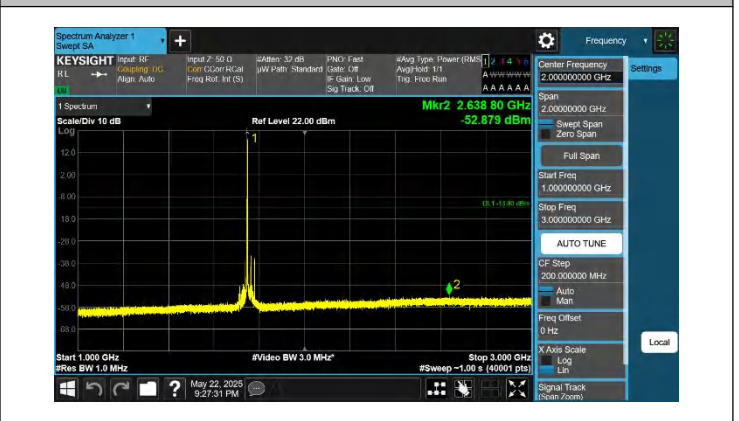
66-66-20MHz-15MHz-QPSK-QPSK-132423-132594-1RB#0-0RB #0-1000~3000MHz-PASS
