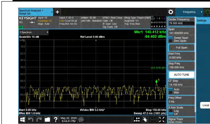
66-66-20MHz-20MHz-QPSK-QPSK-132323-132521-1RB#0-0RB #0-0.009~0.15MHz-PASS
