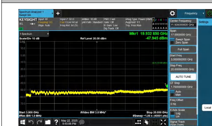
66-66-20MHz-20MHz-QPSK-QPSK-132323-132521-1RB#0-0RB #0-3000~20000MHz-PASS
