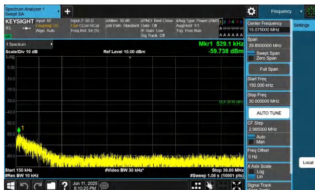
66-66-20MHz-20MHz-QPSK-QPSK-132072-132270-1RB#99-0R B#0-0.15~30MHz-PASS
