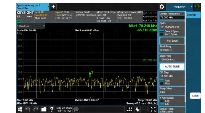
66-66-20MHz-10MHz-QPSK-QPSK-132373-132517-1RB#0-1RB #49-0.009~0.15MHz-PASS
