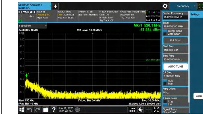
66-66-20MHz-10MHz-QPSK-QPSK-132072-132216-1RB#0-0RB #0-0.15~30MHz-PASS
