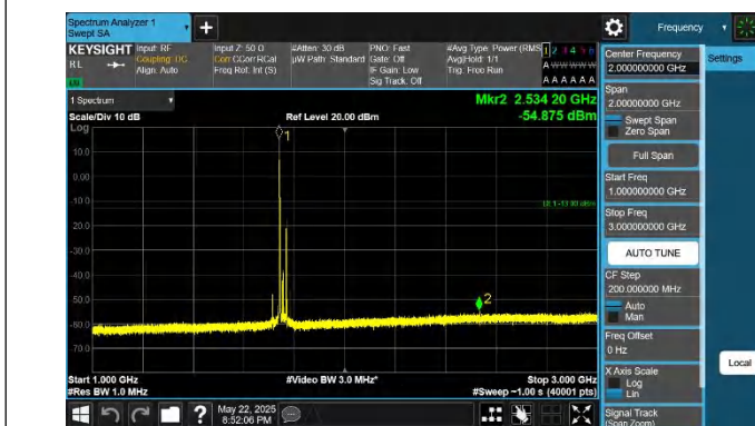
66-66-20MHz-10MHz-QPSK-QPSK-132373-132517-1RB#0-1RB #49-1000~3000MHz-PASS
