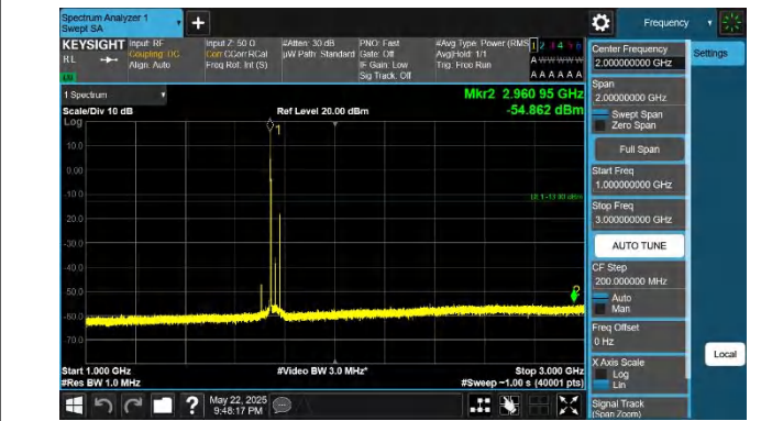
66-66-20MHz-20MHz-QPSK-QPSK-132374-132572-1RB#0-1RB #99-1000~3000MHz-PASS
