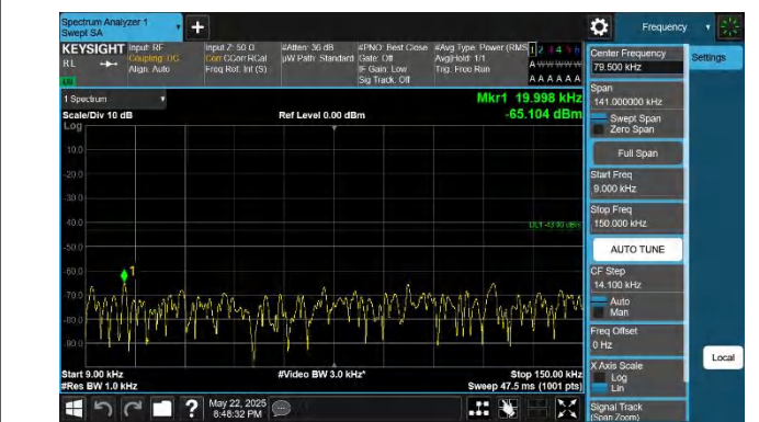
66-66-20MHz-10MHz-QPSK-QPSK-132072-132216-1RB#0-0RB #0-0.009~0.15MHz-PASS
