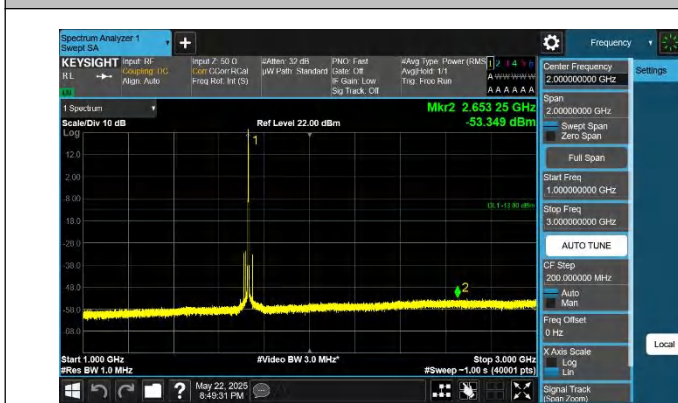
66-66-20MHz-10MHz-QPSK-QPSK-132072-132216-1RB#99-0R B#0-1000~3000MHz-PASS
