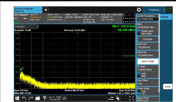
66-66-20MHz-10MHz-QPSK-QPSK-132373-132517-1RB#0-0RB #0-0.15~30MHz-PASS
