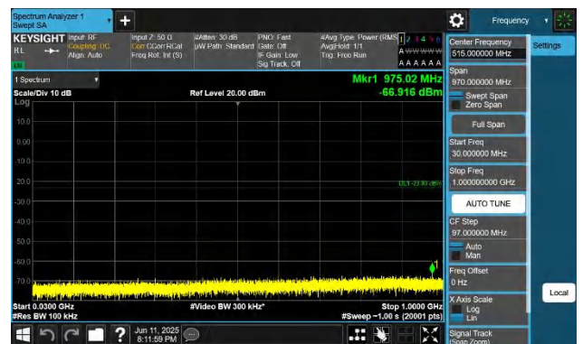
66-66-20MHz-20MHz-QPSK-QPSK-132374-132572-1RB#99-0R B#0-30~1000MHz-PASS
