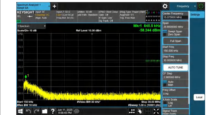
66-66-20MHz-10MHz-QPSK-QPSK-132373-132517-1RB#99-0R B#0-0.15~30MHz-PASS
