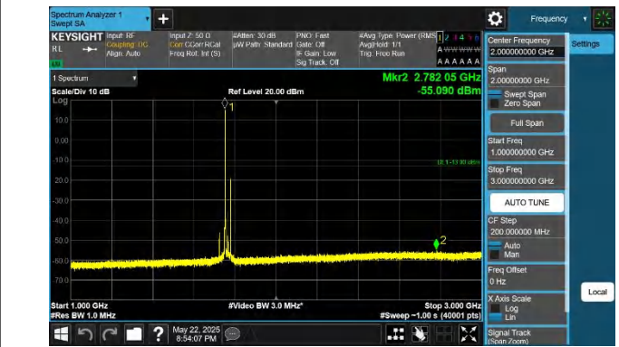
66-66-20MHz-10MHz-QPSK-QPSK-132473-132617-1RB#0-1RB #49-1000~3000MHz-PASS
