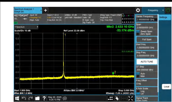
66-66-20MHz-15MHz-QPSK-QPSK-132423-132594-1RB#99-0R B#0-1000~3000MHz-PASS
