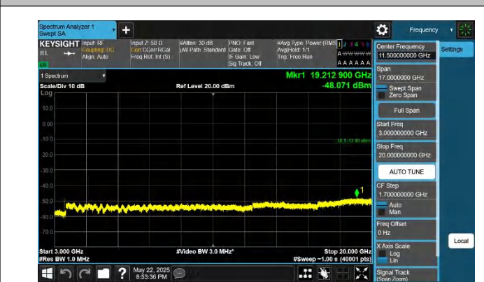
66-66-20MHz-10MHz-QPSK-QPSK-132473-132617-1RB#99-0R B#0-3000~20000MHz-PASS
