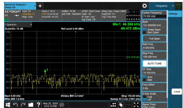
66-66-20MHz-20MHz-QPSK-QPSK-132072-132270-1RB#99-0R B#0-0.009~0.15MHz-PASS
