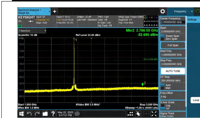
66-66-20MHz-20MHz-QPSK-QPSK-132374-132572-1RB#0-0RB #0-1000~3000MHz-PASS
