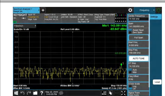
66-66-20MHz-20MHz-QPSK-QPSK-132323-132521-1RB#0-1RB #99-0.009~0.15MHz-PASS
