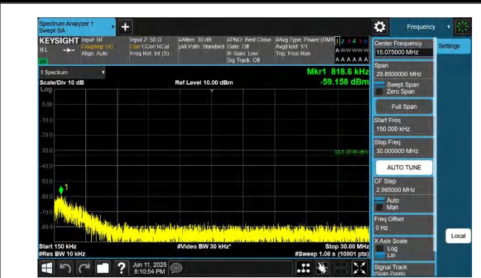
66-66-20MHz-20MHz-QPSK-QPSK-132323-132521-1RB#0-0RB #0-0.15~30MHz-PASS
