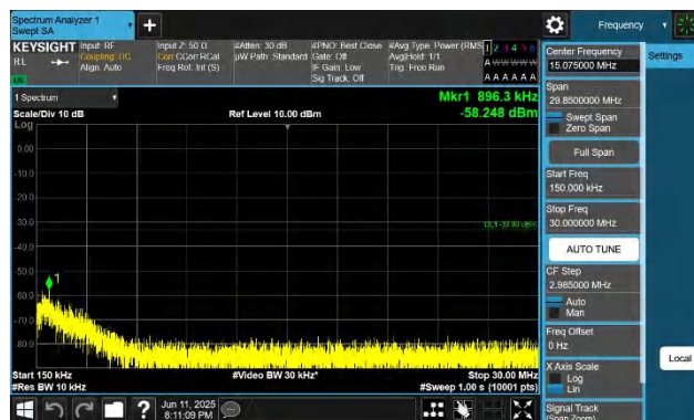
66-66-20MHz-20MHz-QPSK-QPSK-132323-132521-1RB#99-0R B#0-0.15~30MHz-PASS
