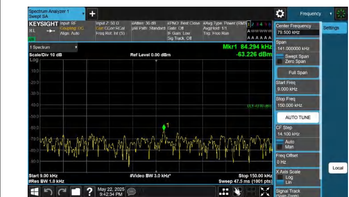
66-66-20MHz-20MHz-QPSK-QPSK-132072-132270-1RB#0-0RB #0-0.009~0.15MHz-PASS
