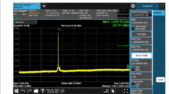
66-66-20MHz-15MHz-QPSK-QPSK-132072-132243-1RB#0-0RB #0-1000~3000MHz-PASS
