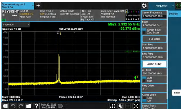
66-66-20MHz-5MHz-QPSK-QPSK-132522-132639-1RB#0-1RB# 24-1000~3000MHz-PASS
