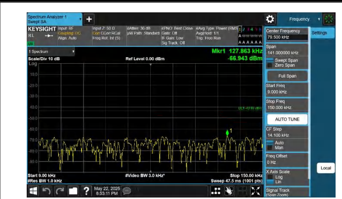
66-66-20MHz-10MHz-QPSK-QPSK-132473-132617-1RB#99-0R B#0-0.009~0.15MHz-PASS
