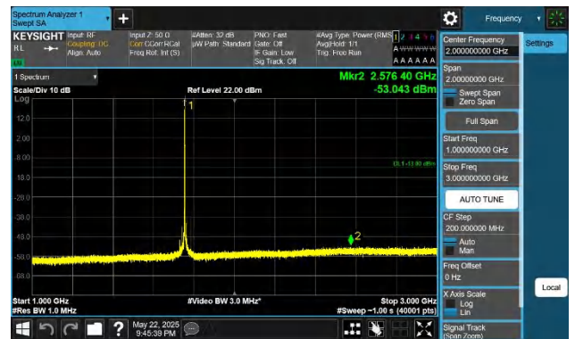
66-66-20MHz-20MHz-QPSK-QPSK-132323-132521-1RB#99-0R B#0-1000~3000MHz-PASS
