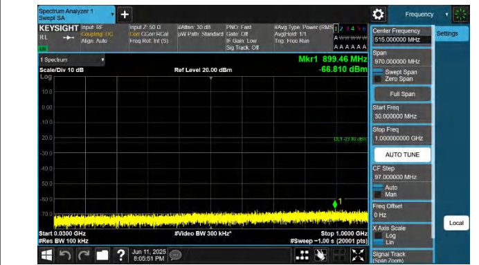
66-66-20MHz-10MHz-QPSK-QPSK-132072-132216-1RB#0-0RB #0-30~1000MHz-PASS
