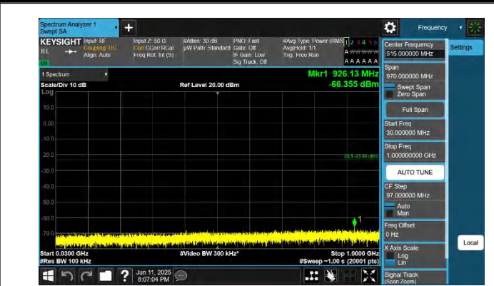
66-66-20MHz-10MHz-QPSK-QPSK-132373-132517-1RB#0-1RB #49-30~1000MHz-PASS
