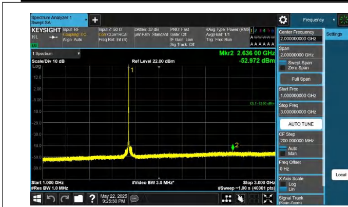
66-66-20MHz-15MHz-QPSK-QPSK-132348-132519-1RB#0-0RB #0-1000~3000MHz-PASS
