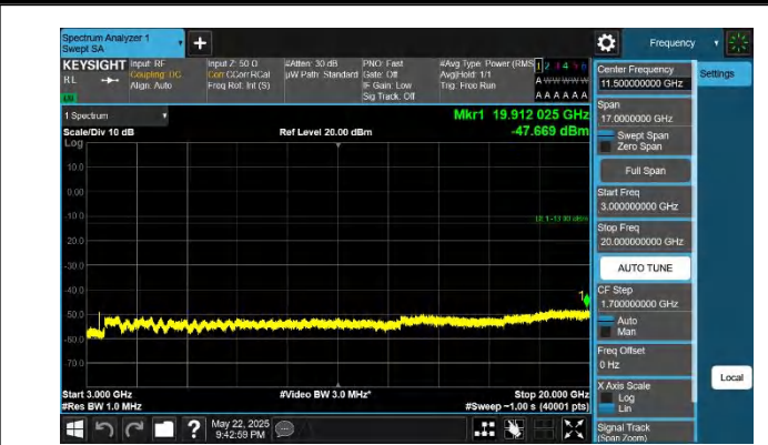
66-66-20MHz-20MHz-QPSK-QPSK-132072-132270-1RB#0-0RB #0-3000~20000MHz-PASS
