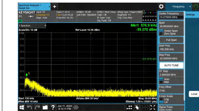
66-66-20MHz-20MHz-QPSK-QPSK-132072-132270-1RB#0-0RB #0-0.15~30MHz-PASS
