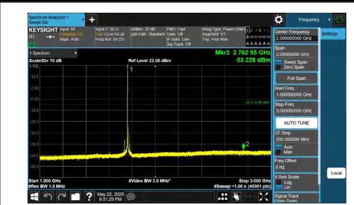
66-66-20MHz-10MHz-QPSK-QPSK-132373-132517-1RB#99-0R B#0-1000~3000MHz-PASS
