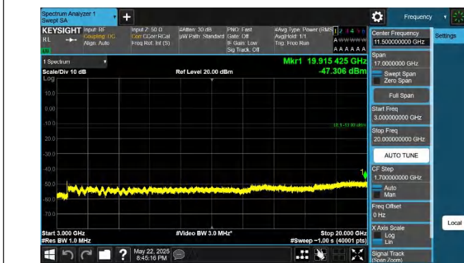
66-66-20MHz-5MHz-QPSK-QPSK-132522-132639-1RB#99-0RB #0-3000~20000MHz-PASS
