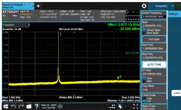
66-66-20MHz-20MHz-QPSK-QPSK-132374-132572-1RB#99-0R B#0-1000~3000MHz-PASS
