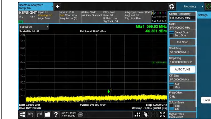
66-66-20MHz-20MHz-QPSK-QPSK-132374-132572-1RB#0-1RB #99-30~1000MHz-PASS
