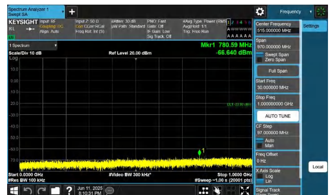
66-66-20MHz-20MHz-QPSK-QPSK-132072-132270-1RB#99-0R B#0-30~1000MHz-PASS
