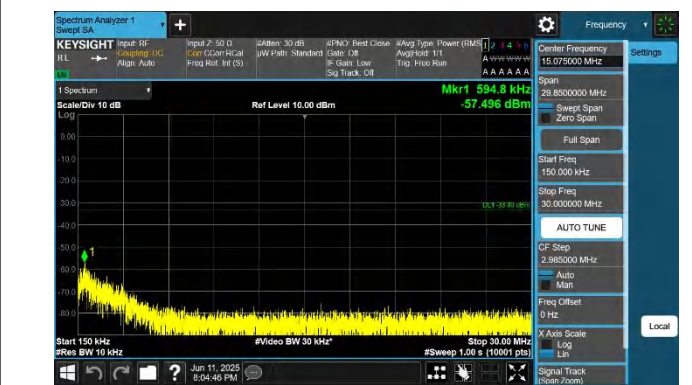
66-66-20MHz-5MHz-QPSK-QPSK-132397-132514-1RB#0-1RB# 24-0.15~30MHz-PASS
