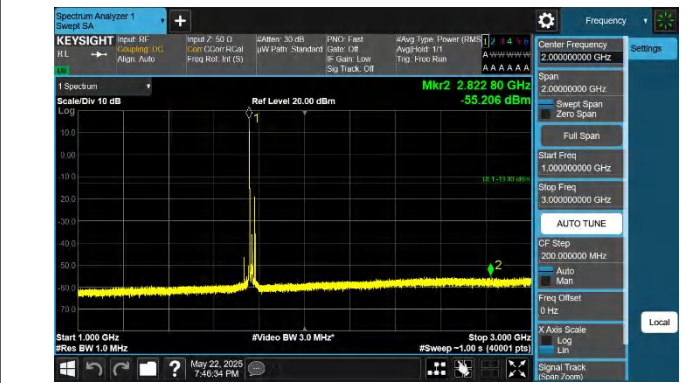
66-66-15MHz-10MHz-QPSK-QPSK-132499-132619-1RB#0-1RB #49-1000~3000MHz-PASS
