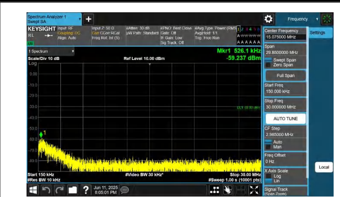
66-66-20MHz-5MHz-QPSK-QPSK-132522-132639-1RB#0-0RB# 0-0.15~30MHz-PASS
