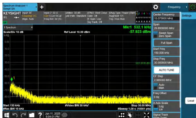
66-66-20MHz-5MHz-QPSK-QPSK-132072-132189-1RB#0-1RB# 24-0.15~30MHz-PASS
