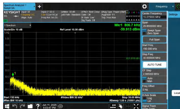
66-66-20MHz-5MHz-QPSK-QPSK-132072-132189-1RB#99-0RB #0-0.15~30MHz-PASS
