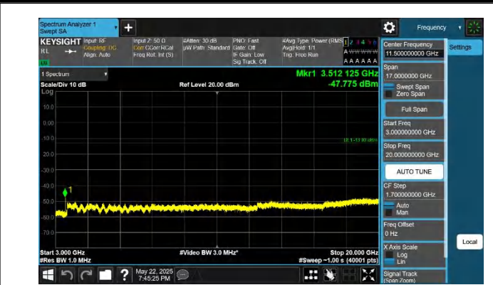
66-66-15MHz-10MHz-QPSK-QPSK-132499-132619-1RB#0-0RB #0-3000~20000MHz-PASS
