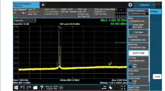
66-66-15MHz-20MHz-QPSK-QPSK-132401-132572-1RB#0-1RB #99-1000~3000MHz-PASS
