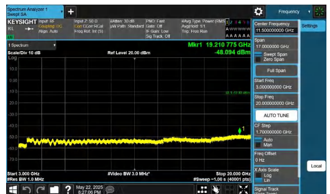
66-66-15MHz-20MHz-QPSK-QPSK-132325-132496-1RB#0-1RB #99-3000~20000MHz-PASS
