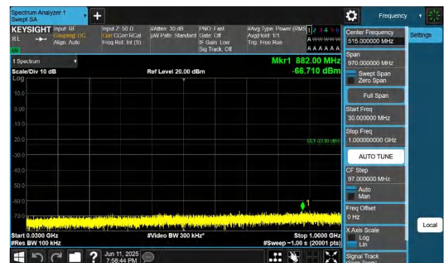
66-66-15MHz-10MHz-QPSK-QPSK-132499-132619-1RB#74-0R B#0-30~1000MHz-PASS
