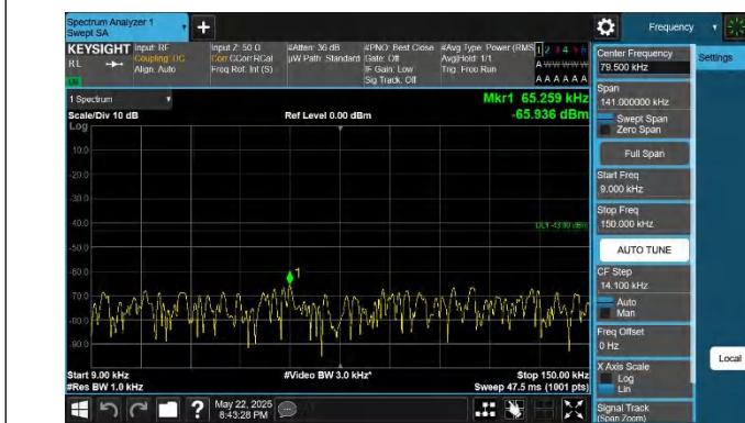
66-66-20MHz-5MHz-QPSK-QPSK-132397-132514-1RB#0-1RB# 24-0.009~0.15MHz-PASS
