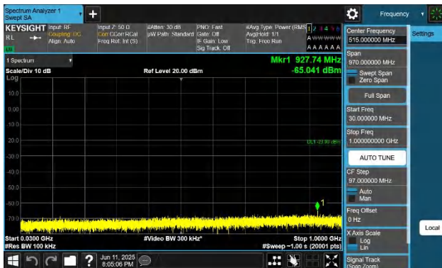
66-66-20MHz-5MHz-QPSK-QPSK-132522-132639-1RB#0-0RB# 0-30~1000MHz-PASS
