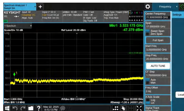
66-66-20MHz-5MHz-QPSK-QPSK-132397-132514-1RB#99-0RB #0-3000~20000MHz-PASS
