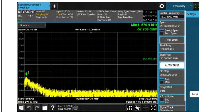
66-66-20MHz-5MHz-QPSK-QPSK-132397-132514-1RB#0-ORB# 0-0.15~30MHz-PASS
