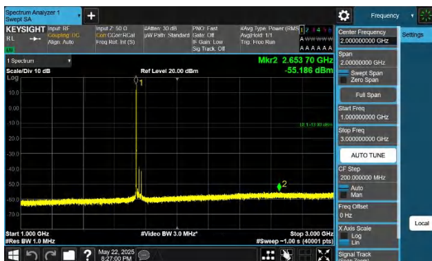
66-66-15MHz-20MHz-QPSK-QPSK-132325-132496-1RB#0-1RB #99-1000~3000MHz-PASS
