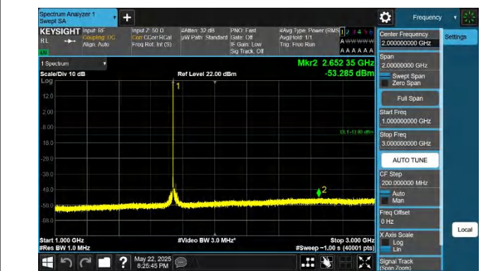
66-66-15MHz-20MHz-QPSK-QPSK-132325-132496-1RB#0-0RB #0-1000~3000MHz-PASS
