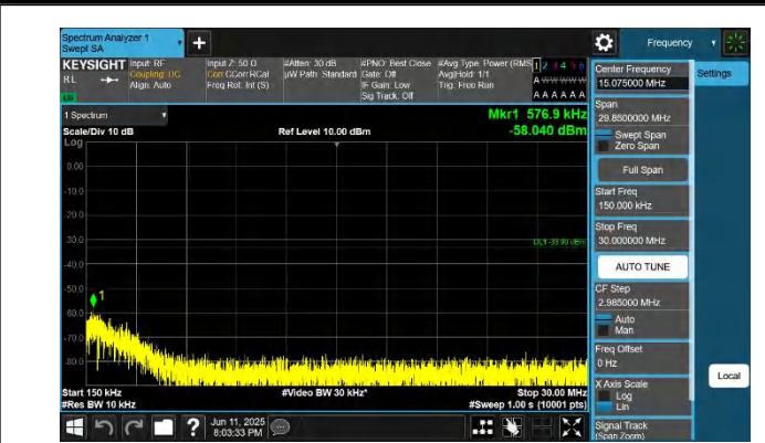
66-66-20MHz-5MHz-QPSK-QPSK-132072-132189-1RB#0-0RB# 0-0.15~30MHz-PASS
