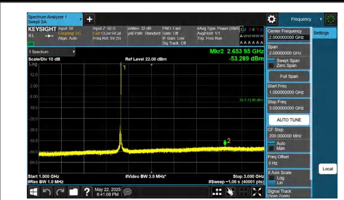
66-66-20MHz-5MHz-QPSK-QPSK-132072-132189-1RB#99-ORB #0-1000~3000MHz-PASS
