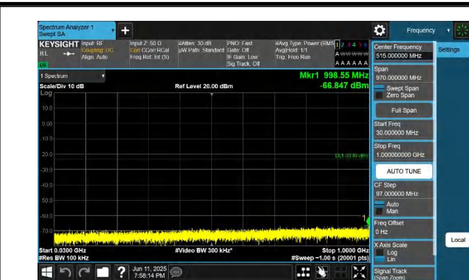
66-66-15MHz-10MHz-QPSK-QPSK-132373-132493-1RB#0-1RB #49-30~1000MHz-PASS
