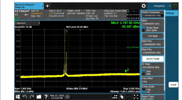
66-66-20MHz-5MHz-QPSK-QPSK-132397-132514-1RB#0-1RB# 24-1000~3000MHz-PASS
