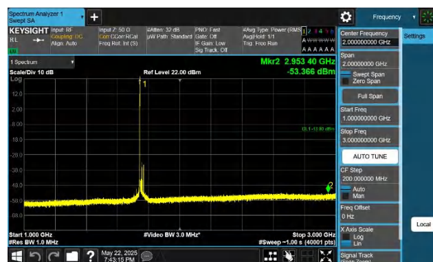
66-66-15MHz-10MHz-QPSK-QPSK-132373-132493-1RB#0-0RB #0-1000~3000MHz-PASS
