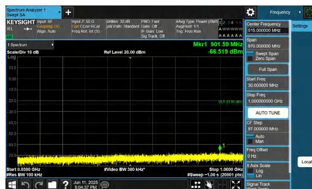
66-66-20MHz-5MHz-QPSK-QPSK-132397-132514-1RB#99-0RB #0-30~1000MHz-PASS
