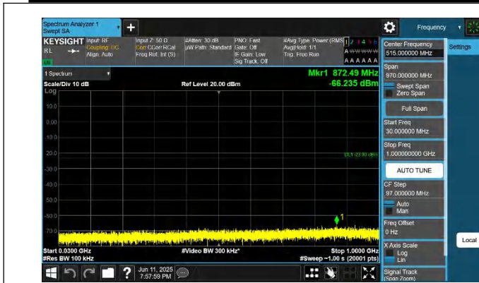
66-66-15MHz-10MHz-QPSK-QPSK-132373-132493-1RB#74-0R B#0-30~1000MHz-PASS
