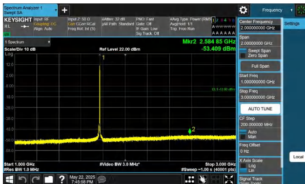
66-66-15MHz-10MHz-QPSK-QPSK-132499-132619-1RB#74-0R B#0-1000~3000MHz-PASS
