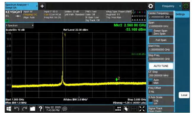
66-66-15MHz-10MHz-QPSK-QPSK-132373-132493-1RB#74-0R B#0-1000~3000MHz-PASS
