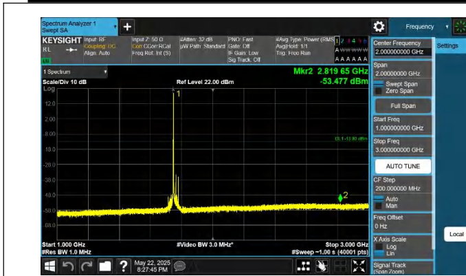
66-66-15MHz-20MHz-QPSK-QPSK-132401-132572-1RB#0-0RB #0-1000~3000MHz-PASS
