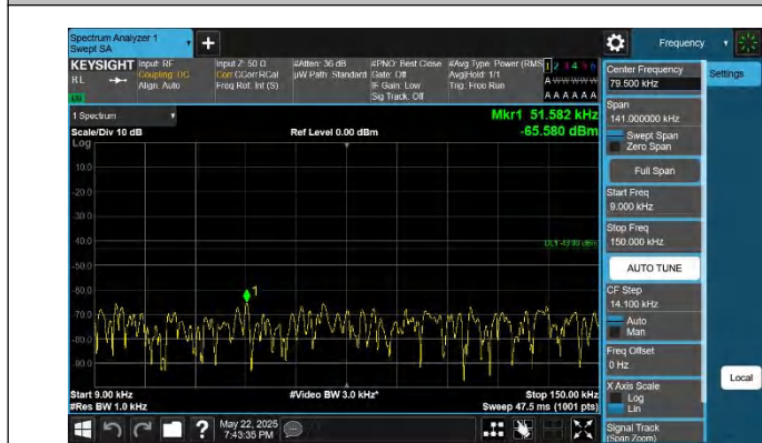
66-66-15MHz-10MHz-QPSK-QPSK-132373-132493-1RB#74-0R B#0-0.009~0.15MHz-PASS
