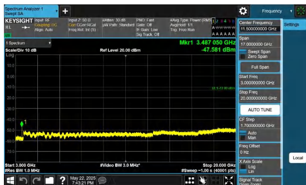
66-66-15MHz-10MHz-QPSK-QPSK-132373-132493-1RB#0-0RB #0-3000~20000MHz-PASS
