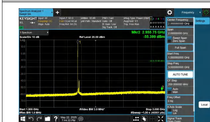
66-66-15MHz-10MHz-QPSK-QPSK-132373-132493-1RB#0-1RB #49-1000~3000MHz-PASS
