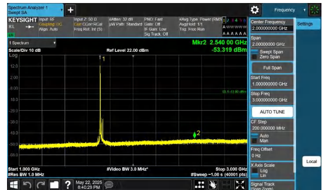
66-66-20MHz-5MHz-QPSK-QPSK-132072-132189-1RB#0-0RB# 0-1000~3000MHz-PASS
