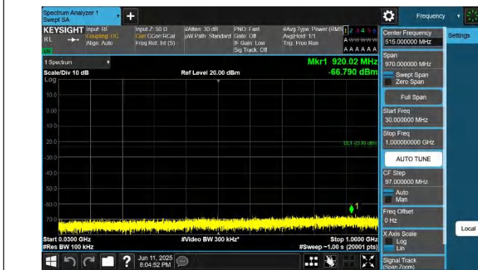
66-66-20MHz-5MHz-QPSK-QPSK-132397-132514-1RB#0-1RB# 24-30~1000MHz-PASS
