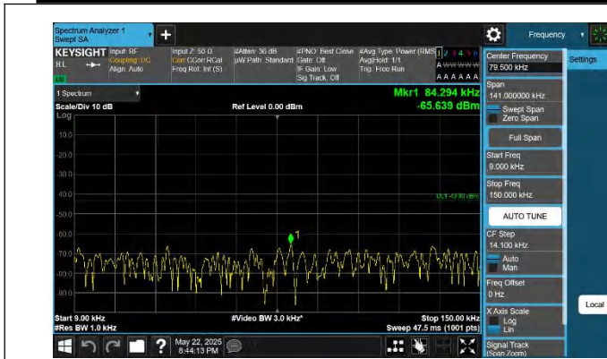
66-66-20MHz-5MHz-QPSK-QPSK-132522-132639-1RB#0-0RB# 0-0.009~0.15MHz-PASS
