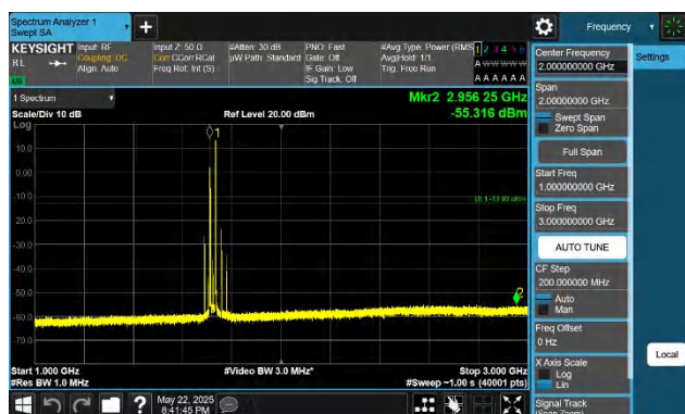
66-66-20MHz-5MHz-QPSK-QPSK-132072-132189-1RB#0-1RB# 24-1000~3000MHz-PASS
