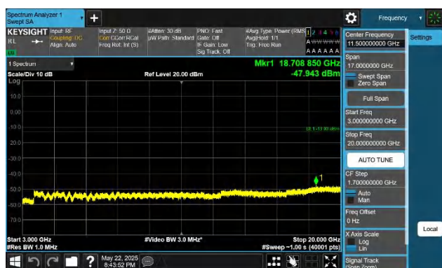
66-66-20MHz-5MHz-QPSK-QPSK-132397-132514-1RB#0-1RB# 24-3000~20000MHz-PASS
