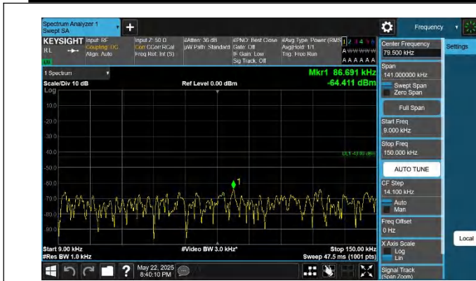
66-66-20MHz-5MHz-QPSK-QPSK-132072-132189-1RB#0-0RB# 0-0.009~0.15MHz-PASS
