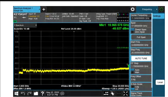
66-66-15MHz-20MHz-QPSK-QPSK-132401-132572-1RB#0-0RB #0-3000~20000MHz-PASS
