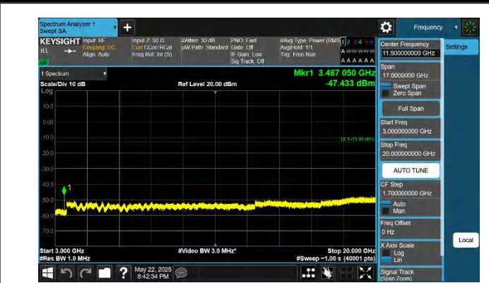
66-66-20MHz-5MHz-QPSK-QPSK-132397-132514-1RB#0-0RB# 0-3000~20000MHz-PASS
