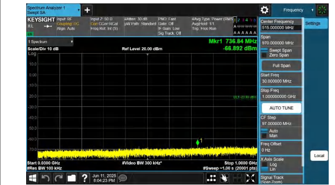
66-66-20MHz-5MHz-QPSK-QPSK-132397-132514-1RB#0-ORB# 0-30~1000MHz-PASS
