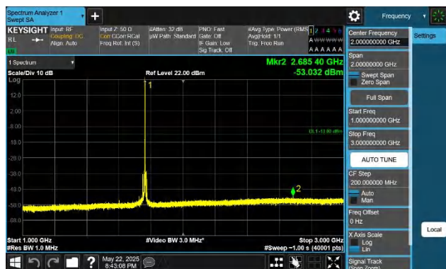
66-66-20MHz-5MHz-QPSK-QPSK-132397-132514-1RB#99-0RB #0-1000~3000MHz-PASS
