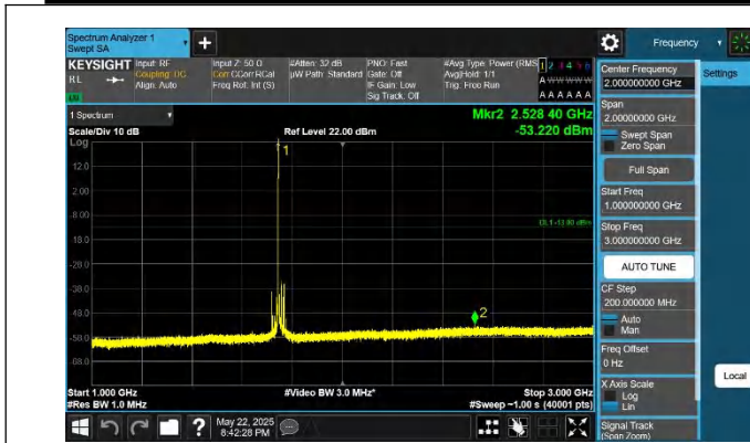
66-66-20MHz-5MHz-QPSK-QPSK-132397-132514-1RB#0-0RB# 0-1000~3000MHz-PASS
