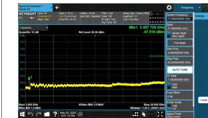
66-66-20MHz-5MHz-QPSK-QPSK-132072-132189-1RB#99-ORB #0-3000~20000MHz-PASS
