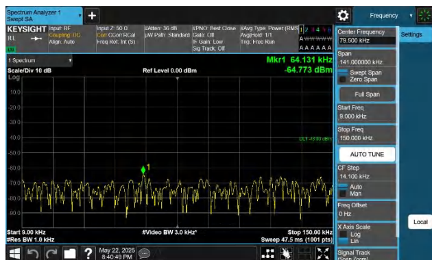
66-66-20MHz-5MHz-QPSK-QPSK-132072-132189-1RB#99-0RB #0-0.009~0.15MHz-PASS
