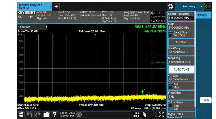
66-66-15MHz-20MHz-QPSK-QPSK-132401-132572-1RB#0-0RB #0-30~1000MHz-PASS
