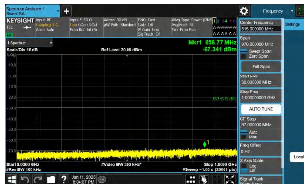
66-66-20MHz-5MHz-QPSK-QPSK-132072-132189-1RB#0-1RB# 24-30~1000MHz-PASS
