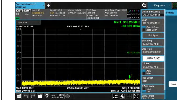
66-66-15MHz-20MHz-QPSK-QPSK-132401-132572-1RB#0-1RB #99-30~1000MHz-PASS
