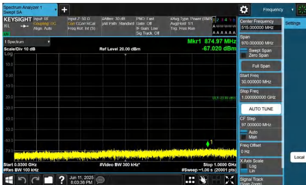
66-66-20MHz-5MHz-QPSK-QPSK-132072-132189-1RB#0-0RB# 0-30~1000MHz-PASS
