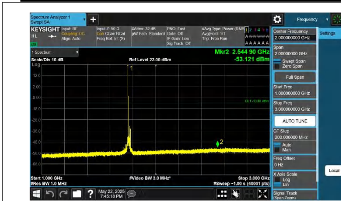
66-66-15MHz-10MHz-QPSK-QPSK-132499-132619-1RB#0-0RB #0-1000~3000MHz-PASS
