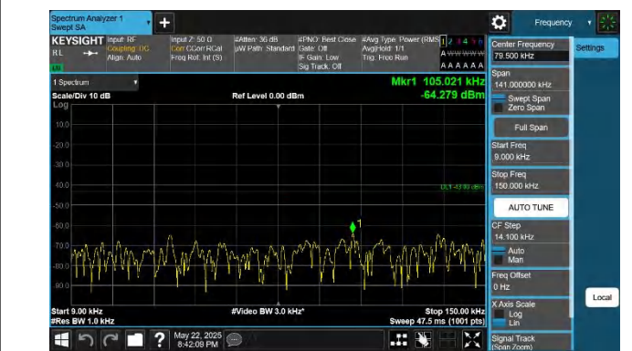
66-66-20MHz-5MHz-QPSK-QPSK-132397-132514-1RB#0-ORB# 0-0.009~0.15MHz-PASS
