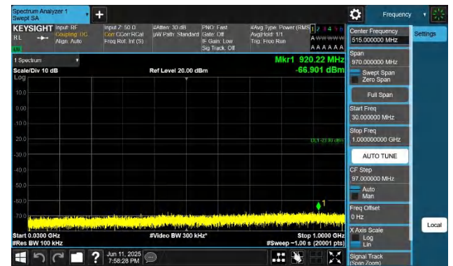
66-66-15MHz-10MHz-QPSK-QPSK-132499-132619-1RB#0-0RB #0-30~1000MHz-PASS
