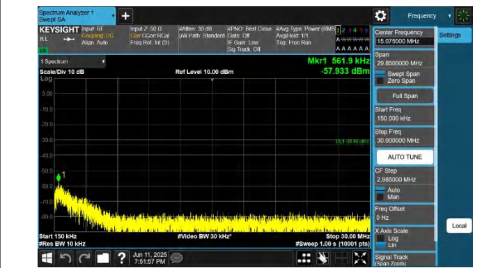
66-66-5MHz-20MHz-QPSK-QPSK-132428-132572-1RB#24-0RB #0-0.15~30MHz-PASS
