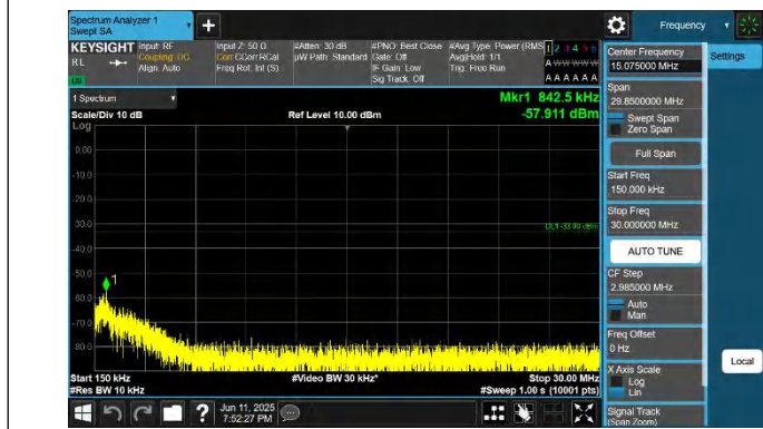
66-66-10MHz-15MHz-QPSK-QPSK-132025-132145-1RB#0-ORB #0-0.15~30MHz-PASS
