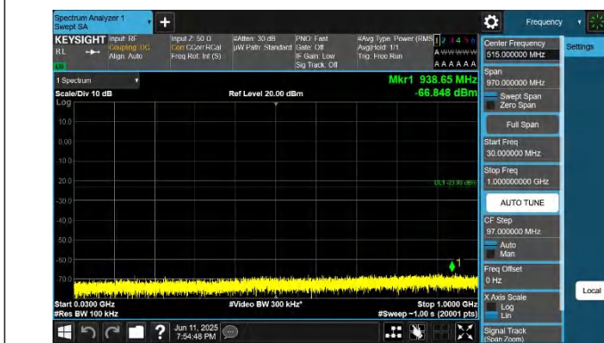
66-66-10MHz-20MHz-QPSK-QPSK-132027-132171-1RB#0-0RB #0-30~1000MHz-PASS
