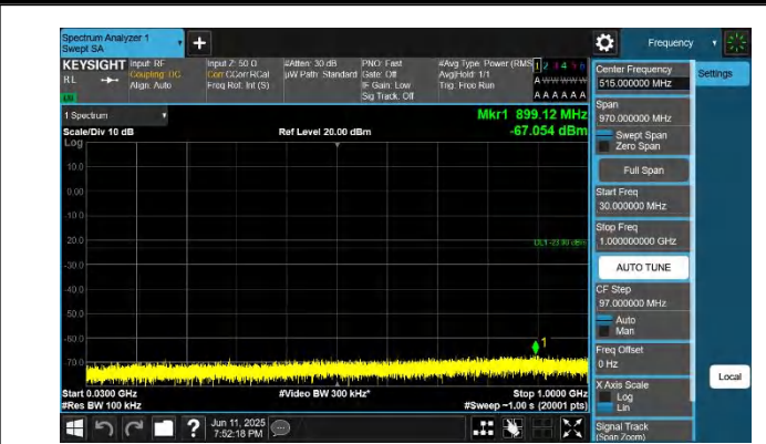
66-66-5MHz-20MHz-QPSK-QPSK-132428-132572-1RB#0-1RB# 99-30~1000MHz-PASS
