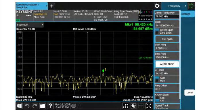
66-66-5MHz-20MHz-QPSK-QPSK-132428-132572-1RB#0-1RB# 99-0.009~0.15MHz-PASS
