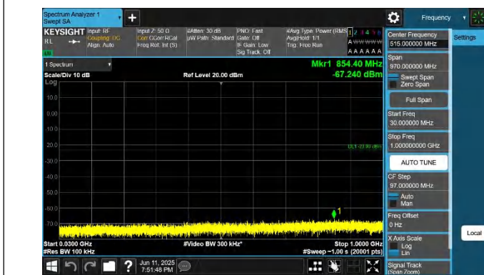
66-66-5MHz-20MHz-QPSK-QPSK-132428-132572-1RB#0-0RB# 0-30~1000MHz-PASS
