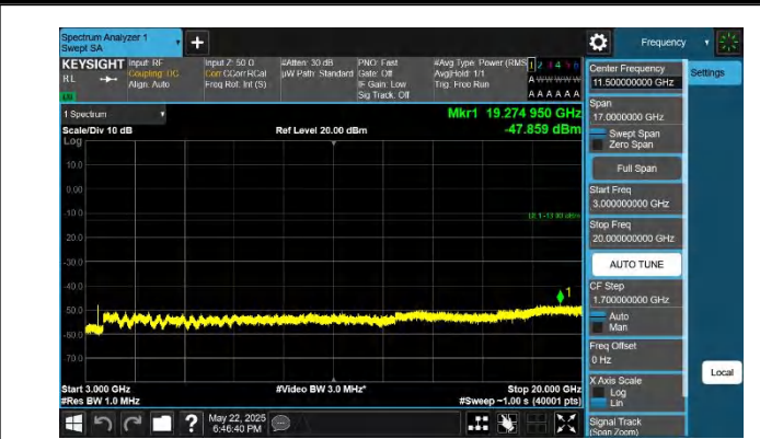
66-66-10MHz-15MHz-QPSK-QPSK-132025-132145-1RB#0-0RB #0-3000~20000MHz-PASS
