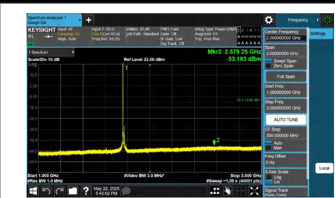
66-66-5MHz-20MHz-QPSK-QPSK-132428-132572-1RB#24-ORB #0-1000~3000MHz-PASS
