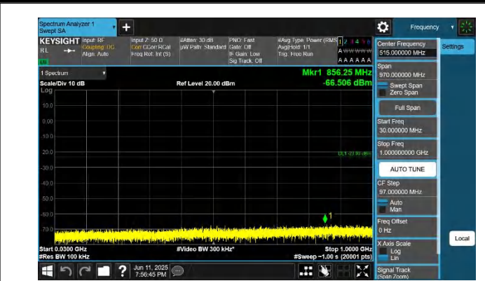
66-66-10MHz-20MHz-QPSK-QPSK-132428-132572-1RB#0-1RB #99-30~1000MHz-PASS
