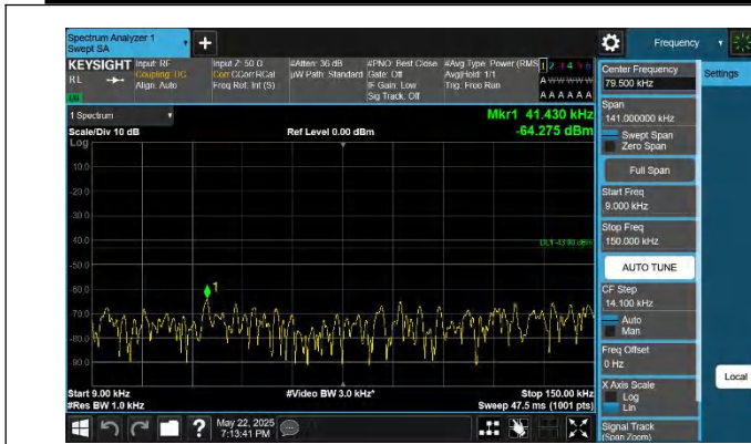
66-66-10MHz-20MHz-QPSK-QPSK-132027-132171-1RB#0-0RB #0-0.009~0.15MHz-PASS
