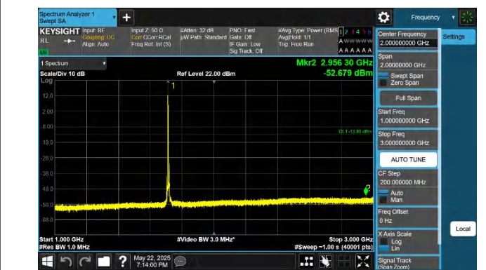
66-66-10MHz-20MHz-QPSK-QPSK-132027-132171-1RB#0-0RB #0-1000~3000MHz-PASS
