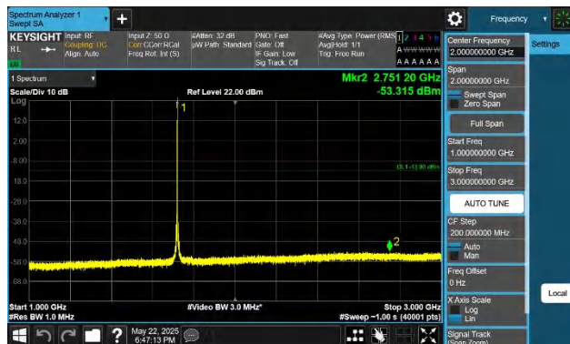
66-66-10MHz-15MHz-QPSK-QPSK-132025-132145-1RB#49-0R B#0-1000~3000MHz-PASS
