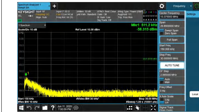
66-66-5MHz-20MHz-QPSK-QPSK-132328-132472-1RB#0-ORB# 0-0.15~30MHz-PASS
