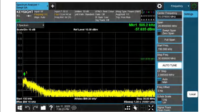
66-66-10MHz-20MHz-QPSK-QPSK-132428-132572-1RB#49-0R B#0-0.15~30MHz-PASS
