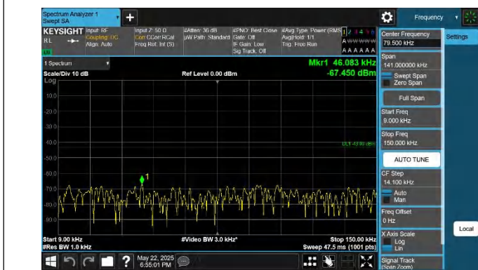
66-66-10MHz-15MHz-QPSK-QPSK-132477-132597-1RB#0-1RB #74-0.009~0.15MHz-PASS
