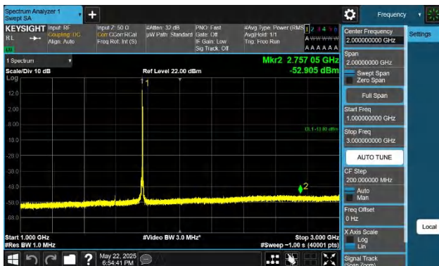
66-66-10MHz-15MHz-QPSK-QPSK-132477-132597-1RB#49-0R B#0-1000~3000MHz-PASS
