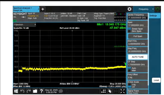
66-66-5MHz-20MHz-QPSK-QPSK-132328-132472-1RB#0-0RB# 0-3000~20000MHz-PASS
