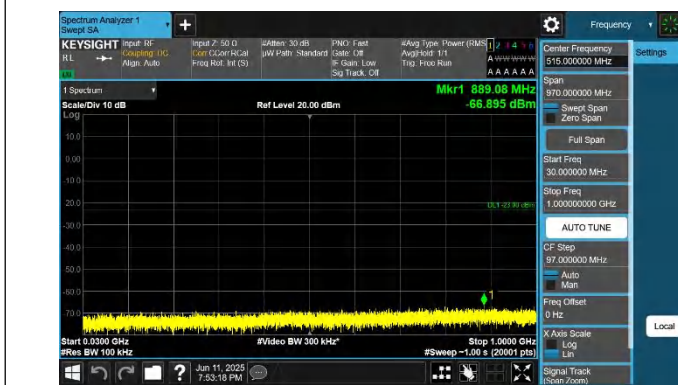
66-66-10MHz-15MHz-QPSK-QPSK-132351-132471-1RB#0-0RB #0-30~1000MHz-PASS
