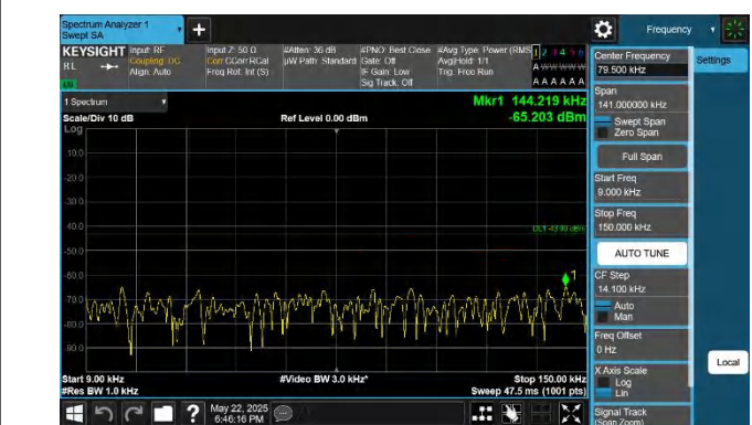
66-66-10MHz-15MHz-QPSK-QPSK-132025-132145-1RB#0-ORB #0-0.009~0.15MHz-PASS
