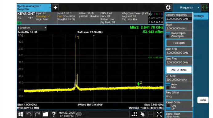
66-66-10MHz-15MHz-QPSK-QPSK-132351-132471-1RB#0-0RB #0-1000~3000MHz-PASS
