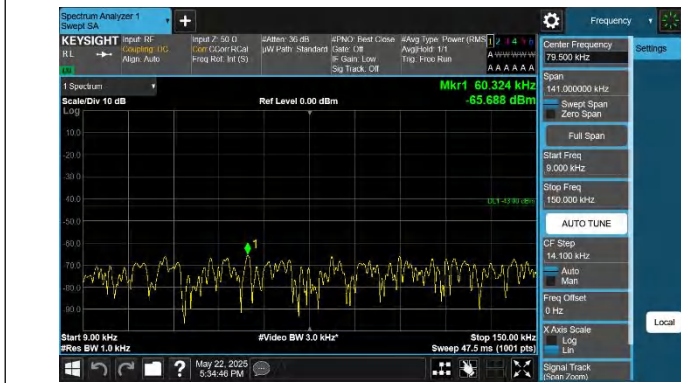
66-66-5MHz-20MHz-QPSK-QPSK-132027-132171-1RB#24-0RB #0-0.009~0.15MHz-PASS
