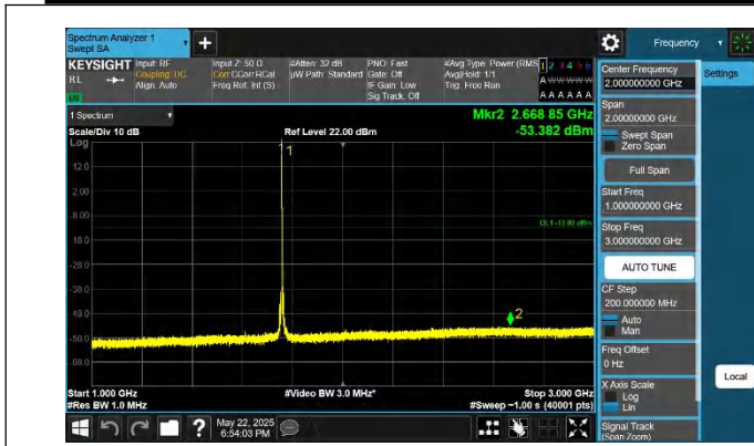
66-66-10MHz-15MHz-QPSK-QPSK-132477-132597-1RB#0-0RB #0-1000~3000MHz-PASS
