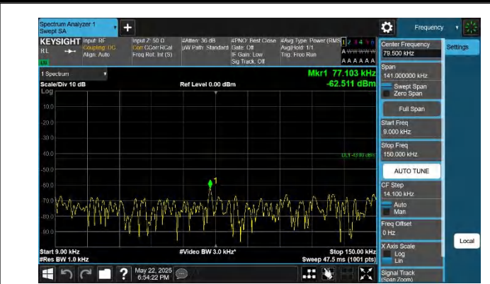
66-66-10MHz-15MHz-QPSK-QPSK-132477-132597-1RB#49-0R B#0-0.009~0.15MHz-PASS
