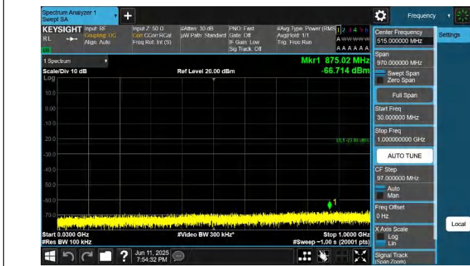
66-66-10MHz-15MHz-QPSK-QPSK-132477-132597-1RB#0-1RB #74-30~1000MHz-PASS
