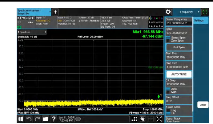
66-66-10MHz-15MHz-QPSK-QPSK-132351-132471-1RB#0-1RB #74-30~1000MHz-PASS
