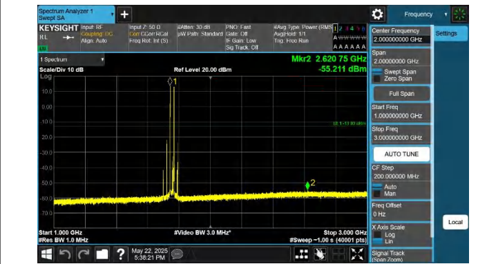
66-66-5MHz-20MHz-QPSK-QPSK-132328-132472-1RB#0-1RB# 99-1000~3000MHz-PASS
