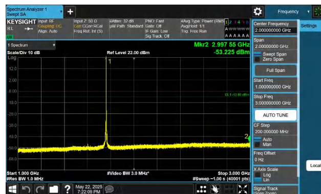
66-66-10MHz-20MHz-QPSK-QPSK-132428-132572-1RB#49-0R B#0-1000~3000MHz-PASS
