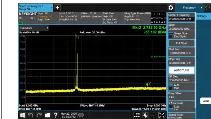
66-66-5MHz-20MHz-QPSK-QPSK-132027-132171-1RB#0-1RB# 99-1000~3000MHz-PASS
