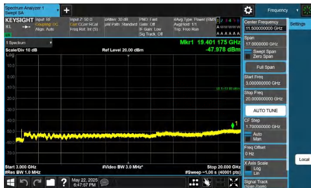
66-66-10MHz-15MHz-QPSK-QPSK-132025-132145-1RB#0-1RB #74-3000~20000MHz-PASS
