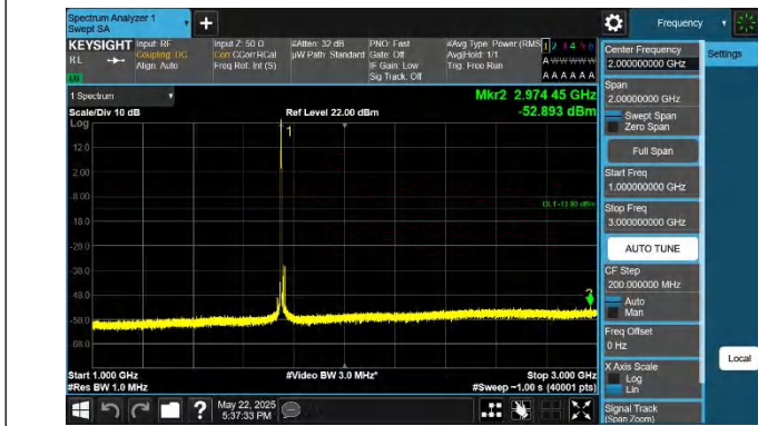
66-66-5MHz-20MHz-QPSK-QPSK-132328-132472-1RB#24-0RB #0-1000~3000MHz-PASS
