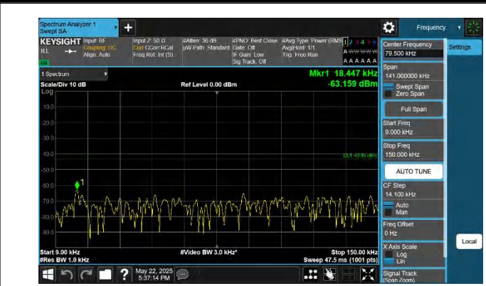
66-66-5MHz-20MHz-QPSK-QPSK-132328-132472-1RB#24-0RB #0-0.009~0.15MHz-PASS
