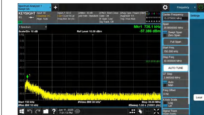
66-66-5MHz-20MHz-QPSK-QPSK-132328-132472-1RB#24-0RB #0-0.15~30MHz-PASS
