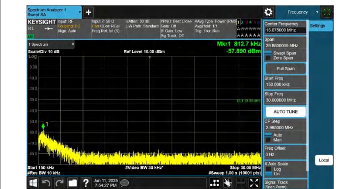
66-66-10MHz-15MHz-QPSK-QPSK-132477-132597-1RB#0-1RB #74-0.15~30MHz-PASS
