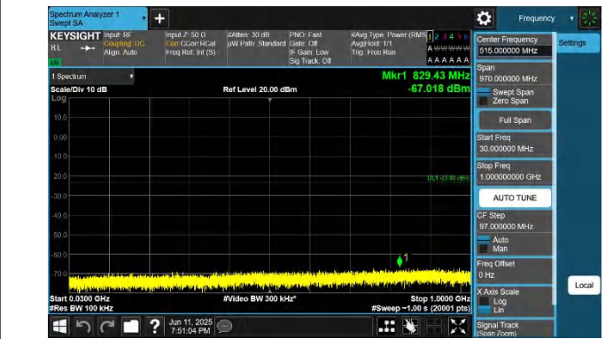
66-66-5MHz-20MHz-QPSK-QPSK-132328-132472-1RB#0-ORB# 0-30~1000MHz-PASS
