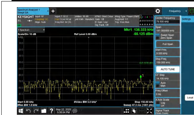
66-66-5MHz-20MHz-QPSK-QPSK-132428-132572-1RB#0-0RB# 0-0.009~0.15MHz-PASS
