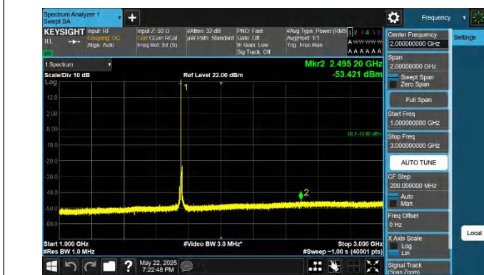
66-66-10MHz-20MHz-QPSK-QPSK-132428-132572-1RB#0-1RB #99-1000~3000MHz-PASS
