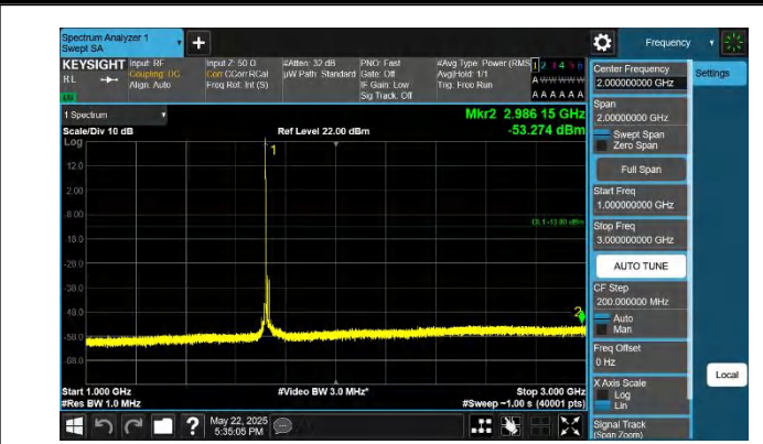
66-66-5MHz-20MHz-QPSK-QPSK-132027-132171-1RB#24-ORB #0-1000~3000MHz-PASS
