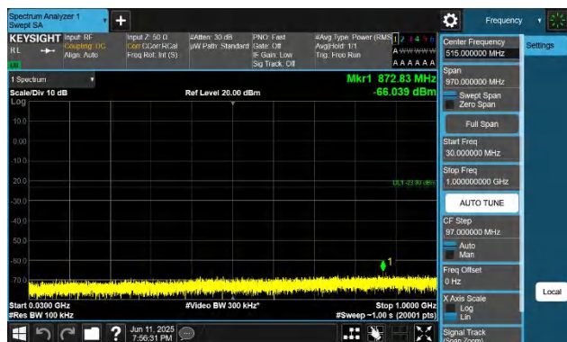
66-66-10MHz-20MHz-QPSK-QPSK-132428-132572-1RB#49-0R B#0-30~1000MHz-PASS
