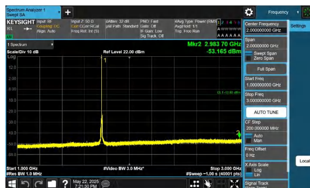
66-66-10MHz-20MHz-QPSK-QPSK-132428-132572-1RB#0-0RB #0-1000~3000MHz-PASS
