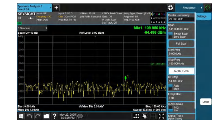
66-66-5MHz-20MHz-QPSK-QPSK-132328-132472-1RB#0-ORB# 0-0.009~0.15MHz-PASS
