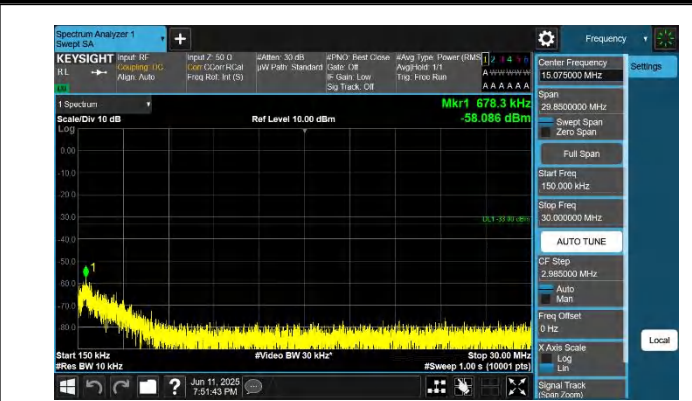
66-66-5MHz-20MHz-QPSK-QPSK-132428-132572-1RB#0-0RB# 0-0.15~30MHz-PASS
