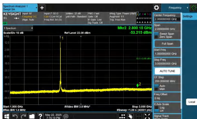
66-66-10MHz-20MHz-QPSK-QPSK-132027-132171-1RB#0-1RB #99-1000~3000MHz-PASS
