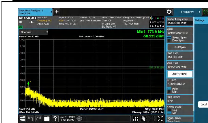
66-66-10MHz-20MHz-QPSK-QPSK-132428-132572-1RB#0-1RB #99-0.15~30MHz-PASS
