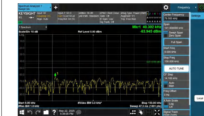
66-66-5MHz-20MHz-QPSK-QPSK-132328-132472-1RB#0-1RB# 99-0.009~0.15MHz-PASS
