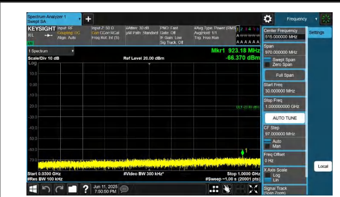
66-66-5MHz-20MHz-QPSK-QPSK-132027-132171-1RB#0-1RB# 99-30~1000MHz-PASS
