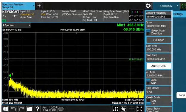
66-66-10MHz-15MHz-QPSK-QPSK-132477-132597-1RB#49-0R B#0-0.15~30MHz-PASS
