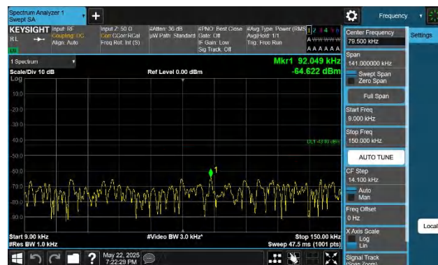
66-66-10MHz-20MHz-QPSK-QPSK-132428-132572-1RB#0-1RB #99-0.009~0.15MHz-PASS
