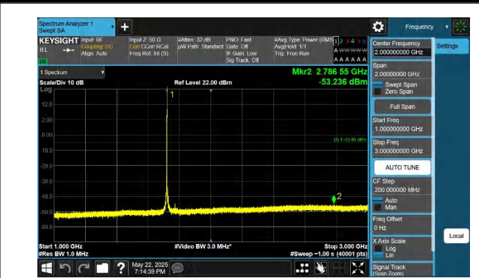
66-66-10MHz-20MHz-QPSK-QPSK-132027-132171-1RB#49-0R B#0-1000~3000MHz-PASS
