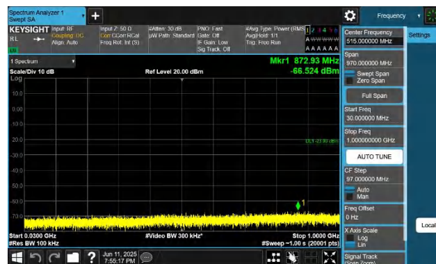
66-66-10MHz-20MHz-QPSK-QPSK-132027-132171-1RB#0-1RB #99-30~1000MHz-PASS
