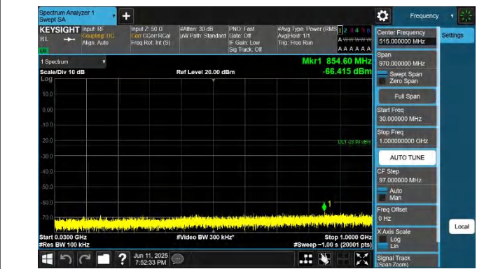
66-66-10MHz-15MHz-QPSK-QPSK-132025-132145-1RB#0-ORB #0-30~1000MHz-PASS
