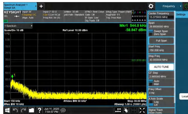
66-66-10MHz-20MHz-QPSK-QPSK-132027-132171-1RB#49-0R B#0-0.15~30MHz-PASS
