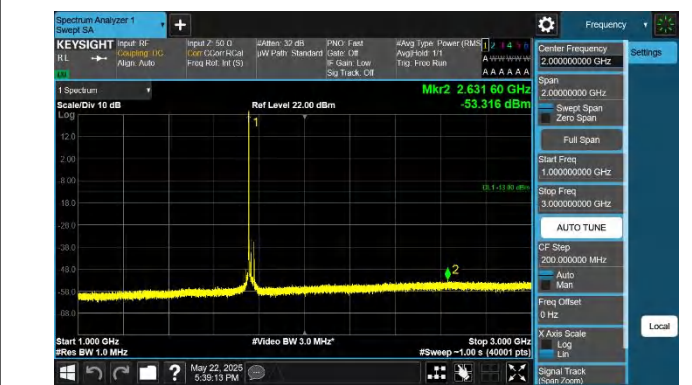
66-66-5MHz-20MHz-QPSK-QPSK-132428-132572-1RB#0-0RB# 0-1000~3000MHz-PASS
