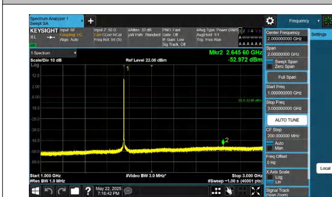
66-66-10MHz-20MHz-QPSK-QPSK-132328-132472-1RB#49-0R B#0-1000~3000MHz-PASS
