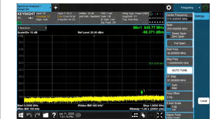
66-66-5MHz-20MHz-QPSK-QPSK-132328-132472-1RB#24-0RB #0-30~1000MHz-PASS
