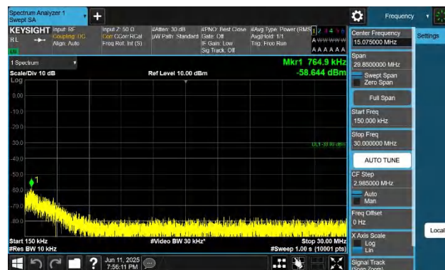
66-66-10MHz-20MHz-QPSK-QPSK-132428-132572-1RB#0-0RB #0-0.15~30MHz-PASS
