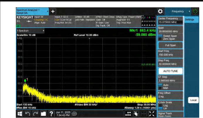
66-66-10MHz-20MHz-QPSK-QPSK-132027-132171-1RB#0-0RB #0-0.15~30MHz-PASS
