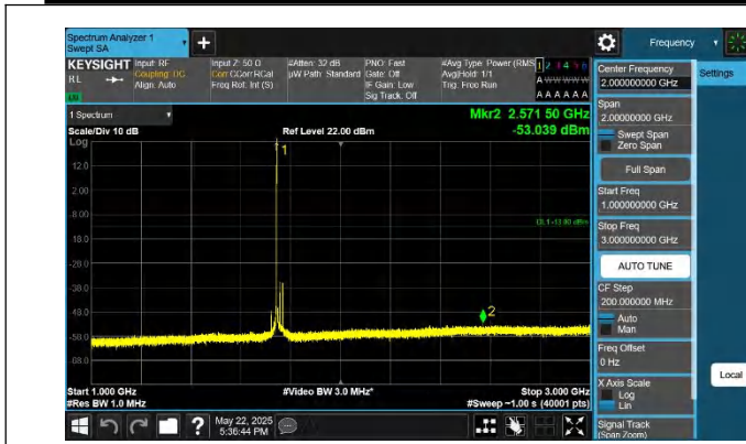
66-66-5MHz-20MHz-QPSK-QPSK-132328-132472-1RB#0-0RB# 0-1000~3000MHz-PASS
