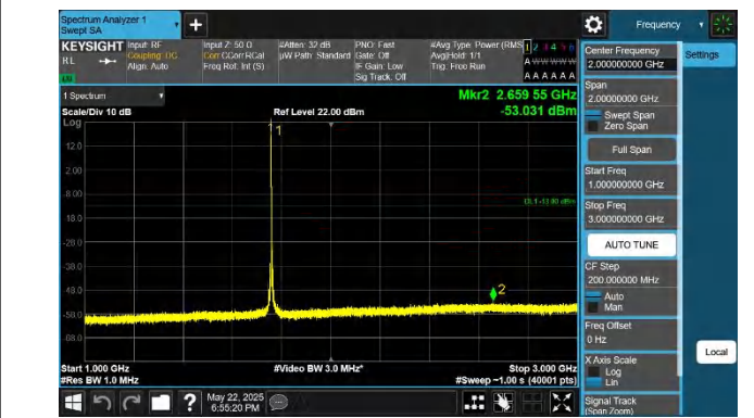
66-66-10MHz-15MHz-QPSK-QPSK-132477-132597-1RB#0-1RB #74-1000~3000MHz-PASS
