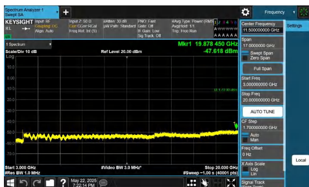
66-66-10MHz-20MHz-QPSK-QPSK-132428-132572-1RB#49-0R B#0-3000~20000MHz-PASS
