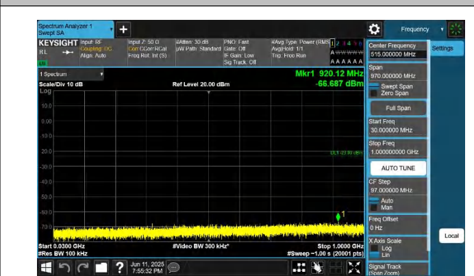
66-66-10MHz-20MHz-QPSK-QPSK-132328-132472-1RB#0-0RB #0-30~1000MHz-PASS
