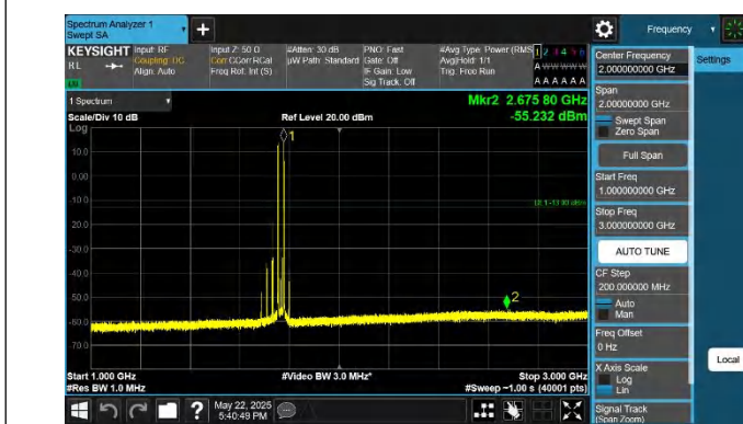
66-66-5MHz-20MHz-QPSK-QPSK-132428-132572-1RB#0-1RB# 99-1000~3000MHz-PASS
