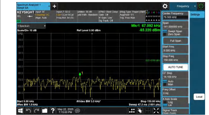
66-66-10MHz-20MHz-QPSK-QPSK-132027-132171-1RB#0-1RB #99-0.009~0.15MHz-PASS
