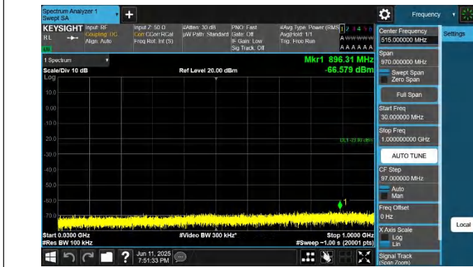
66-66-5MHz-20MHz-QPSK-QPSK-132328-132472-1RB#0-1RB# 99-30~1000MHz-PASS
