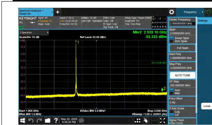
66-66-10MHz-15MHz-QPSK-QPSK-132025-132145-1RB#0-0RB #0-1000~3000MHz-PASS
