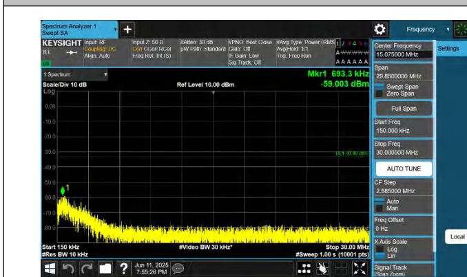
66-66-10MHz-20MHz-QPSK-QPSK-132328-132472-1RB#0-0RB #0-0.15~30MHz-PASS
