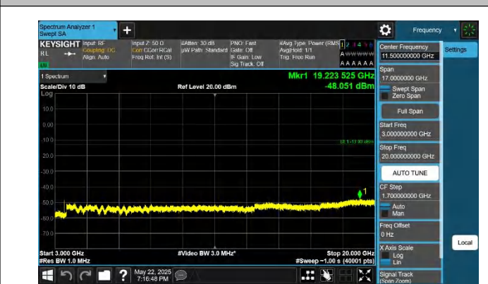
66-66-10MHz-20MHz-QPSK-QPSK-132328-132472-1RB#49-0R B#0-3000~20000MHz-PASS
