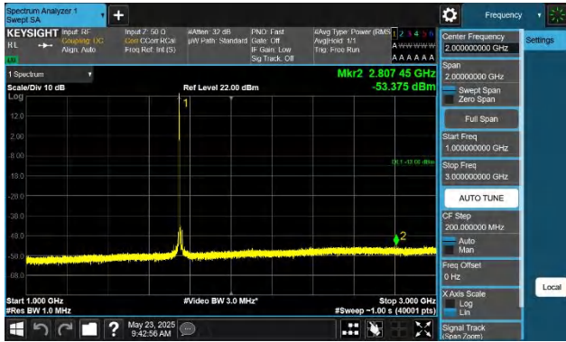
66-66-15MHz-5MHz-QPSK-QPSK-132398-132491-1RB#0-0RB# 0-1000~3000MHz-PASS
