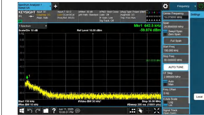
66-66-15MHz-5MHz-QPSK-QPSK-132398-132491-1RB#0-ORB# 0-0.15~30MHz-PASS
