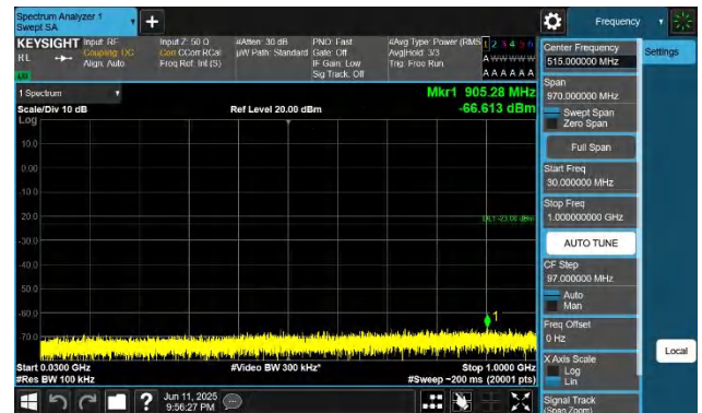
66-66-10MHz-10MHz-QPSK-QPSK-132523-132622-1RB#49-0R B#0-30~1000MHz-PASS
