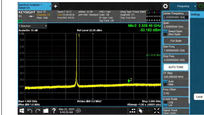
66-66-15MHz-5MHz-QPSK-QPSK-132398-132491-1RB#74-ORB #0-1000~3000MHz-PASS
