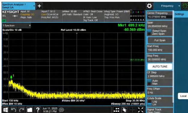
66-66-10MHz-10MHz-QPSK-QPSK-132523-132622-1RB#49-0R B#0-0.15~30MHz-PASS
