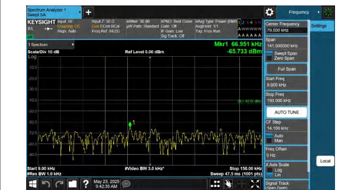
66-66-15MHz-5MHz-QPSK-QPSK-132398-132491-1RB#0-ORB# 0-0.009~0.15MHz-PASS
