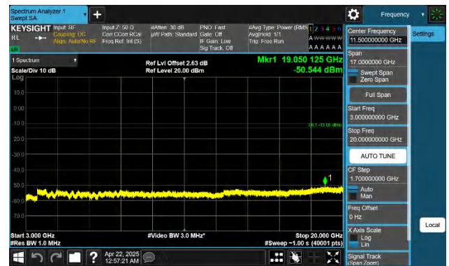
66-66-10MHz-10MHz-QPSK-QPSK-132523-132622-1RB#49-0R B#0-3000~20000MHz-PASS
