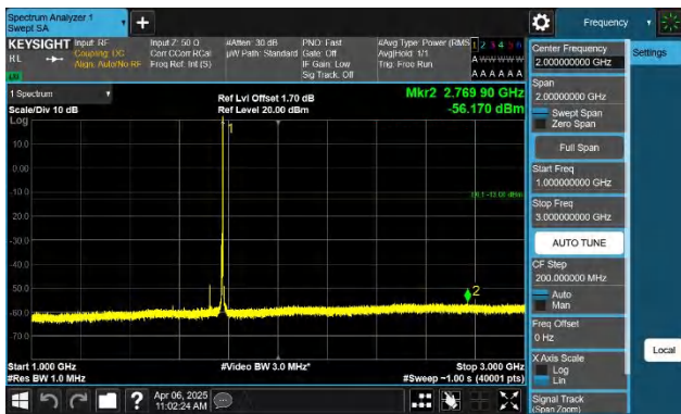
66-66-10MHz-10MHz-QPSK-QPSK-132523-132622-1RB#49-0R B#0-1000~3000MHz-PASS
