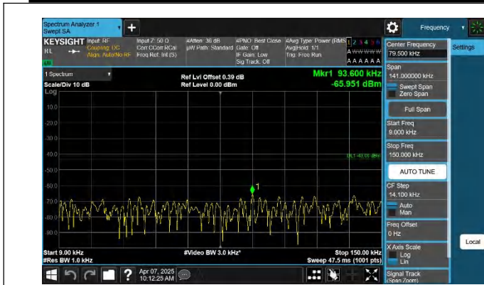
66-66-10MHz-5MHz-QPSK-QPSK-132022-132094-1RB#0-0RB# 0-0.009~0.15MHz-PASS
