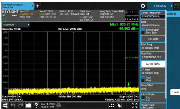
66-66-10MHz-10MHz-QPSK-QPSK-132022-132121-1RB#0-1RB #49-30~1000MHz-PASS
