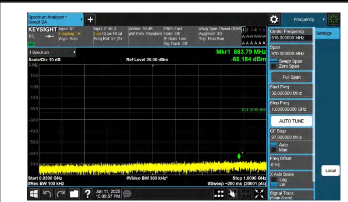
42-42-20MHz-20MHz-QPSK-QPSK-42491-42689-1RB#99-0RB# 0-30~1000MHz-PASS
