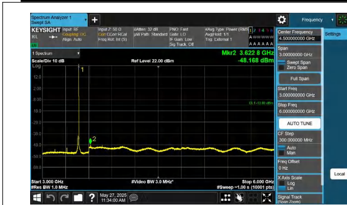
42-42-20MHz-20MHz-QPSK-QPSK-42190-42388-1RB#99-0RB# 0-3000~6000MHz-PASS
