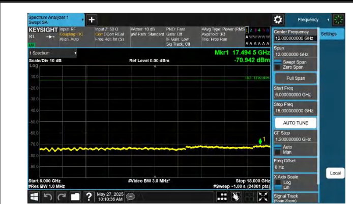
42-42-20MHz-20MHz-QPSK-QPSK-42190-42388-1RB#99-0RB# 0-6000~18000MHz-PASS
