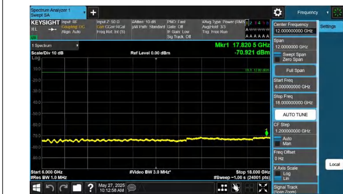
42-42-20MHz-20MHz-QPSK-QPSK-42491-42689-1RB#0-0RB#0- 6000~18000MHz-PASS
