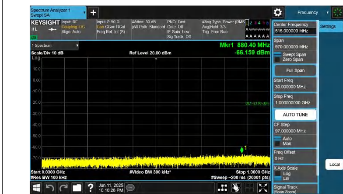
42-42-20MHz-20MHz-QPSK-QPSK-42792-42990-1RB#0-0RB#0- 30~1000MHz-PASS
