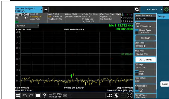
42-42-20MHz-20MHz-QPSK-QPSK-42792-42990-1RB#0-0RB#0- 0.009~0.15MHz-PASS
