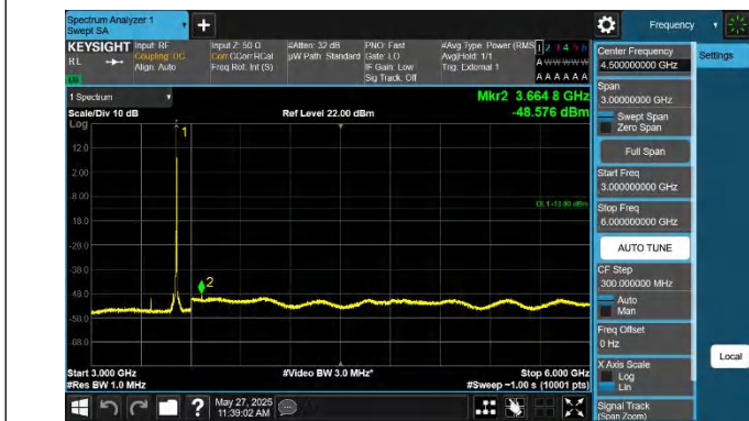
42-42-20MHz-20MHz-QPSK-QPSK-42792-42990-1RB#0-0RB#0- 3000~6000MHz-PASS
