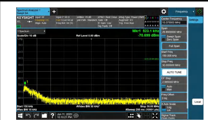
42-42-20MHz-20MHz-QPSK-QPSK-42792-42990-1RB#0-0RB#0- 0.15~30MHz-PASS
