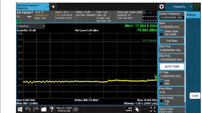
42-42-15MHz-20MHz-QPSK-QPSK-42168-42339-1RB#0-0RB#0- 6000~18000MHz-PASS
