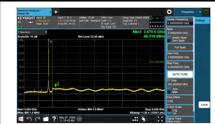
42-42-10MHz-20MHz-QPSK-QPSK-42846-42990-1RB#0-0RB#0-3000~6000MHz-PASS
