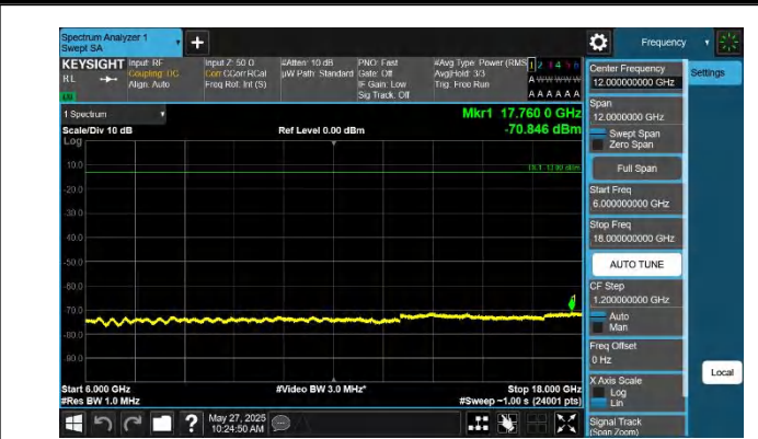
42-42-20MHz-5MHz-QPSK-QPSK-42565-42682-1RB#99-0RB#0- 6000~18000MHz-PASS
