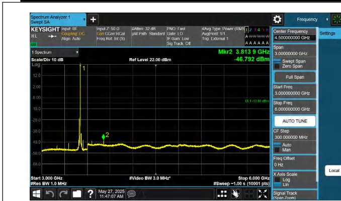
42-42-20MHz-5MHz-QPSK-QPSK-42565-42682-1RB#99-0RB#0- 3000~6000MHz-PASS
