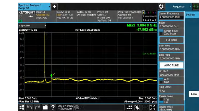
42-42-15MHz-20MHz-QPSK-QPSK-42168-42339-1RB#0-0RB#0- 3000~6000MHz-PASS
