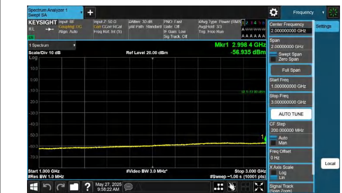
42-42-15MHz-20MHz-QPSK-QPSK-42168-42339-1RB#0-0RB#0- 1000~3000MHz-PASS
