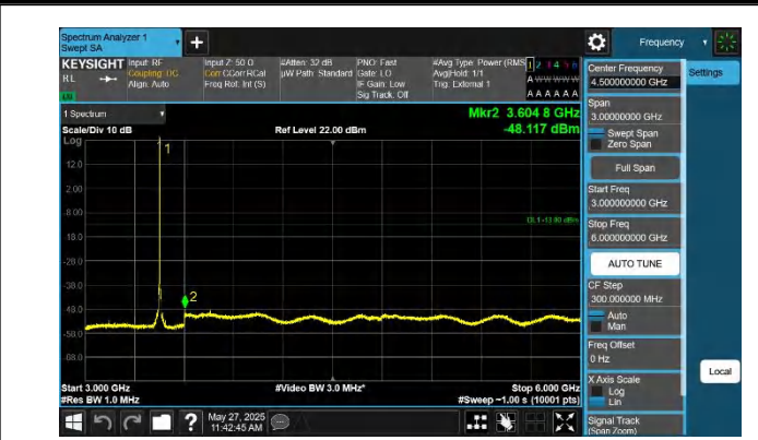
42-42-20MHz-5MHz-QPSK-QPSK-42190-42307-1RB#0-0RB#0-3 000~6000MHz-PASS
