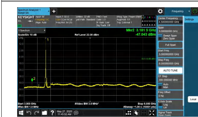
42-42-20MHz-5MHz-QPSK-QPSK-42565-42682-1RB#0-0RB#0-3 000~6000MHz-PASS
