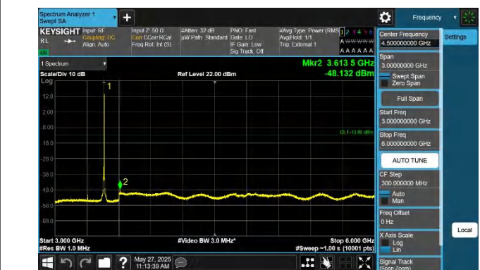
42-42-10MHz-20MHz-QPSK-QPSK-42145-42289-1RB#49-0RB# 0-3000~6000MHz-PASS
