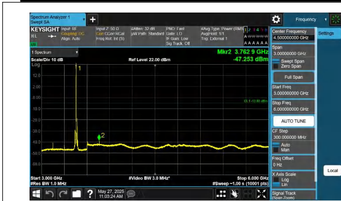
42-42-5MHz-20MHz-QPSK-QPSK-42123-42240-1RB#24-0RB#0- 3000~6000MHz-PASS
