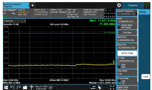
42-42-5MHz-20MHz-QPSK-QPSK-42498-42615-1RB#0-1RB#99- 6000~18000MHz-PASS
