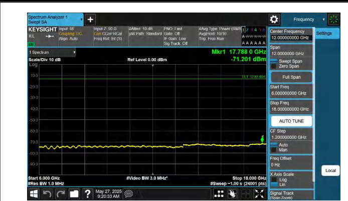
42-42-5MHz-20MHz-QPSK-QPSK-42123-42240-1RB#24-0RB#0- 6000~18000MHz-PASS
