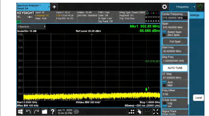
42-42-10MHz-20MHz-QPSK-QPSK-42145-42289-1RB#0-0RB#0- 30~1000MHz-PASS
