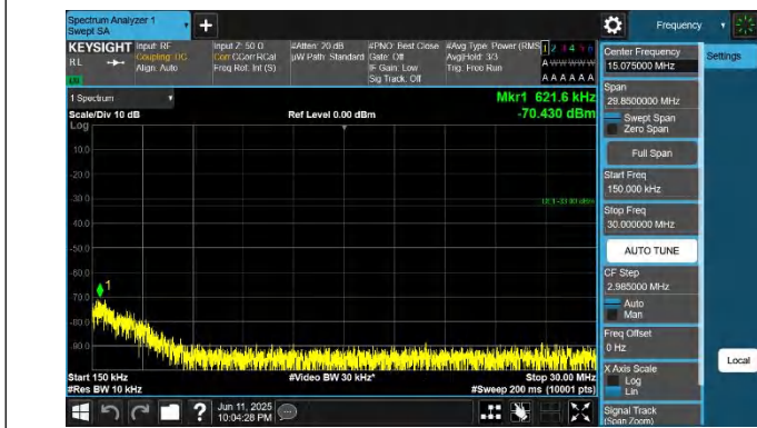
42-42-10MHz-20MHz-QPSK-QPSK-42145-42289-1RB#0-0RB#0- 0.15~30MHz-PASS
