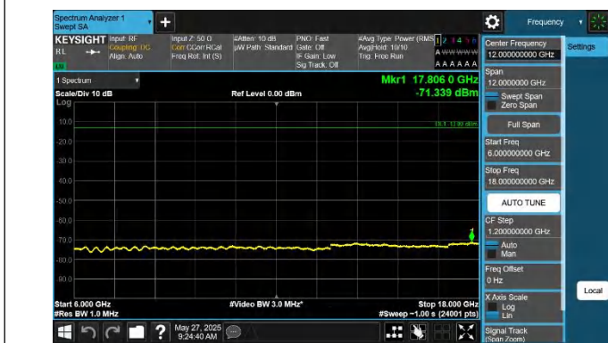
42-42-5MHz-20MHz-QPSK-QPSK-42498-42615-1RB#0-0RB#0-6 000~18000MHz-PASS
