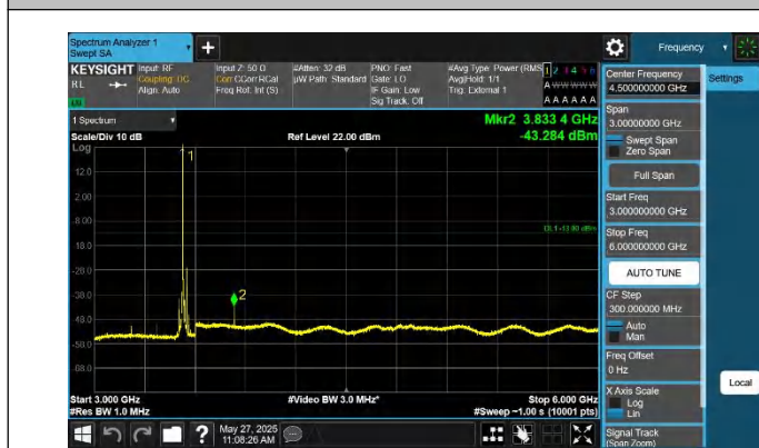
42-42-5MHz-20MHz-QPSK-QPSK-42873-42990-1RB#0-0RB#0-3 000~6000MHz-PASS
