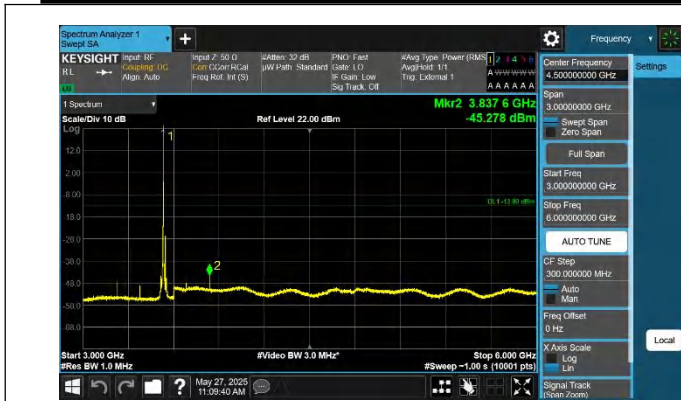
42-42-5MHz-20MHz-QPSK-QPSK-42873-42990-1RB#24-0RB#0- 3000~6000MHz-PASS
