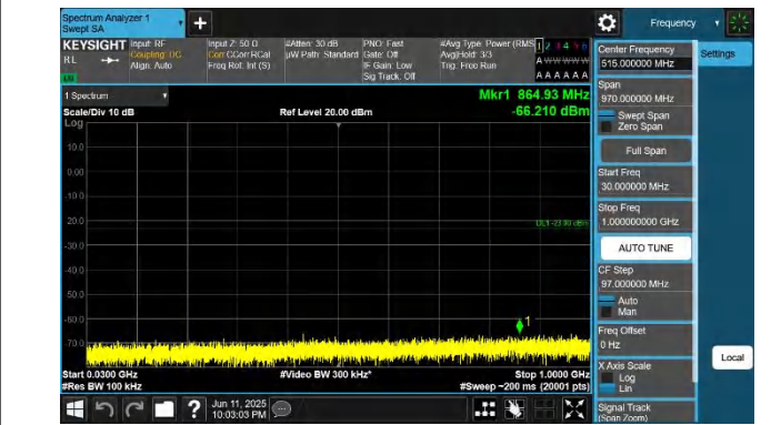
42-42-5MHz-20MHz-QPSK-QPSK-42498-42615-1RB#0-0RB#0-3 0~1000MHz-PASS
