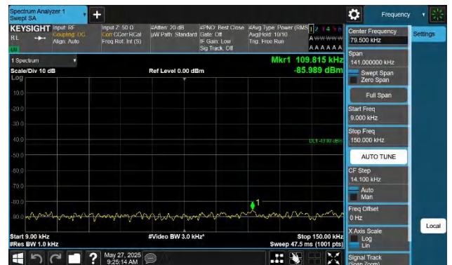
42-42-5MHz-20MHz-QPSK-QPSK-42498-42615-1RB#24-0RB#0- 0.009~0.15MHz-PASS
