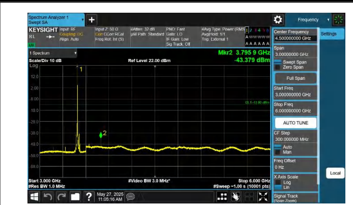
42-42-5MHz-20MHz-QPSK-QPSK-42498-42615-1RB#0-0RB#0-3 000~6000MHz-PASS
