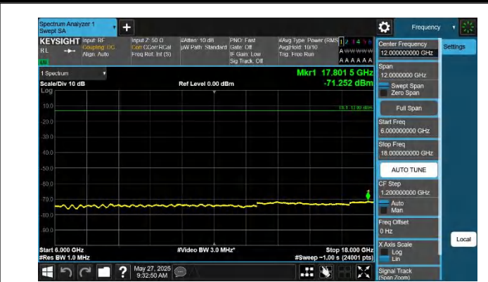
42-42-5MHz-20MHz-QPSK-QPSK-42873-42990-1RB#24-0RB#0- 6000~18000MHz-PASS
