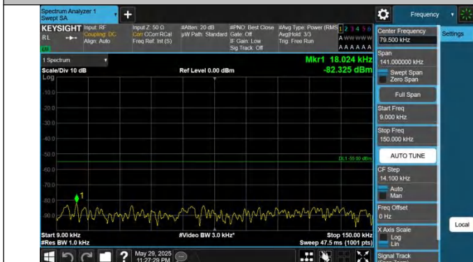
41-41-20MHz-20MHz-QPSK-QPSK-39750-39948-1RB#99-0RB# 0-0.009~0.15MHz-PASS
