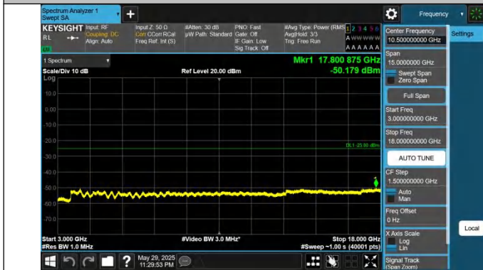
41-41-20MHz-20MHz-QPSK-QPSK-40521-40719-1RB#99-0RB# 0-3000~18000MHz-PASS
