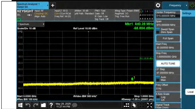
41-41-20MHz-20MHz-QPSK-QPSK-39750-39948-1RB#99-0RB# 0-30~1000MHz-PASS
