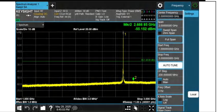
41-41-20MHz-20MHz-QPSK-QPSK-39750-39948-1RB#99-0RB#0 -1000~3000MHz-PASS
