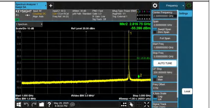
41-1-20MHz-10MHz-QPSK-QPSK-41391-41535-1RB#0-0RB#0- 1000~3000MHz-PASS
