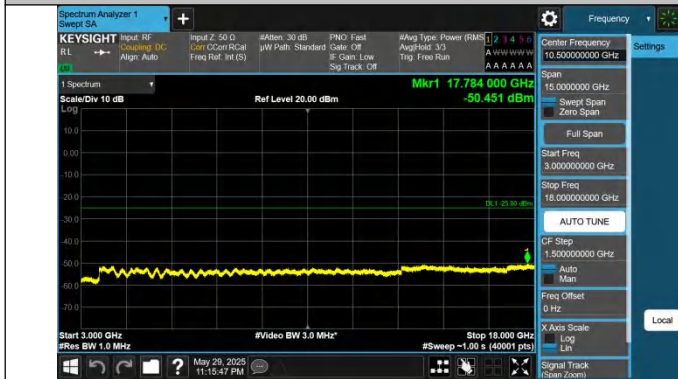
41-41-20MHz-10MHz-QPSK-QPSK-39750-39894-1RB#99-0RB# 0-3000~18000MHz-PASS
