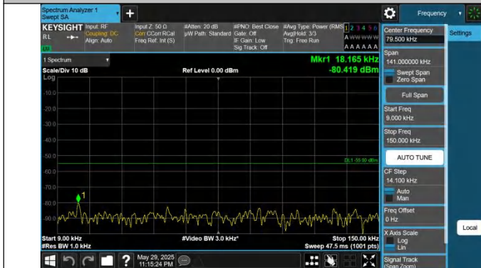
41-41-20MHz-10MHz-QPSK-QPSK-39750-39894-1RB#99-0RB# 0-0.009~0.15MHz-PASS
