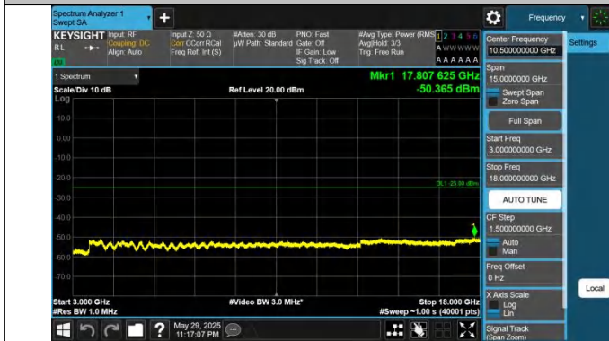
41-41-20MHz-10MHz-QPSK-QPSK-40571-40715-1RB#0-0RB#0- 3000~18000MHz-PASS
