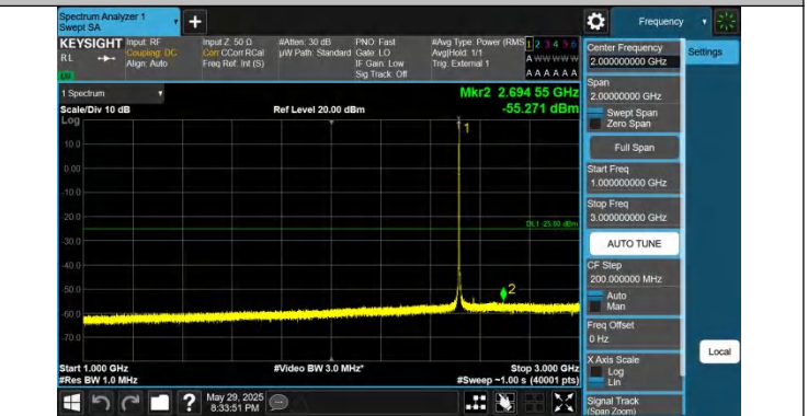
41-41-20MHz-10MHz-QPSK-QPSK-39750-39894-1RB#99-0RB#0 -1000~3000MHz-PASS
