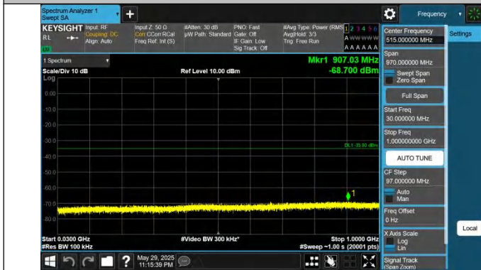
41-41-20MHz-10MHz-QPSK-QPSK-39750-39894-1RB#99-0RB# 0-30~1000MHz-PASS
