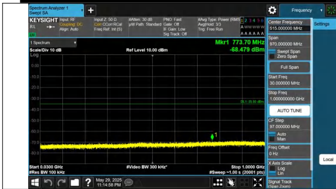
41-41-20MHz-10MHz-QPSK-QPSK-39750-39894-1RB#0-0RB#0-30~1000MHz-PASS
