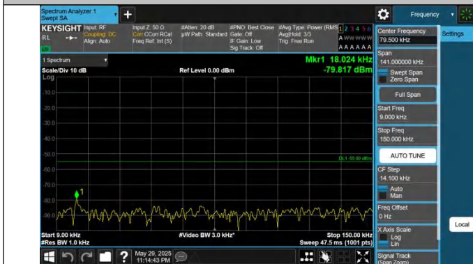
41-41-20MHz-10MHz-QPSK-QPSK-39750-39894-1RB#0-0RB#0-0.009~0.15MHz-PASS
