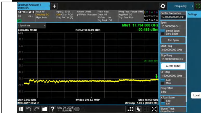
41-1-20MHz-10MHz-QPSK-QPSK-40571-40715-1RB#99-0RB# 0-3000~18000MHz-PASS
