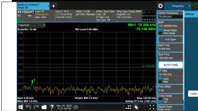
41-41-20MHz-15MHz-QPSK-QPSK-39750-39921-1RB#99-0RB# 0-0.009~0.15MHz-PASS
