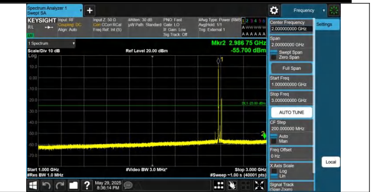
41-41-20MHz-10MHz-QPSK-QPSK-40571-40715-1RB#0-1RB#49 -1000~3000MHz-PASS
