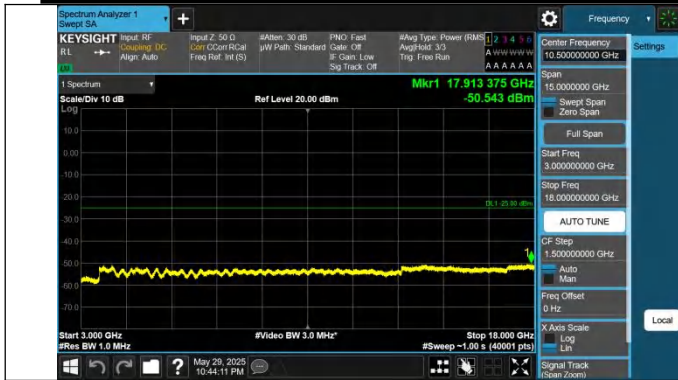
41-41-10MHz-20MHz-QPSK-QPSK-39705-39849-1RB#0-1RB#9 9-3000~18000MHz-PASS
