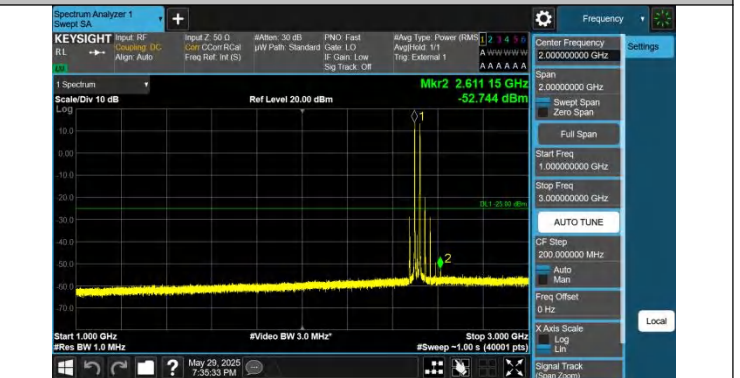
41-41-5MHz-20MHz-QPSK-QPSK-39683-39800-1RB#0-1RB#99- 1000~3000MHz-PASS
