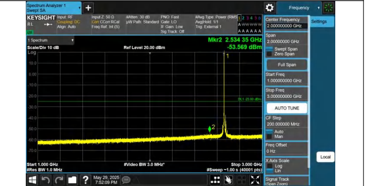
41-41-10MHz-20MHz-QPSK-QPSK-41346-41490-1RB#0-0RB#0- 1000~3000MHz-PASS
