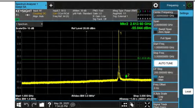
41-41-5MHz-20MHz-QPSK-QPSK-39683-39800-1RB#0-0RB#0-1000~3000MHz-PASS
