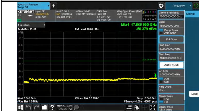
41-41-5MHz-20MHz-QPSK-QPSK-40528-40645-1RB#24-0RB#0- 3000~18000MHz-PASS
