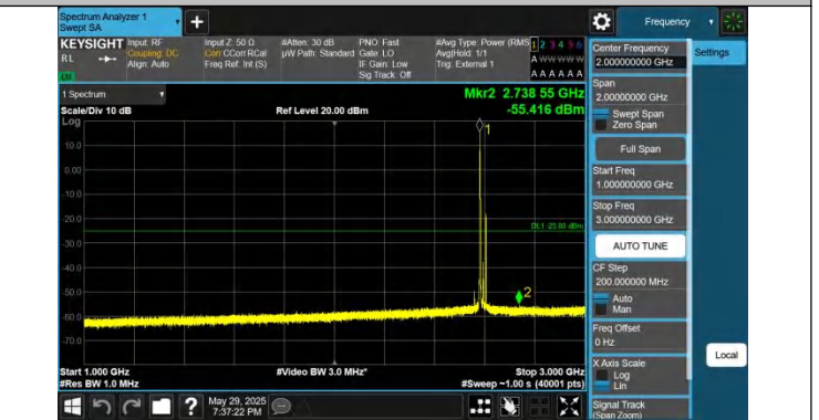
41-41-5MHz-20MHz-QPSK-QPSK-40528-40645-1RB#0-1RB#99- 1000~3000MHz-PASS
