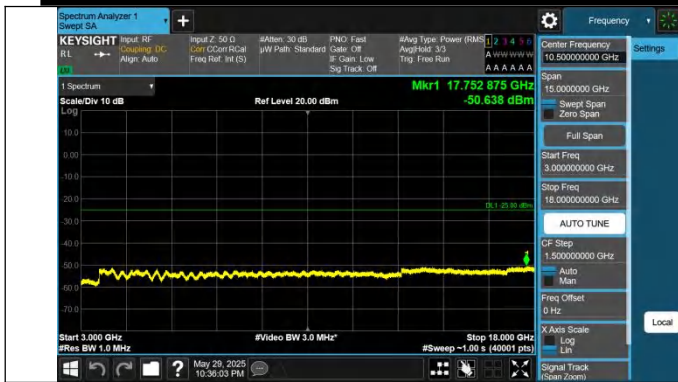
41-41-5MHz-20MHz-QPSK-QPSK-41373-41490-1RB#0-1RB#99- 3000~18000MHz-PASS
