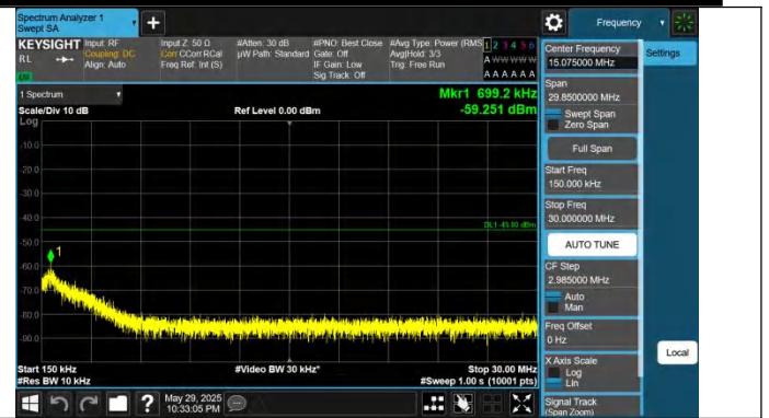
41-41-5MHz-20MHz-QPSK-QPSK-40528-40645-1RB#24-0RB#0- 0.15~30MHz-PASS
