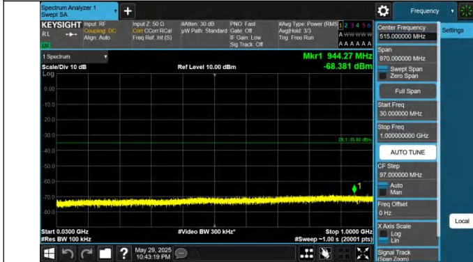
41-41-10MHz-20MHz-QPSK-QPSK-39705-39849-1RB#49-0RB# 0-30~1000MHz-PASS
