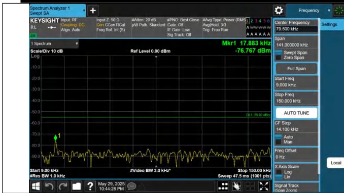
41-41-10MHz-20MHz-QPSK-QPSK-40526-40670-1RB#0-0RB#0-0.009~0.15MHz-PASS
