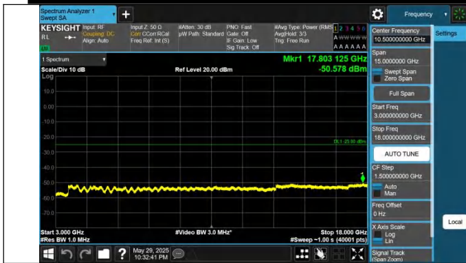
41-41-5MHz-20MHz-QPSK-QPSK-40528-40645-1RB#0-0RB#0-3 000~18000MHz-PASS
