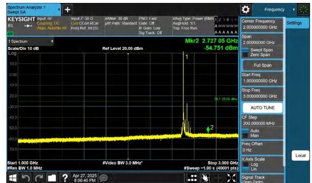
7-7-20MHz-20MHz-QPSK-QPSK-20850-21048-1RB#0-0RB#0-10 00~3000MHz-PASS
