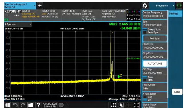
7-7-20MHz-10MHz-QPSK-QPSK-21251-21395-1RB#0-0RB#0-10 00~3000MHz-PASS
