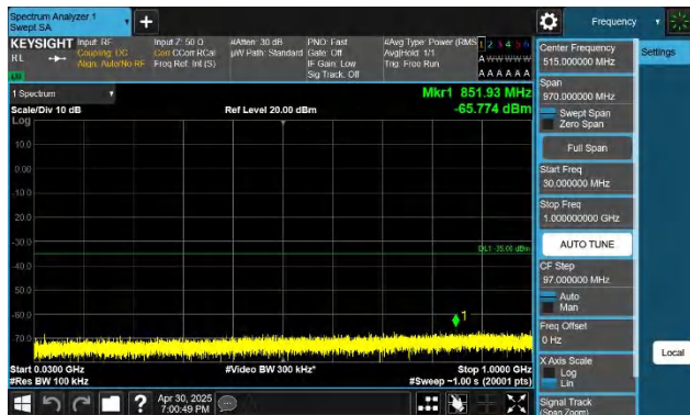
7-7-20MHz-15MHz-QPSK-QPSK-21201-21372-1RB#0-0RB#0-3 0~1000MHz-PASS
