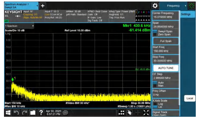
7-7-20MHz-10MHz-QPSK-QPSK-21251-21395-1RB#99-0RB#0-0. 15~30MHz-PASS
