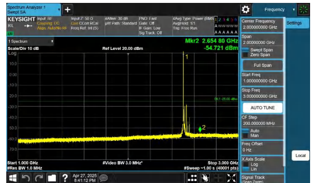
7-7-20MHz-10MHz-QPSK-QPSK-20850-20994-1RB#0-0RB#0-10 00~3000MHz-PASS
