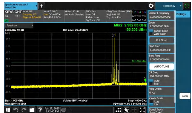
7-7-20MHz-10MHz-QPSK-QPSK-20850-20994-1RB#0-1RB#49-1 000~3000MHz-PASS
