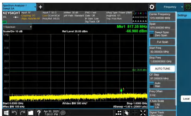
7-7-20MHz-15MHz-QPSK-QPSK-21026-21197-1RB#99-ORB#0-3 0~1000MHz-PASS
