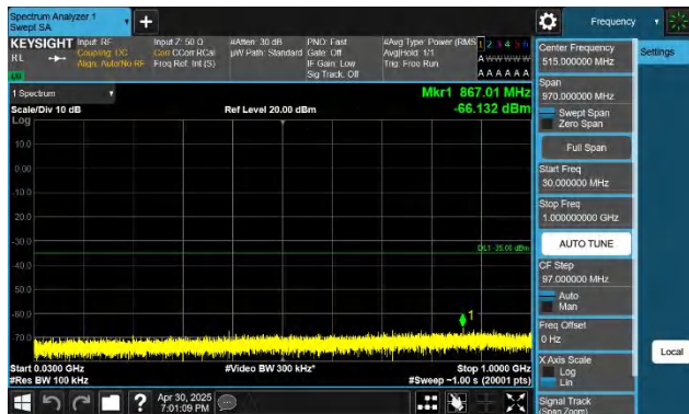
7-7-20MHz-15MHz-QPSK-QPSK-21201-21372-1RB#99-0RB#0-30~1000MHz-PASS
