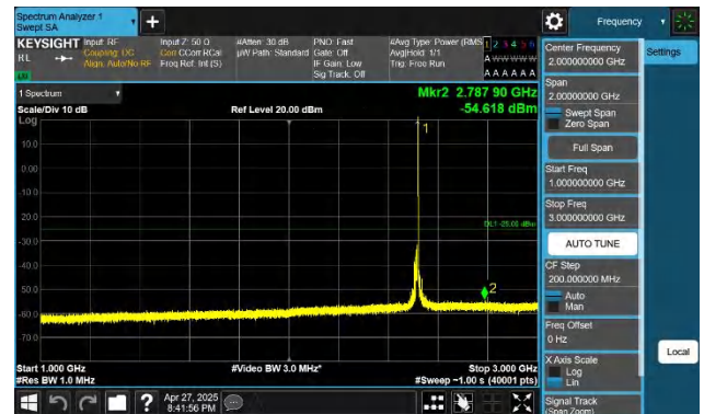
7-7-20MHz-10MHz-QPSK-QPSK-20850-20994-1RB#99-ORB#0-1.000~3000MHz-PASS
