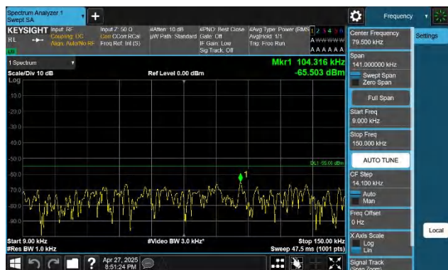
7-7-20MHz-15MHz-QPSK-QPSK-21026-21197-1RB#0-0RB#0-0. 009~0.15MHz-PASS
