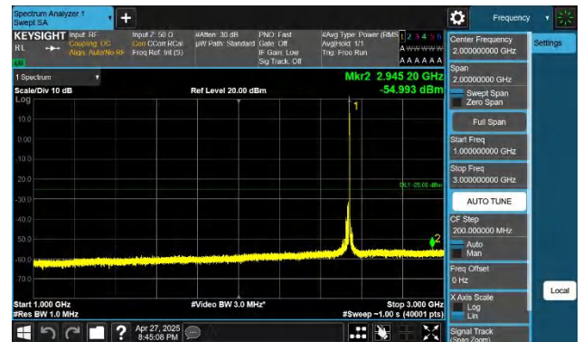
7-7-20MHz-10MHz-QPSK-QPSK-21051-21195-1RB#99-ORB#0-1 000~3000MHz-PASS
