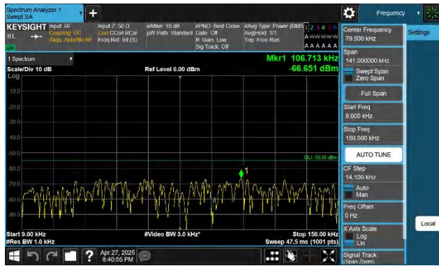
7-7-20MHz-10MHz-QPSK-QPSK-20850-20994-1RB#0-0RB#0-0. 009~0.15MHz-PASS
