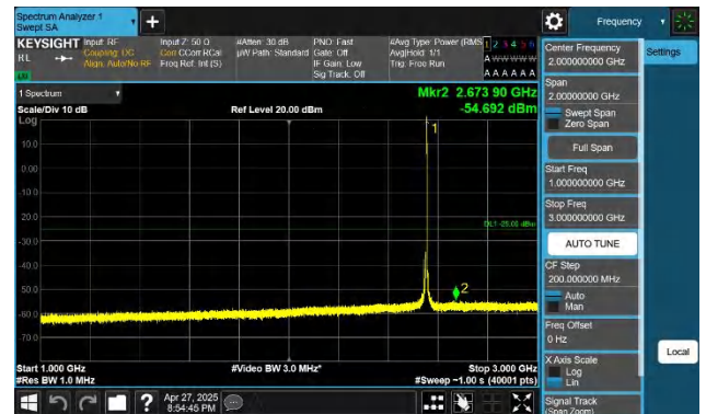
7-7-20MHz-15MHz-QPSK-QPSK-21201-21372-1RB#99-0RB#0-1000~3000MHz-PASS
