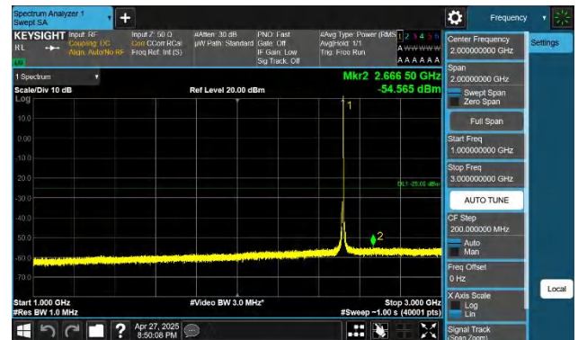
7-7-20MHz-15MHz-QPSK-QPSK-20850-21021-1RB#99-0RB#0-1 000~3000MHz-PASS
