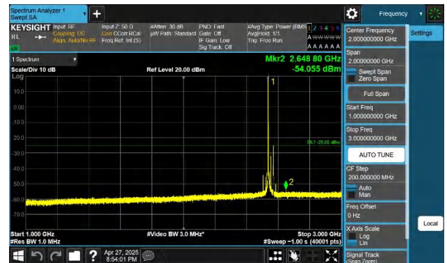
7-7-20MHz-15MHz-QPSK-QPSK-21201-21372-1RB#0-0RB#0-10 00~3000MHz-PASS
