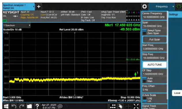
7-7-20MHz-15MHz-QPSK-QPSK-21026-21197-1RB#0-0RB#0-30 00~18000MHz-PASS
