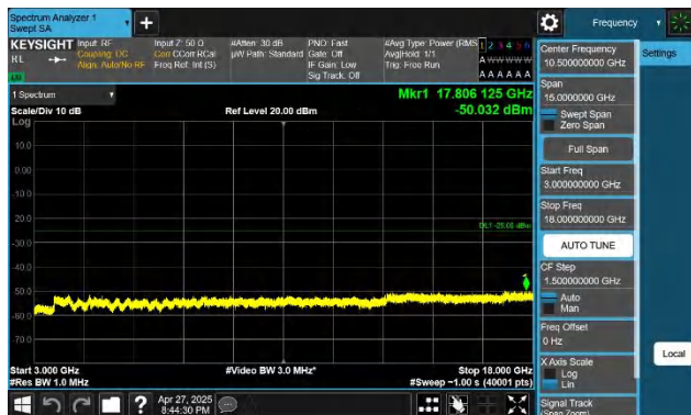
7-7-20MHz-10MHz-QPSK-QPSK-21051-21195-1RB#0-0RB#0-30 00~18000MHz-PASS
