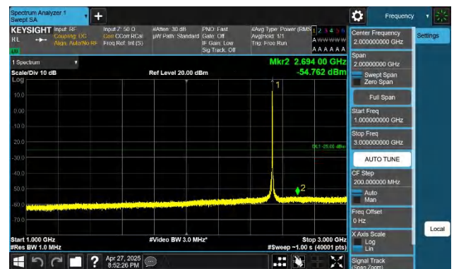
7-7-20MHz-15MHz-QPSK-QPSK-21026-21197-1RB#99-ORB#0-1 000~3000MHz-PASS
