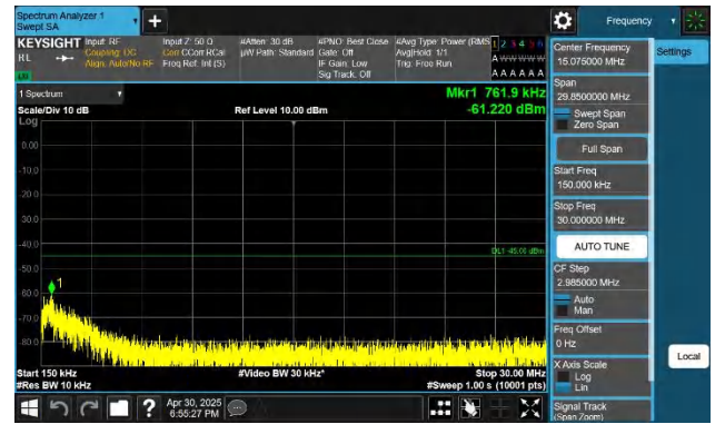
7-7-20MHz-10MHz-QPSK-QPSK-20850-20994-1RB#0-1RB#49-0. 15~30MHz-PASS
