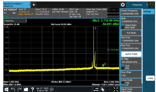
7-7-15MHz-20MHz-QPSK-QPSK-21179-21350-1RB#0-0RB#0-10 00~3000MHz-PASS
