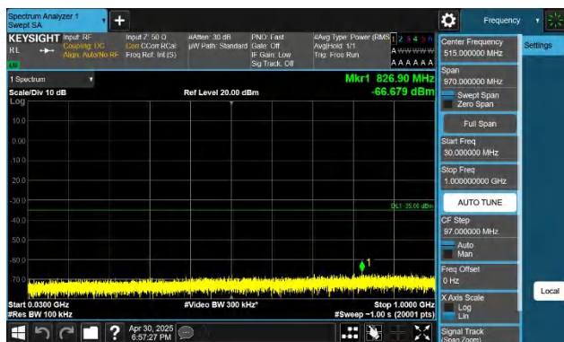
7-7-20MHz-10MHz-QPSK-QPSK-21251-21395-1RB#99-0RB#0- 30~1000MHz-PASS
