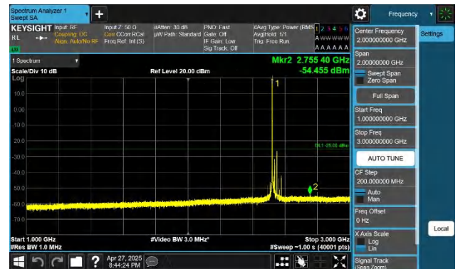
7-7-20MHz-10MHz-QPSK-QPSK-21051-21195-1RB#0-0RB#0-10 00~3000MHz-PASS
