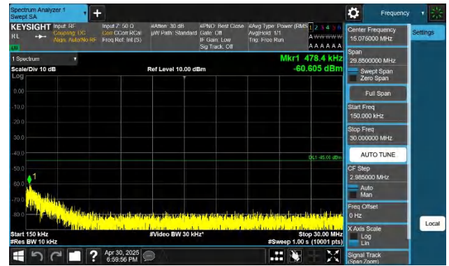
7-7-20MHz-15MHz-QPSK-QPSK-21026-21197-1RB#99-ORB#0-0. 15~30MHz-PASS
