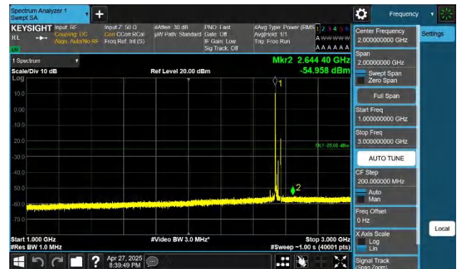
7-7-15MHz-20MHz-QPSK-QPSK-21179-21350-1RB#0-1RB#99-1 000~3000MHz-PASS
