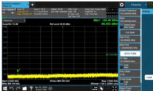
7-7-20MHz-10MHz-QPSK-QPSK-20850-20994-1RB#0-0RB#0-3 0~1000MHz-PASS
