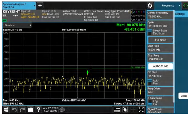
7-7-20MHz-10MHz-QPSK-QPSK-21251-21395-1RB#0-0RB#0-0. 009~0.15MHz-PASS
