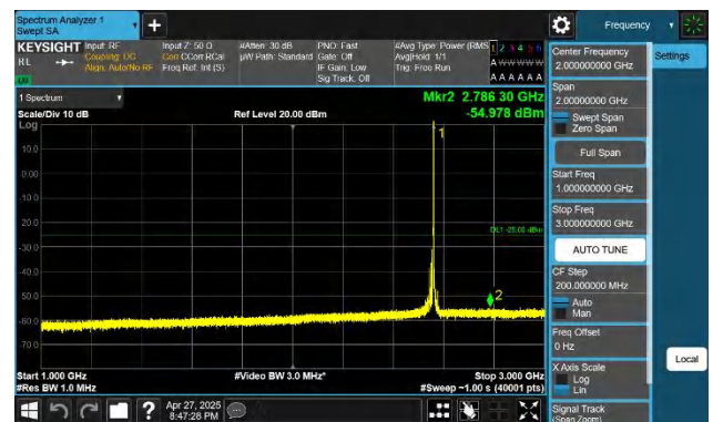
7-7-20MHz-10MHz-QPSK-QPSK-21251-21395-1RB#99-0RB#0-1 000~3000MHz-PASS
