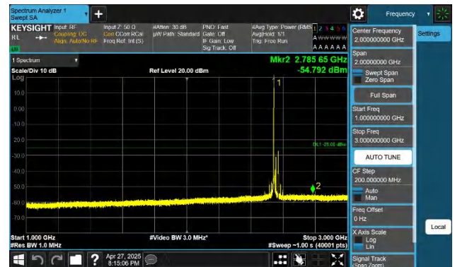
7-7-10MHz-20MHz-QPSK-QPSK-21206-21350-1RB#0-0RB#0-10 00~3000MHz-PASS
