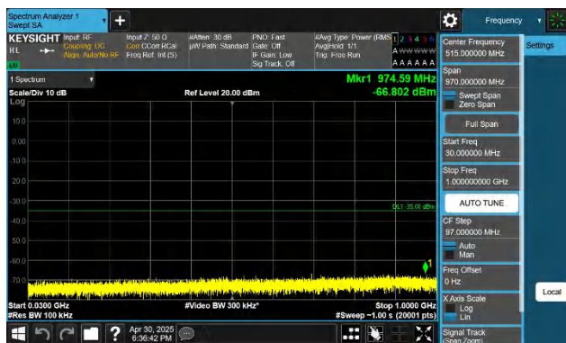
7-7-10MHz-20MHz-QPSK-QPSK-20805-20949-1RB#0-1RB#99- 30~1000MHz-PASS
