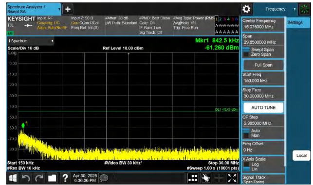
7-7-10MHz-20MHz-QPSK-QPSK-20805-20949-1RB#0-1RB#99-0. 15~30MHz-PASS
