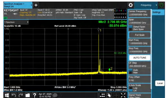
7-7-10MHz-20MHz-QPSK-QPSK-21006-21150-1RB#0-1RB#99-1 000~3000MHz-PASS
