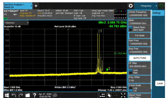
7-7-10MHz-20MHz-QPSK-QPSK-20805-20949-1RB#0-1RB#99-1 000~3000MHz-PASS
