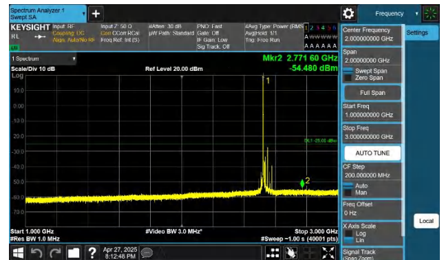
7-7-10MHz-20MHz-QPSK-QPSK-21006-21150-1RB#0-0RB#0-10 00~3000MHz-PASS
