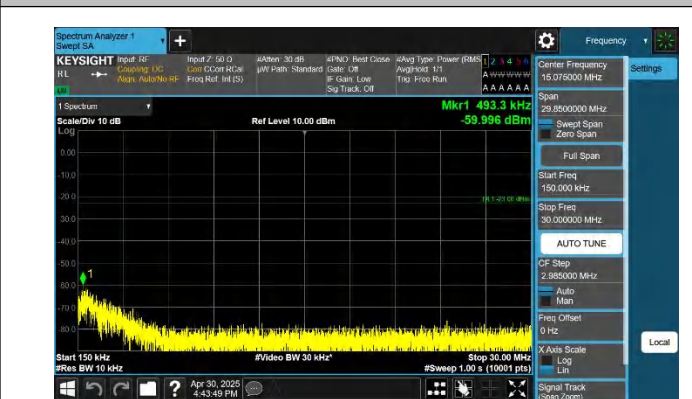
5-5-5MHz-10MHz-QPSK-QPSK-20478-20550-1RB#0-1RB#49-0. 15~30MHz-PASS
