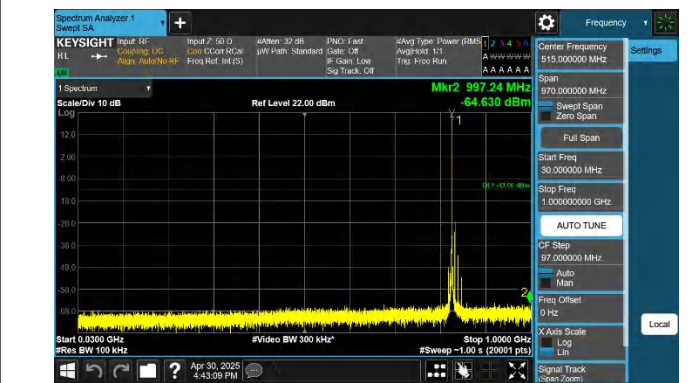
5-5-5MHz-10MHz-QPSK-QPSK-20478-20550-1RB#0-ORB#0-30~ 1000MHz-PASS
