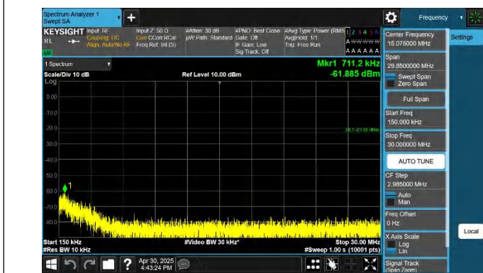
5-5-5MHz-10MHz-QPSK-QPSK-20478-20550-1RB#24-0RB#0-0. 15~30MHz-PASS
