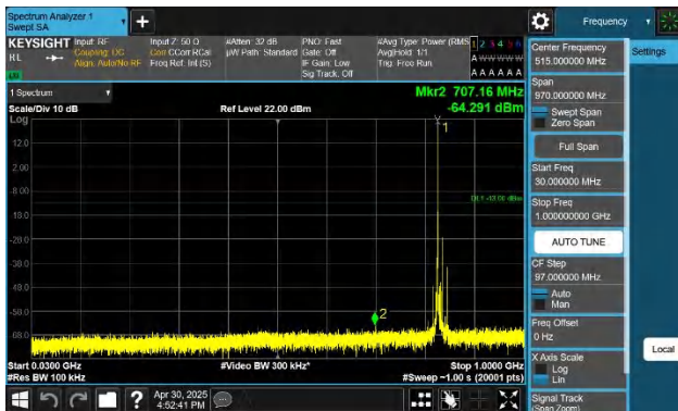
5-5-10MHz-10MHz-QPSK-QPSK-20501-20600-1RB#0-0RB#0-30 ~1000MHz-PASS
