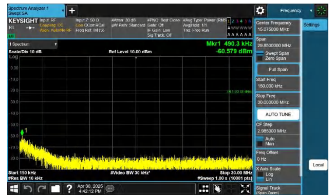
5-5-5MHz-10MHz-QPSK-QPSK-20428-20500-1RB#24-0RB#0-0. 15~30MHz-PASS
