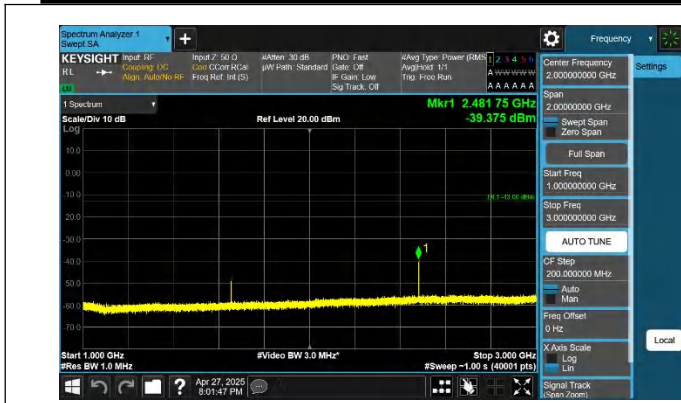
5-5-10MHz-10MHz-QPSK-QPSK-20476-20575-1RB#0-0RB#0-10 00~3000MHz-PASS
