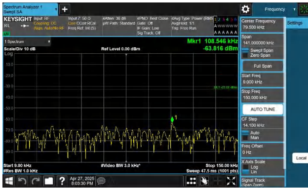
5-5-10MHz-10MHz-QPSK-QPSK-20501-20600-1RB#0-0RB#0-0. 009~0.15MHz-PASS
