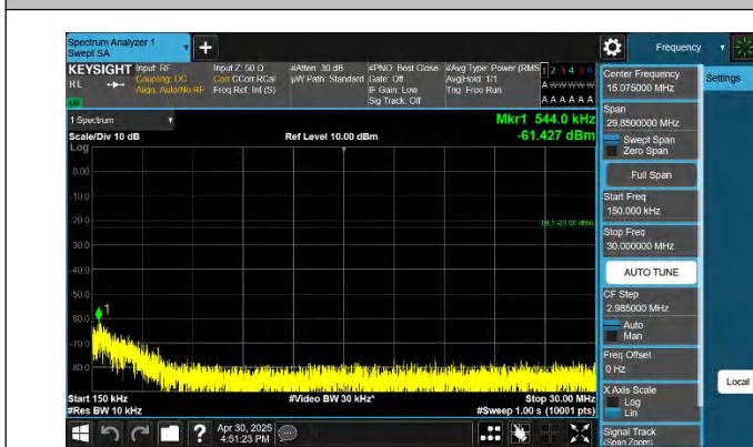
5-5-10MHz-10MHz-QPSK-QPSK-20476-20575-1RB#0-0RB#0-0. 15~30MHz-PASS
