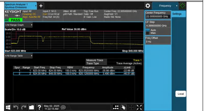
5-5-5MHz-10MHz-QPSK@QPSK-QPSK-20428-20500-25 RB#0@25RB#0-50RB#0@50RB#0-PASS
