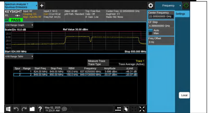
5-5-5MHz-10MHz-QPSK@QPSK-QPSK@QPSK-20528-20600-25 RB#0@25RB#0-50RB#0@50RB#0-PASS
