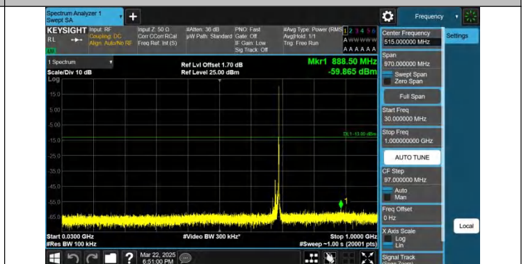
Band71-20MHz-QPSK-133372-1RB#99-30~1000-PASS
