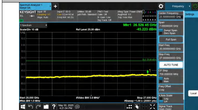
Band41-20MHz-QPSK-41490-1RB#0-20000~27000-PASS
