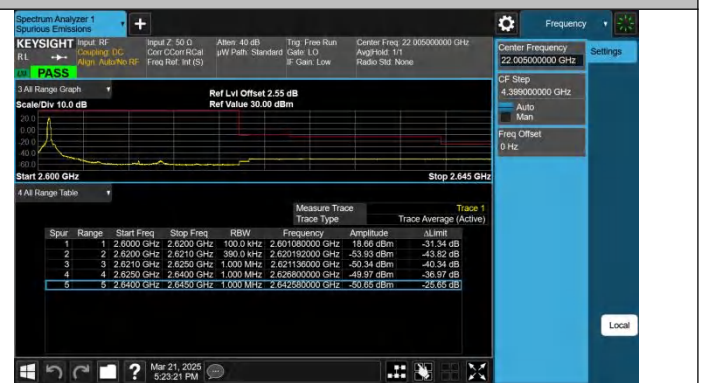
Band38-20MHz-QPSK-38150-1RB#0-PASS
