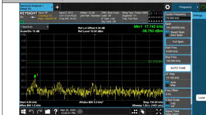
Band26(824-849)-3MHz-QPSK-27025-1RB#0-0.009~0.15-PASS
