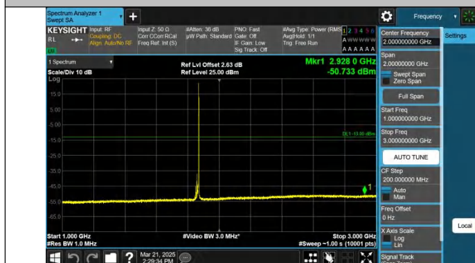
Band25-20MHz-QPSK-26140-1RB#99-1000~3000-PASS
