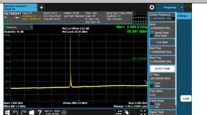
Band25-20MHz-QPSK-26365-1RB#0-1000~3000-PASS
