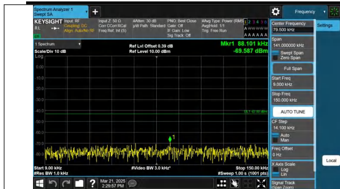
Band25-20MHz-QPSK-26365-1RB#0-0.009~0.15-PASS
