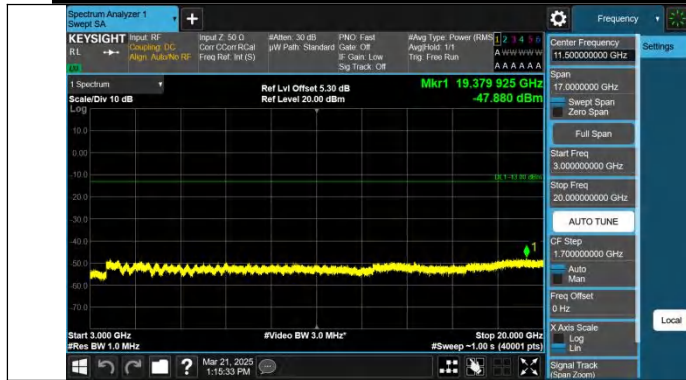
Band25-10MHz-QPSK-26365-1RB#0-3000-PASS
