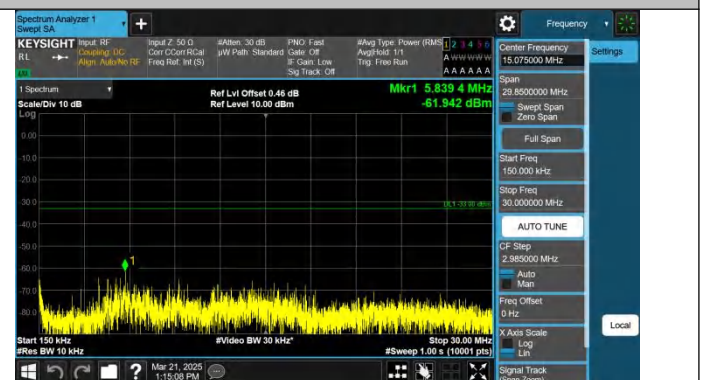
Band25-10MHz-QPSK-26365-1RB#0-0.15~30-PASS
