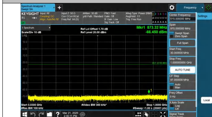
Band25-20MHz-QPSK-26365-1RB#0-30~1000-PASS
