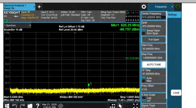
Band25-20MHz-QPSK-26365-1RB#99-30~1000-PASS
