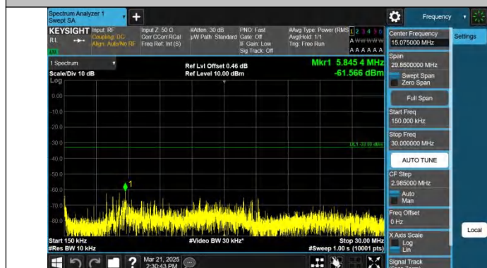
Band25-20MHz-QPSK-26365-1RB#99-0.15~30-PASS
