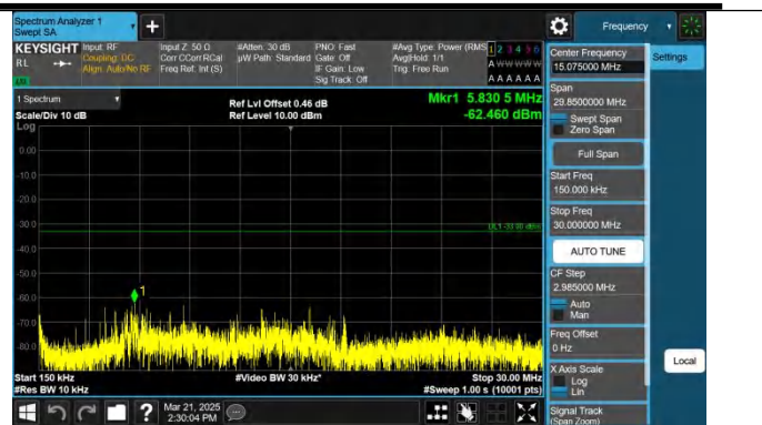
Band25-20MHz-QPSK-26365-1RB#0-0.15~30-PASS
