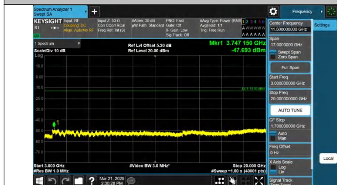
Band25-20MHz-QPSK-26365-1RB#0-3000~20000-PASS
