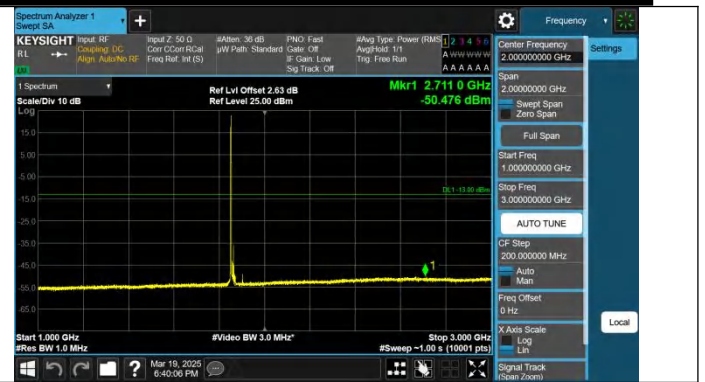
Band2-20MHz-QPSK-18700-1RB#0-1000~3000-PASS
