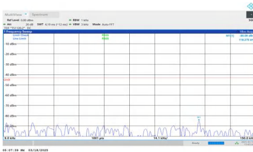
NTNV-DC_7A-n25A-PC3-15-5+10-M+M-QPSK-IDLE-DFT-QPSK-I nner_1RB_Left-0.009-0.15-PASS
