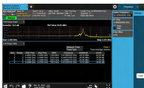
NTNV-n78(3450-3550)-PC2-30-20-L-CP-QPSK-Edge_1RB_Left-P ASS
