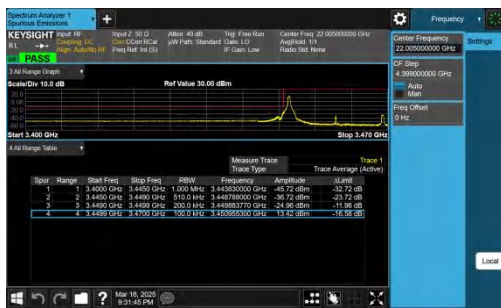
NTNV-n78(3450-3550)-PC2-30-20-L-CP-QPSK-Edge_1RB_Left-P ASS
