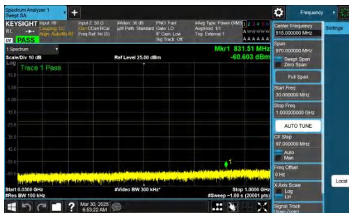
NTNV-n77(3700-3980)-PC2-30-80-M-CP-QPSK-Inner_1RB_Left-30-1000-PASS
