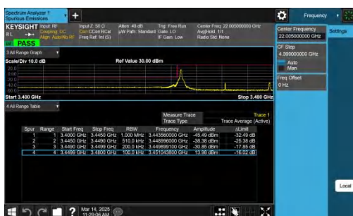
NTNV-n77(3450-3550)-PC2-30-30-L-CP-QPSK-Edge_1RB_Left-P ASS
