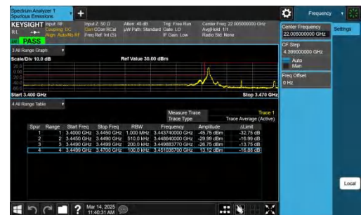
NTNV-n77(3450-3550)-PC2-30-20-L-CP-QPSK-Edge_1RB_Left-PA SS
