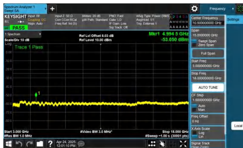
NTNV-n41-PC2-30-30-L-CP-QPSK-Inner_1RB_Left-3000-18000-
