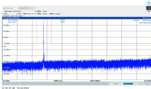
NTNV-n77(3700-3980)-PC2-30-30-M-DFT-QPSK-Inner_1RB_Lef t-3000-6000-PASS
