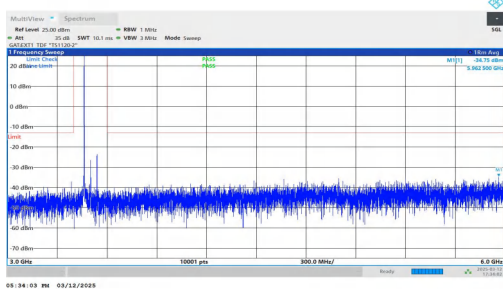
NTNV-n77(3450-3550)-PC2-30-80-M-DFT-QPSK-Inner_1RB_Lef t-3000-6000-PASS
