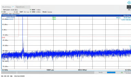
NTNV-n77(3450-3550)-PC2-30-30-M-DFT-QPSK-Inner_1RB_Lef t-3000-6000-PASS
