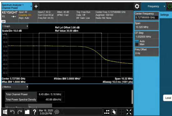
11AX40MIMO-Ant1-5755-PASS
