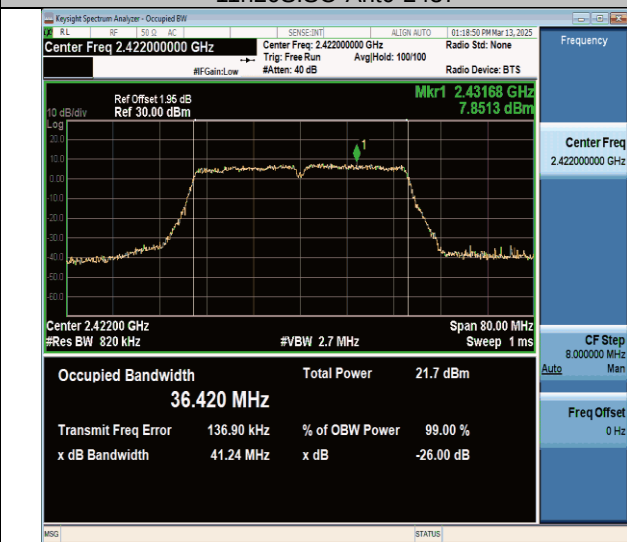
11n40SISO-Ant0-2422
