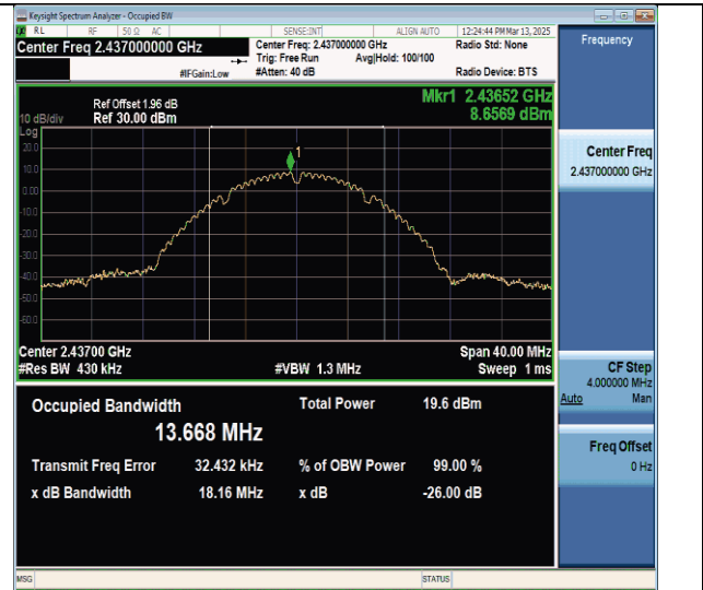
11b-Ant0-2437
