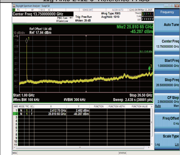
11g-Ant0-2412-1000~26500-PASS
