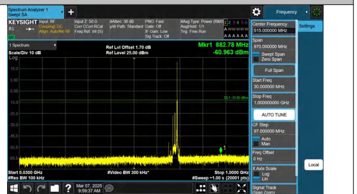
Band71-20MHz-QPSK-133372-1RB#99-30~1000-PASS
