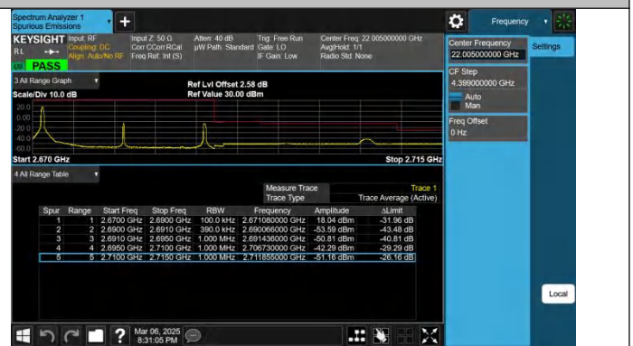
Band41-20MHz-QPSK-41490-1RB#0-PASS
