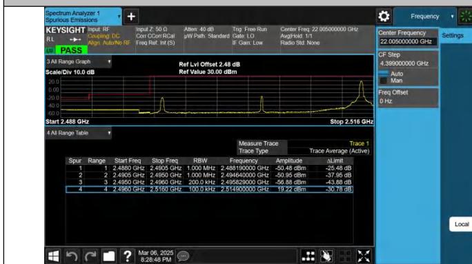
Band41-20MHz-QPSK-39750-1RB#99-PASS
