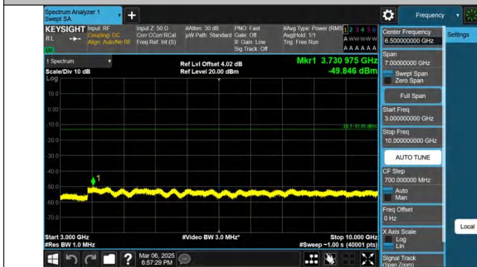
Band26(824-849)-10MHz-QPSK-26990-1RB#0-3000~10000-PAS
