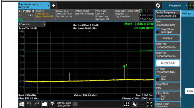
Band26(824-849)-3MHz-QPSK-27025-1RB#14-1000~3000-PASS
