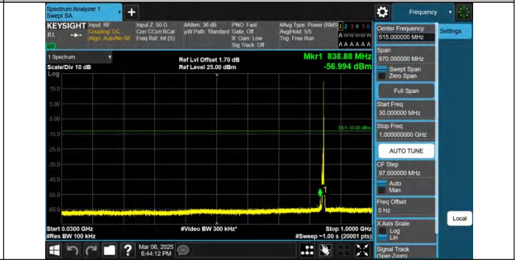
Band26(824-849)-3MHz-QPSK-27025-1RB#14-30~1000-PASS
