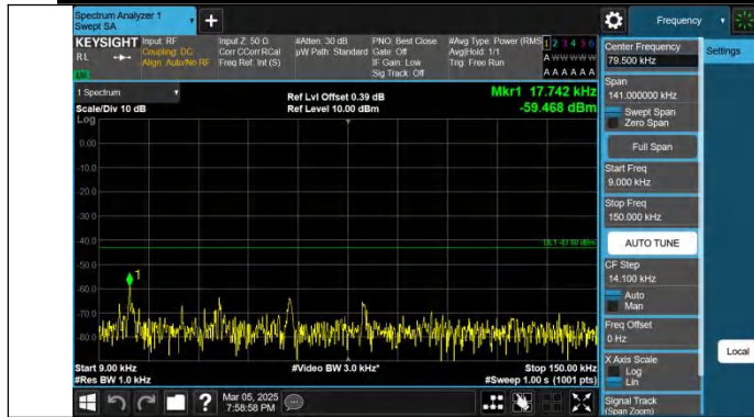
Band4-20MHz-QPSK-20175-1RB#0-0.009~0.15-PASS
